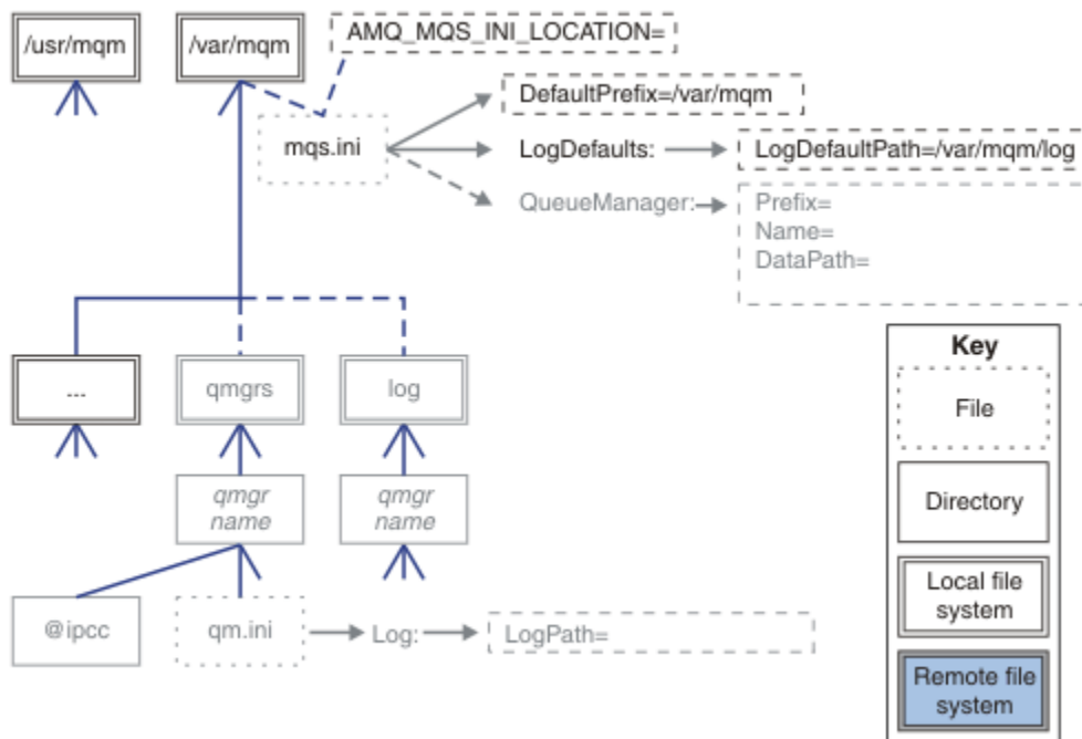
Figura 36. Modello di modello struttura di directory
