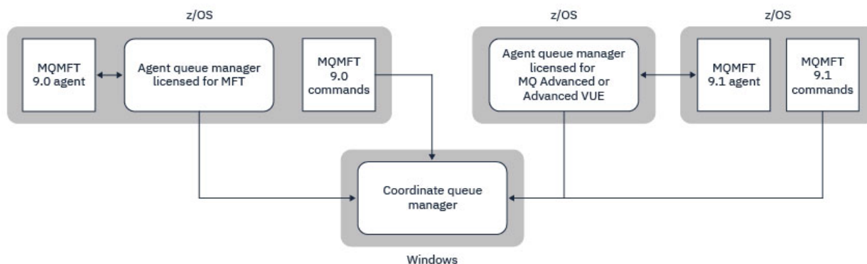
Figura 48. Alcuni comandi, come fteListAgents , si connettono direttamente al gestore code di coordinamento per una topologia MFT.
