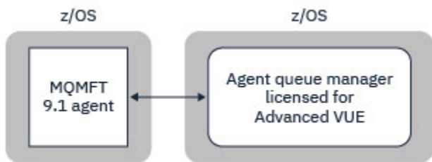
Figura 44. Gli agent di MFT 9.1 su z/OS possono connettersi ad un gestore code utilizzando il trasporto CLIENT, supponendo che il gestore code sia concesso in licenza per Advanced VUE.
