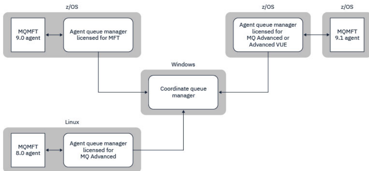
Figura 47. Gli agent MFT in esecuzione su z/OS possono far parte di una topologia MFT in cui il gestore code di coordinamento è in esecuzione su una piattaforma multipla IBM MQ.
