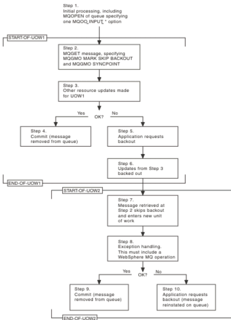
Figura 67. Il backout viene ignorato utilizzando MQGMO_MARK_SKIP_BACKOUT
