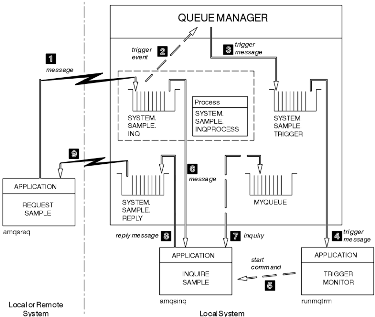
Figura 136. Richiedi e richiedi esempi utilizzando il trigger
