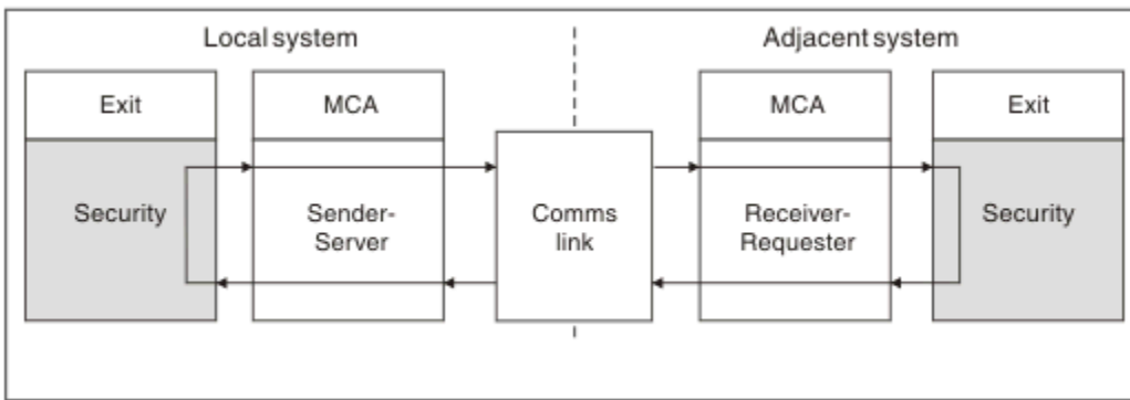
Figura 107. Loop uscita di sicurezza
