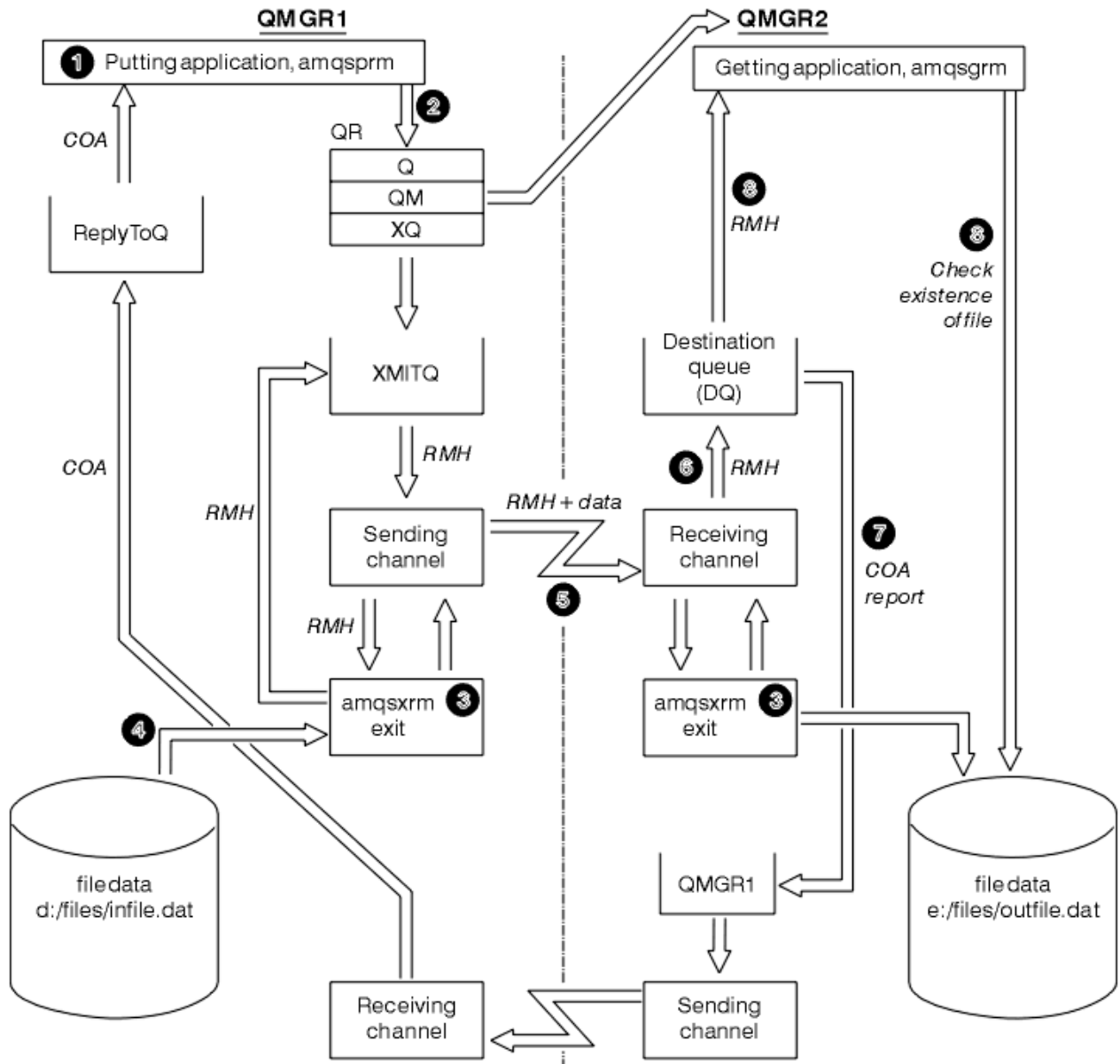
Figura 135. Esecuzione degli esempi del messaggio di riferimento
