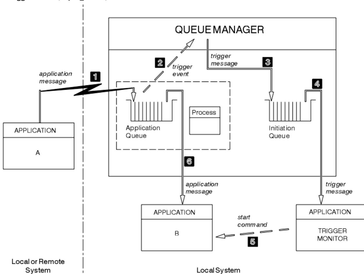
Figura 99. Flusso di messaggi di applicazione e trigger
