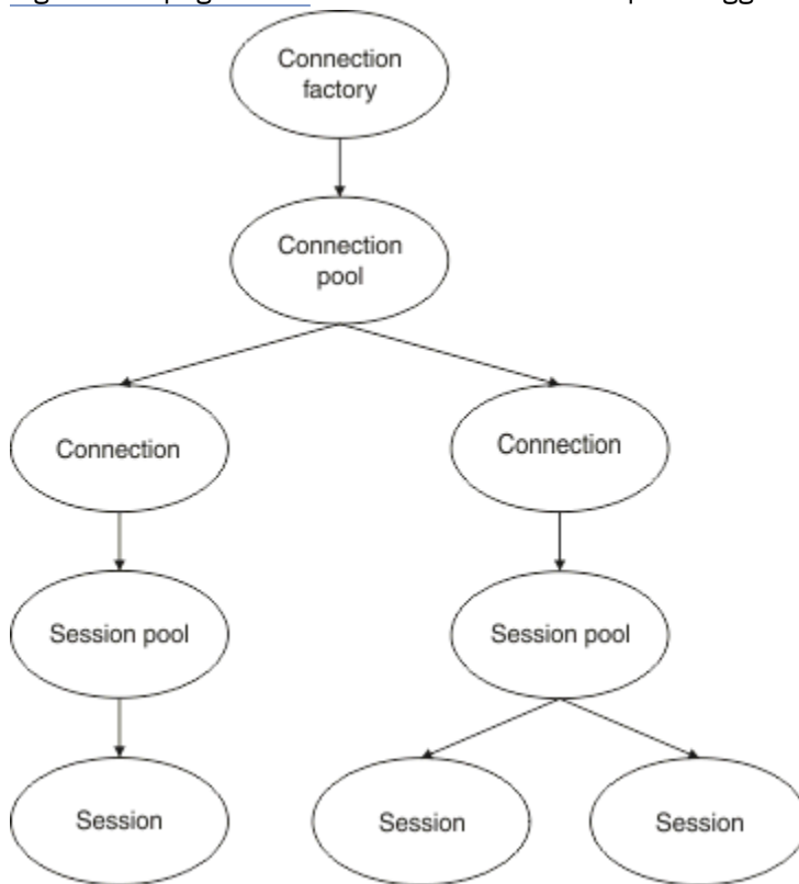
Figura 48. Pool di connessioni e pool di sessione
