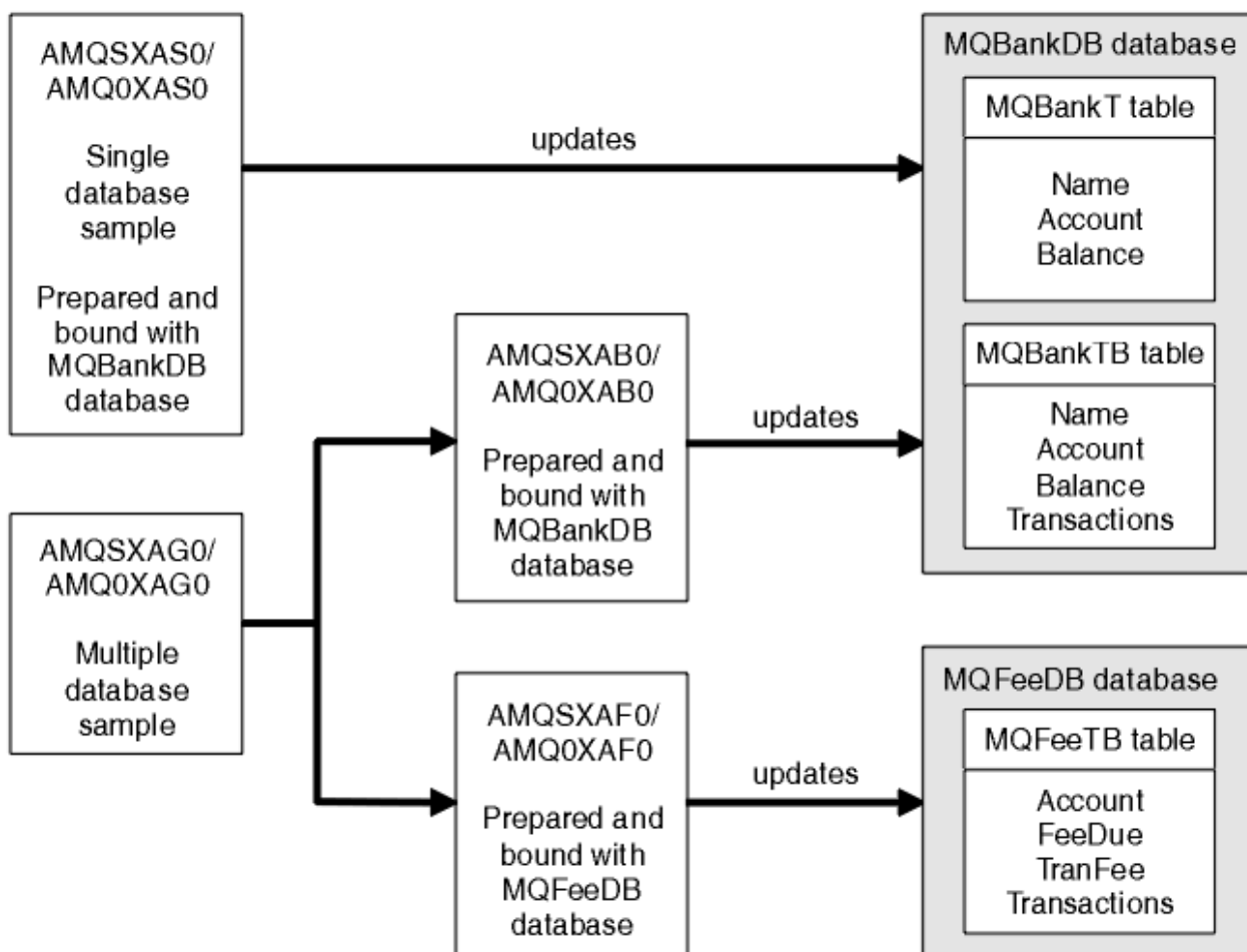
Figura 132. Gli esempi di coordinamento del database
