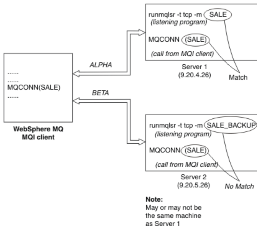
Figura 102. Esempio MQCONN
