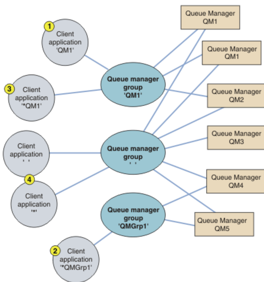
Figura 101. Gruppi gestore code
