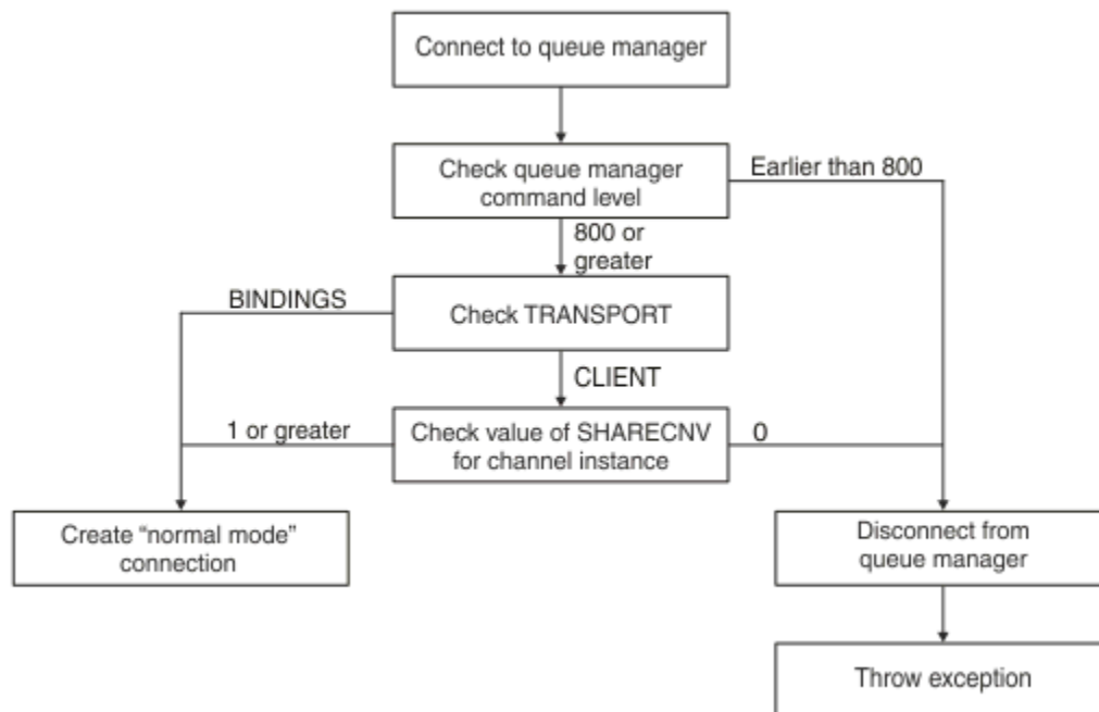
Figura 93. Modalità normale PROVIDERVERSION
