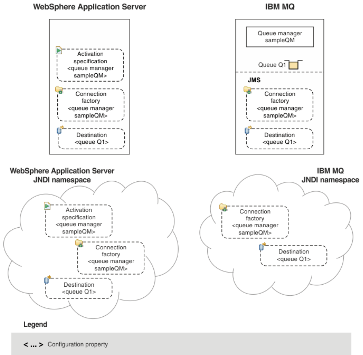
Figura 91. Oggetti creati in WebSphere Application Server e oggetti corrispondenti in IBM MQ
