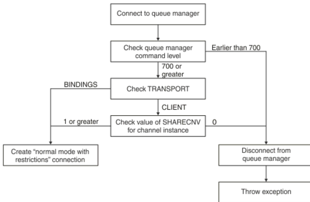
Figura 94. Modalità normale PROVIDERVERSION con restrizioni
