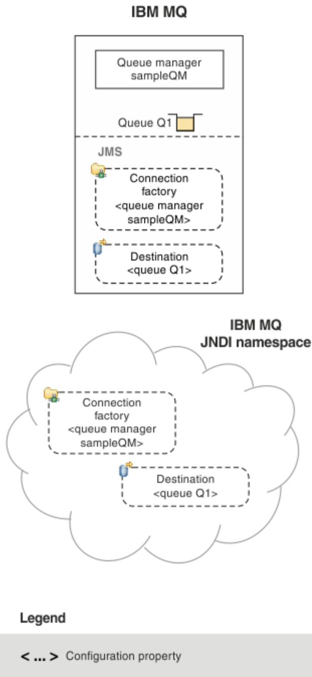
Figura 90. JMS oggetti creati in IBM MQ
