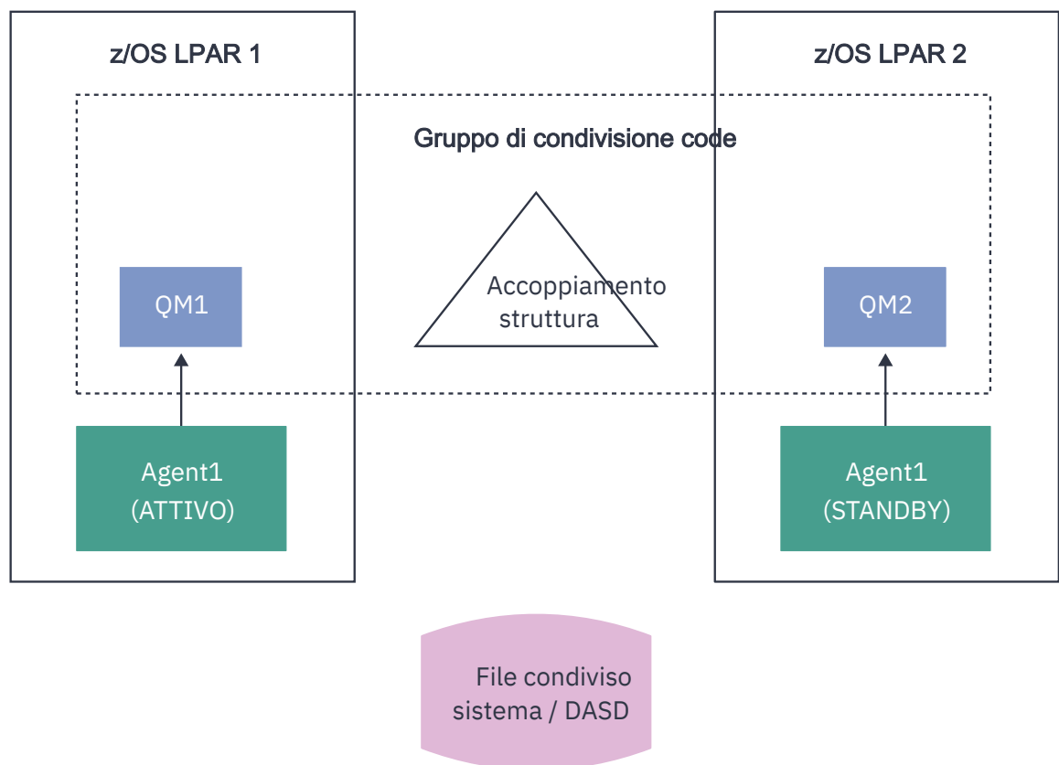
Figura 98. Agent MFT ad alta disponibilità che utilizza un gruppo di condivisione code
