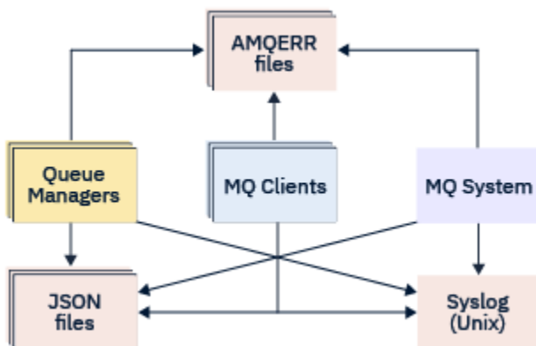
Figura 5. Come le diverse parti di IBM MQ possono riportare i messaggi diagnostici
