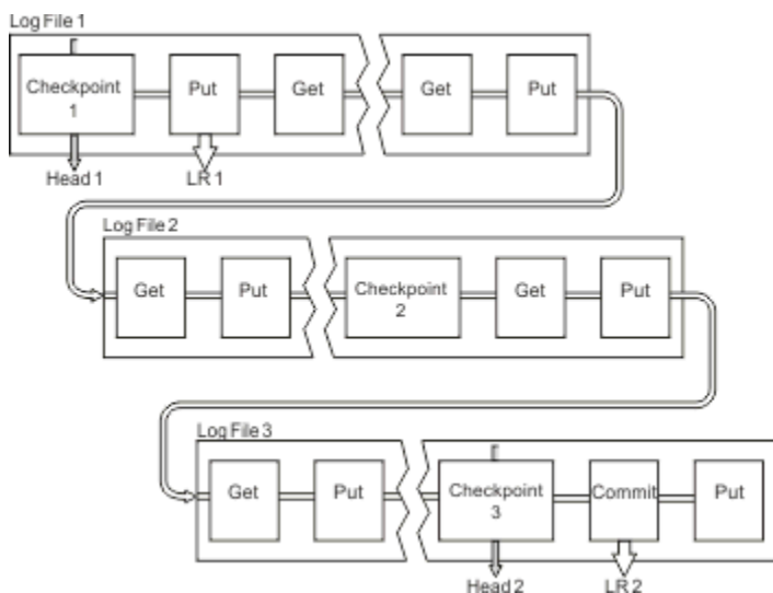
Figura 88. Checkpoint con una transazione di lunga durata
