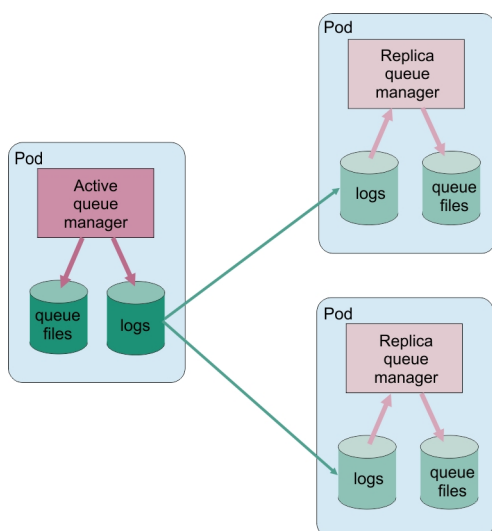
Figura 86. Esempio di configurazione della HA nativa
