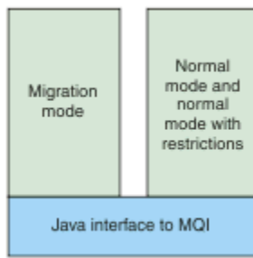
Figura 92. Modalità del provider di messaggistica
