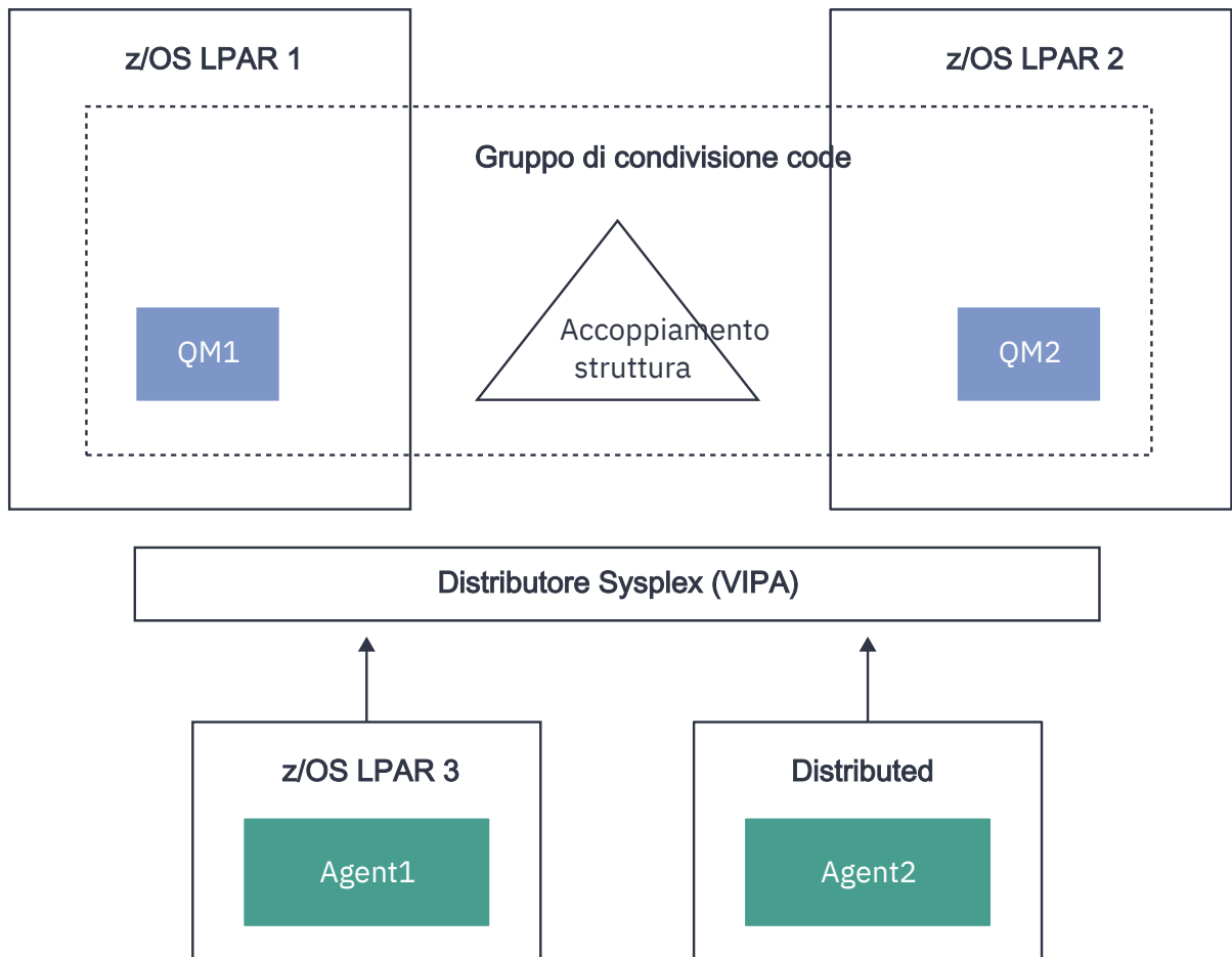
Figura 99. Agent MFT che si connettono a un gruppo di condivisione code come client
