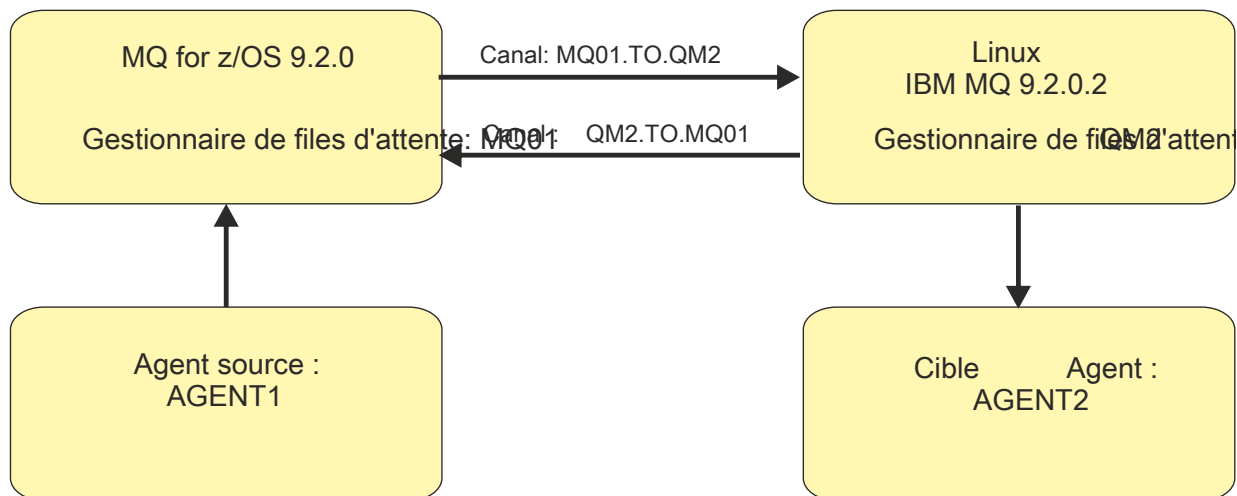
Figure 56. Exemple de diagramme simple montrant comment un agent source, AGENT1, et un agent de destination, AGENT2, et leurs gestionnaires de files d'attente d'agent, MQ01 et QM2, sont connectés.
