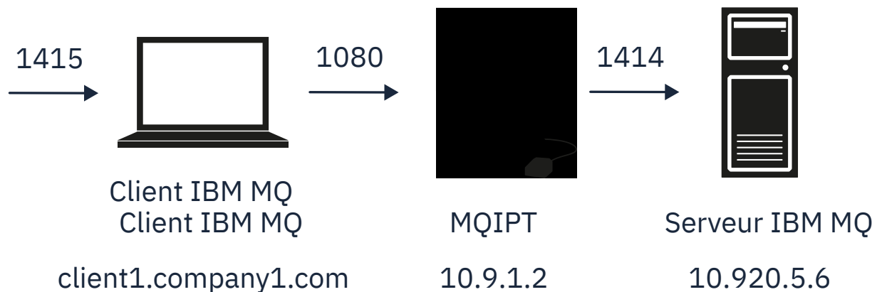
Figure 35. Diagramme réseau du proxy SOCKS
