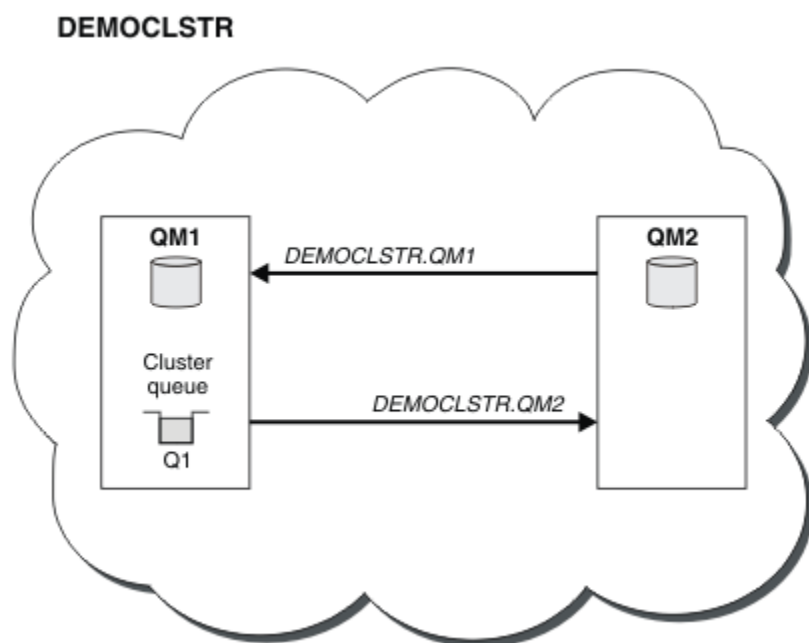
Figure 8. Un petit cluster de deux gestionnaires de files d'attente
