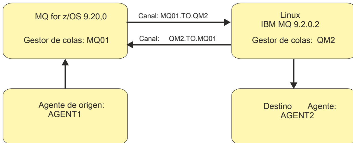
Figura 56. Ejemplo de un diagrama simple que muestra cómo se conectan un agente de origen, AGENT1, y un agente de destino, AGENT2, y sus gestores de colas de agente, MQ01 y QM2 .
