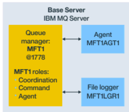
Figura 25. Topología básica con un gestor de colas
