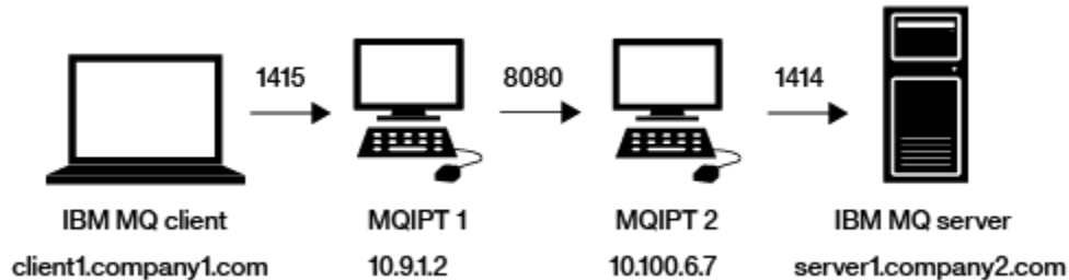
Figura 33. Diagrama de red de túneles HTTP
