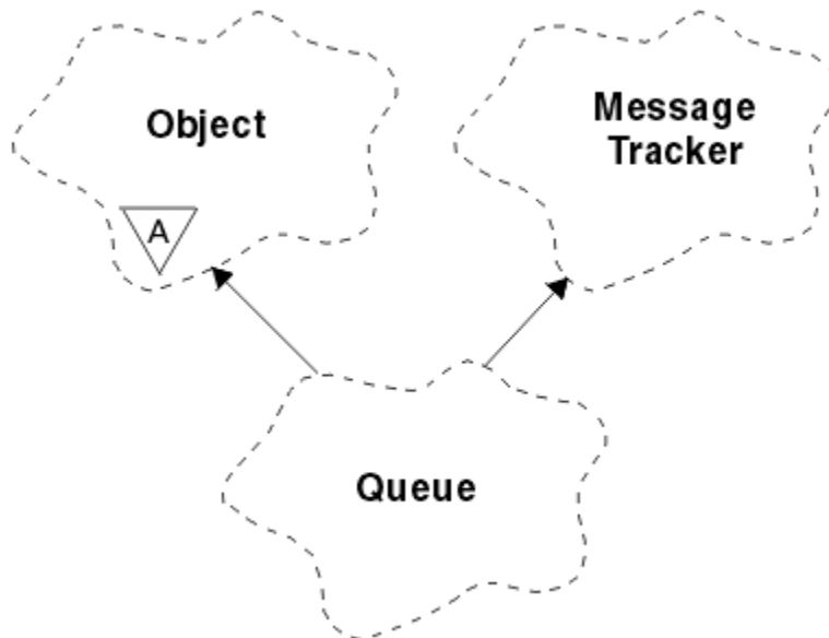
Figura 32. Clase ImqQueue
