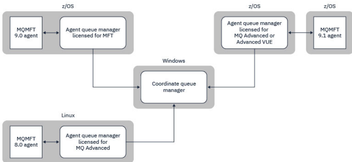
Figura 47. Los agentes de MFT que se ejecutan en z/OS pueden formar parte de una topología de MFT donde el gestor de colas de coordinación se ejecuta en una multiplataforma IBM MQ.
