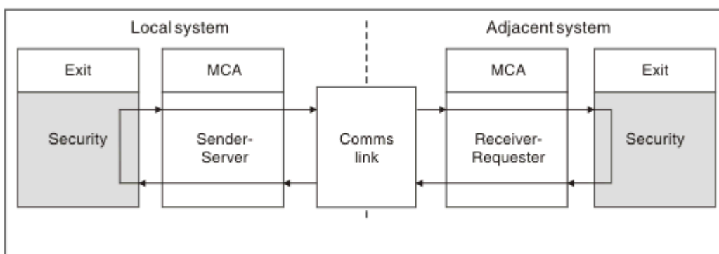
Figura 107. Bucle de salida de seguridad
