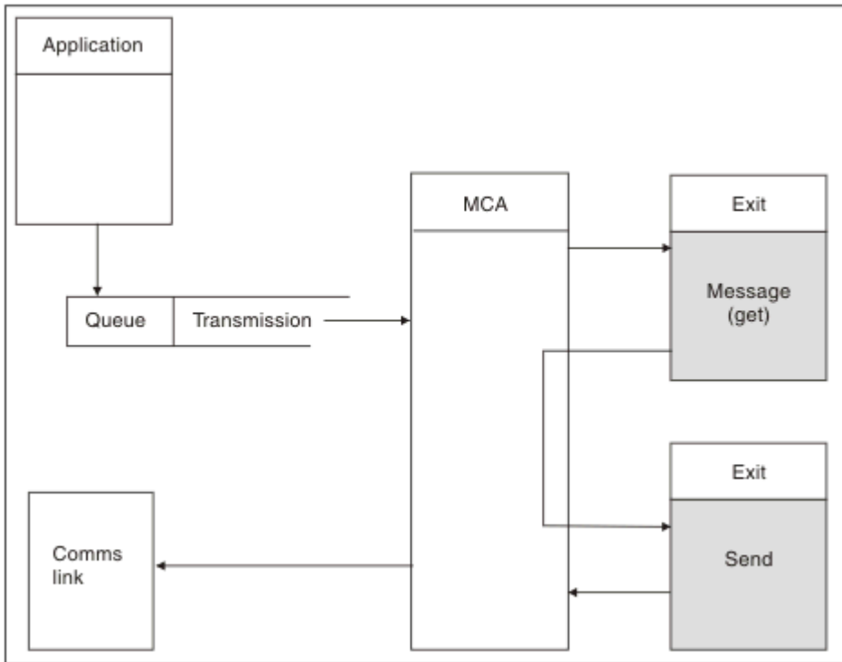
Figura 108. Ejemplo de una salida de envío en el extremo emisor del canal de mensajes
