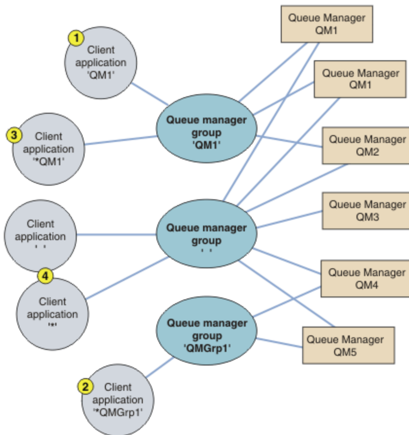
Figura 101. Grupos de gestores de colas
