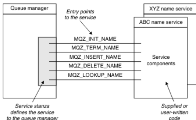
Figura 103. Servicios, componentes y puntos de entrada
