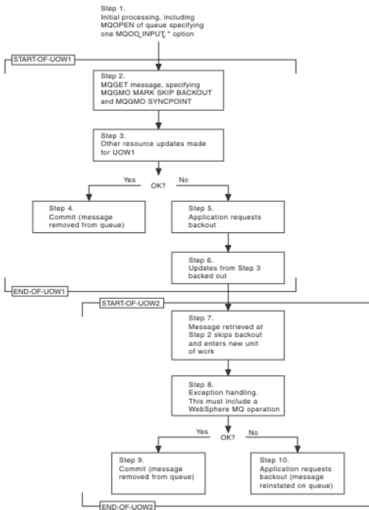
Figura 67. Omisión de restitución utilizando MQGMO_MARK_SKIP_BACKOUT
