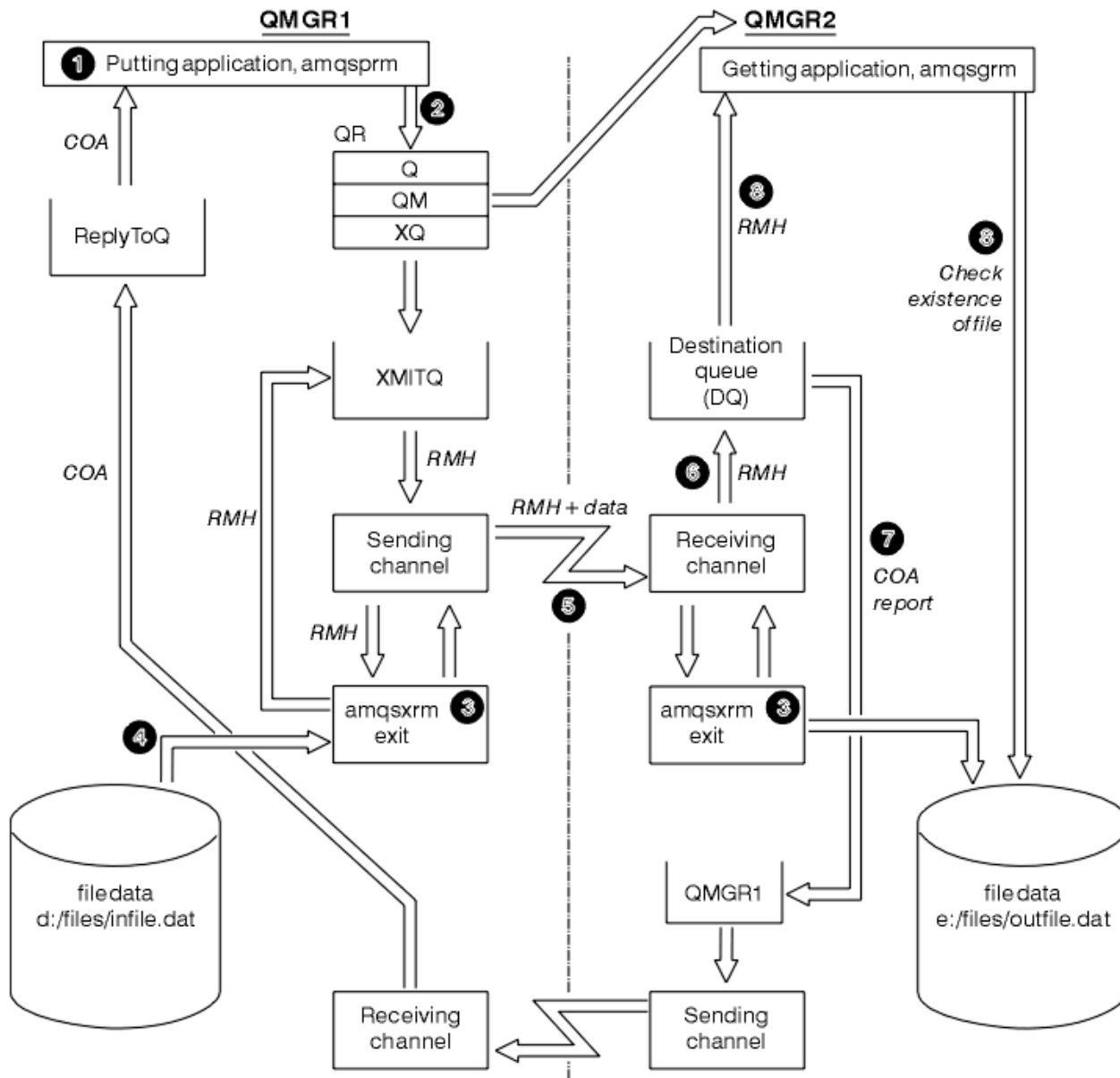
Figura 135. Ejecución de los ejemplos de mensajes de referencia
