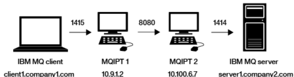
Abbildung 33. HTTP-Tunneling-Netzdiagramm
