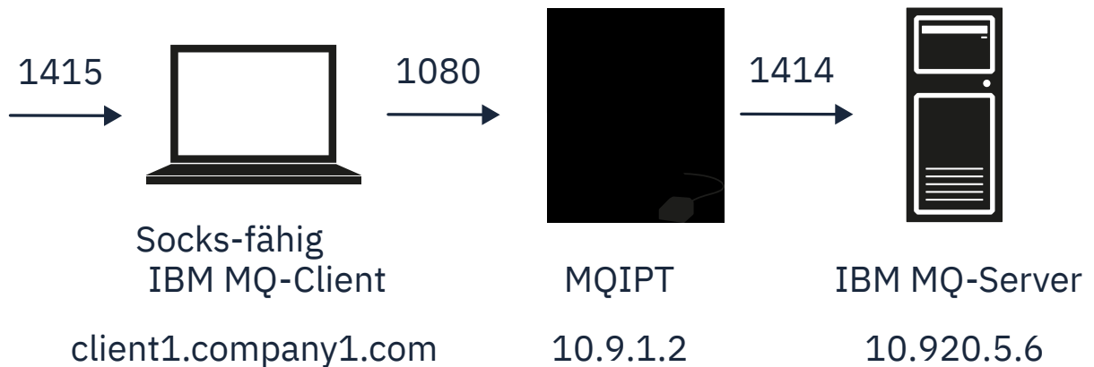
Abbildung 35. SOCKS-Proxy-Netzdiagramm
