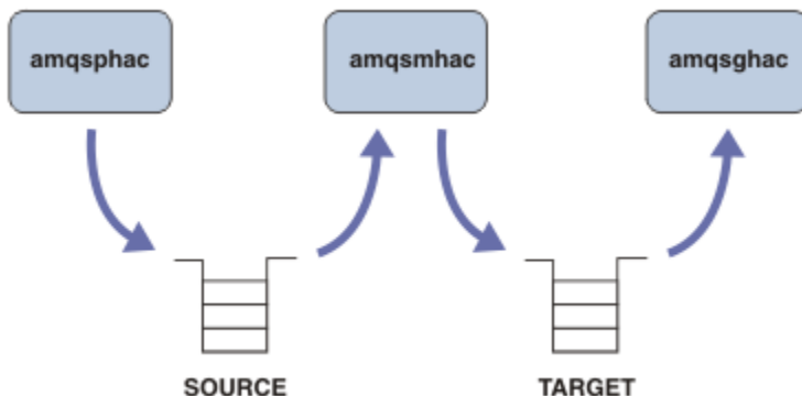
圖 134: 可重新連接的用戶端範例
