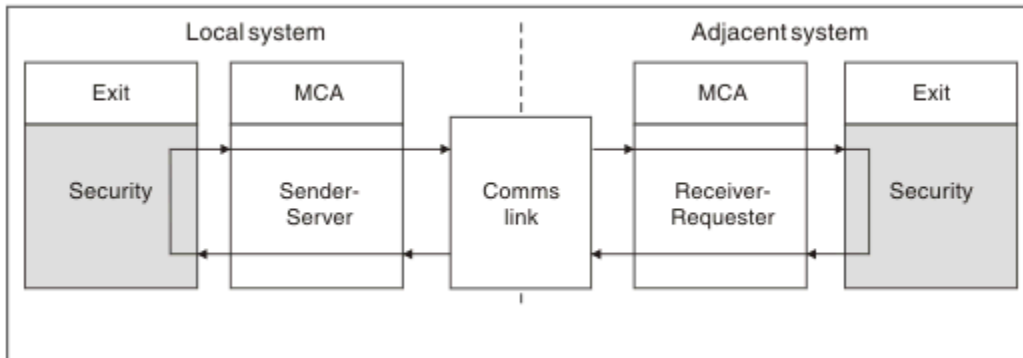
圖 108: 安全結束程式迴圈
