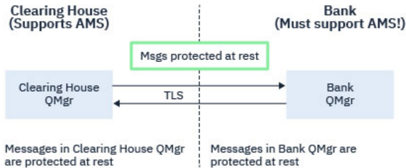
图 32: AMS 的当前使用情况
