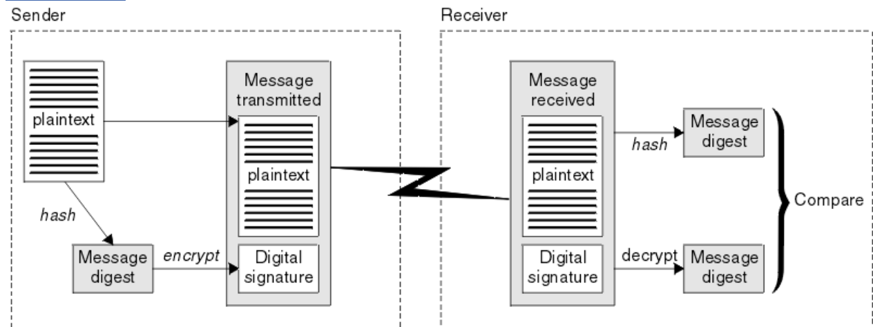
图 6: 数字签名过程
