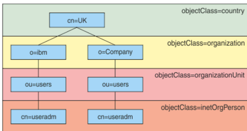
图 8: 示例 LDAP 层次结构
