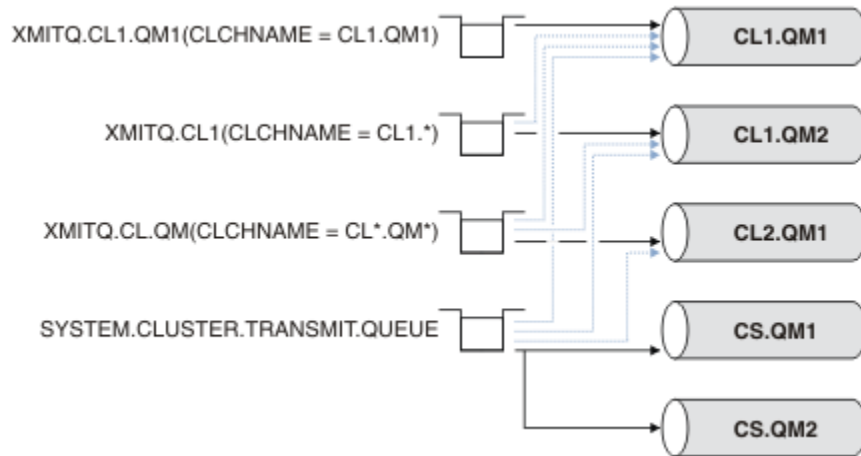
图 40: 多个集群发送方通道
