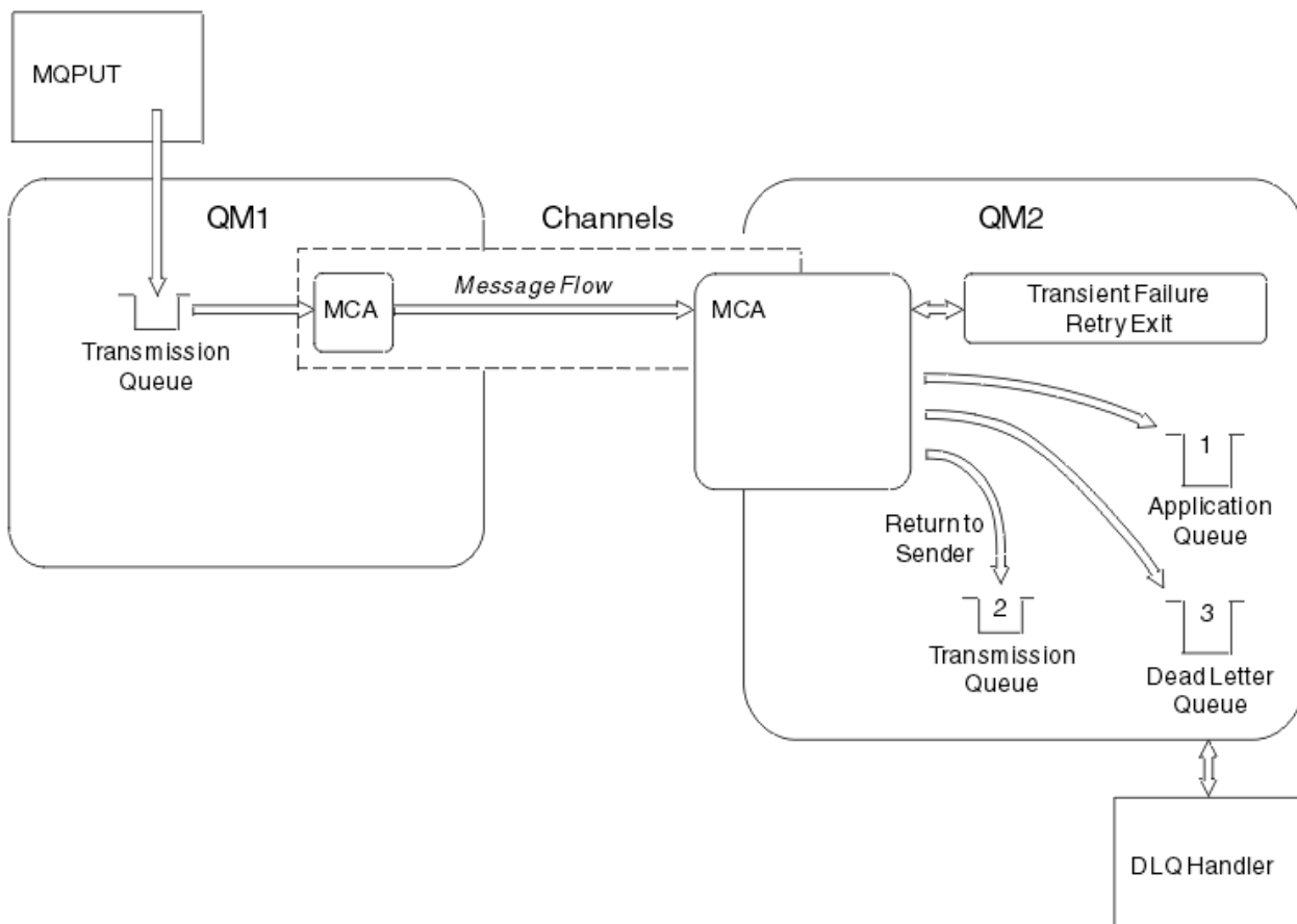
图 25: 无法传递消息时发生的情况
