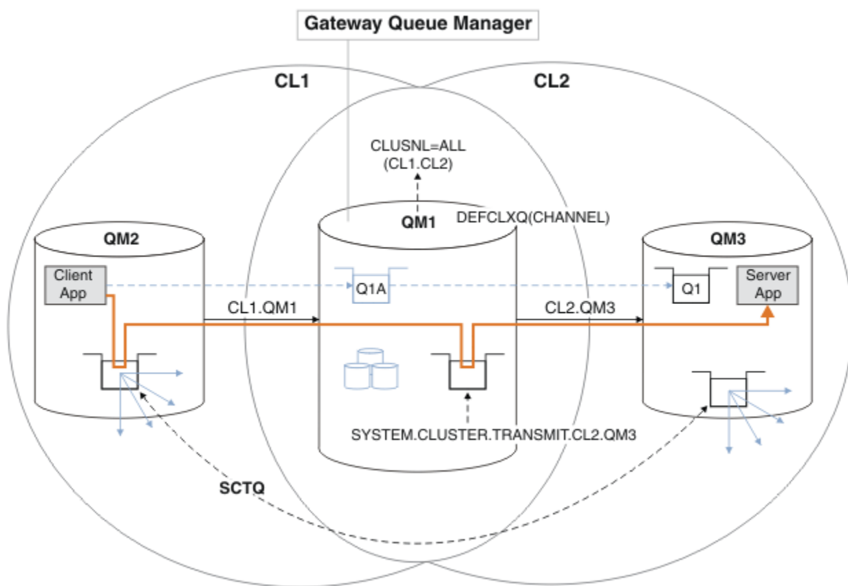
图 54: 客户机/服务器应用程序已部署到具有网关队列管理器上的独立集群传输队列的中心和辐射体系结构。
