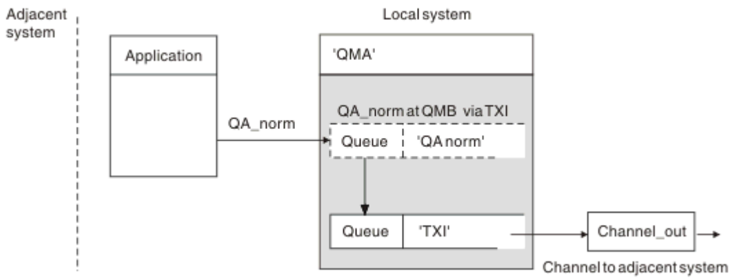
图 9: 远程队列定义允许使用其他传输队列
