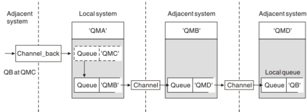
图 14: 将消息流转移到另一个目标
