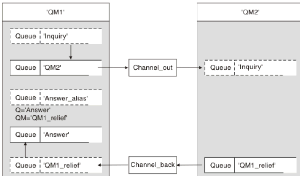
图 16: 应答队列别名示例
