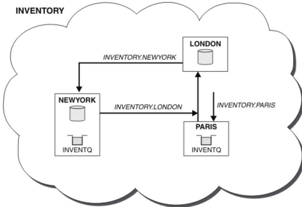
图 62: 具有三个队列管理器的 INVENTORY 集群
