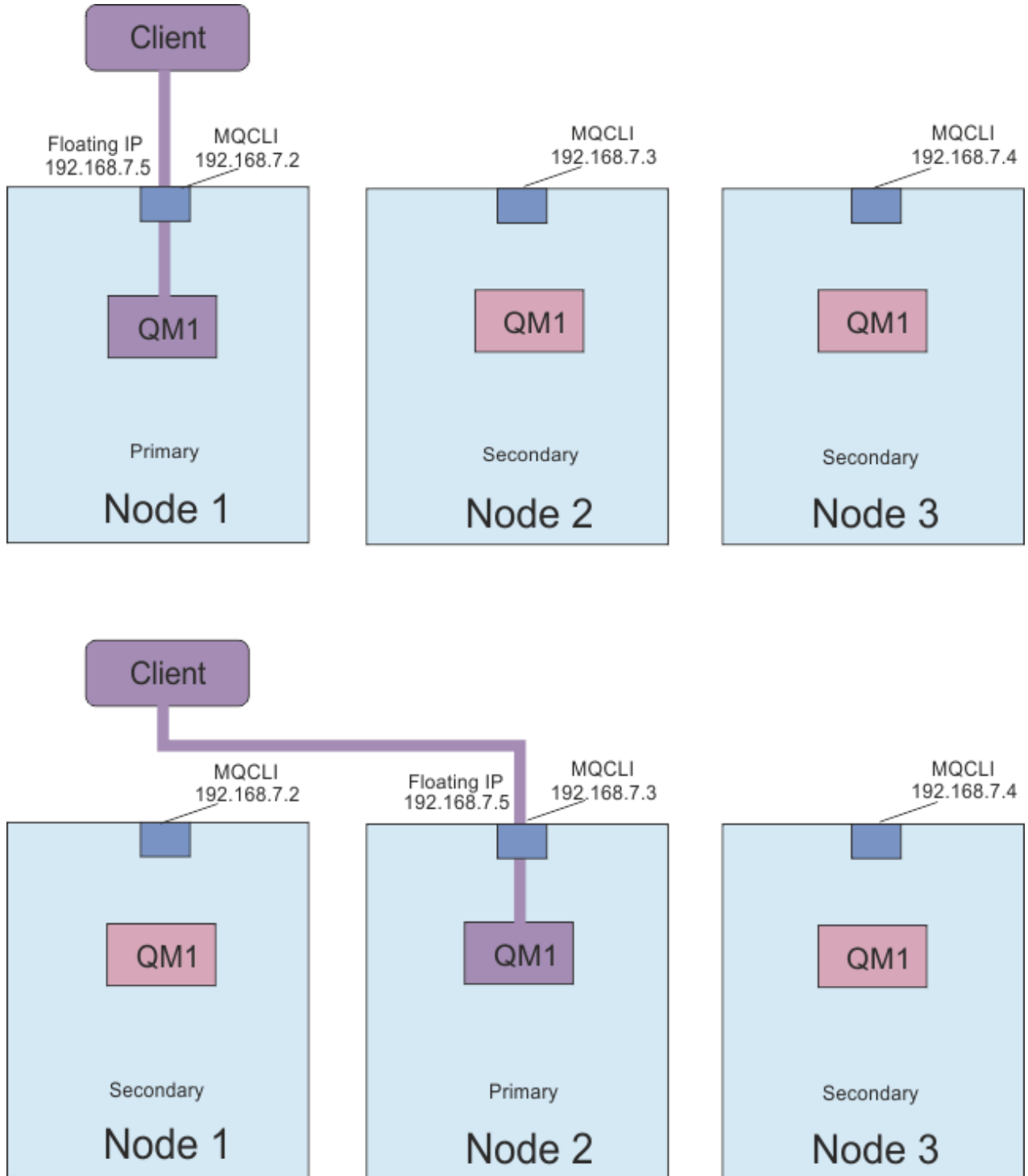
图 83: 浮动 IP 地址
