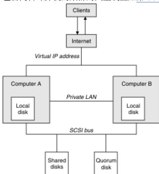
图 74: 双计算机 MSCS 集群
