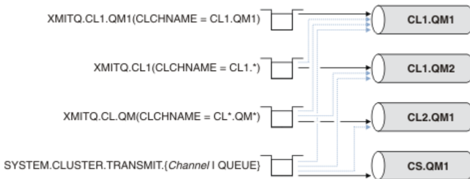
图 39: 传输队列/集群发送方通道优先顺序
