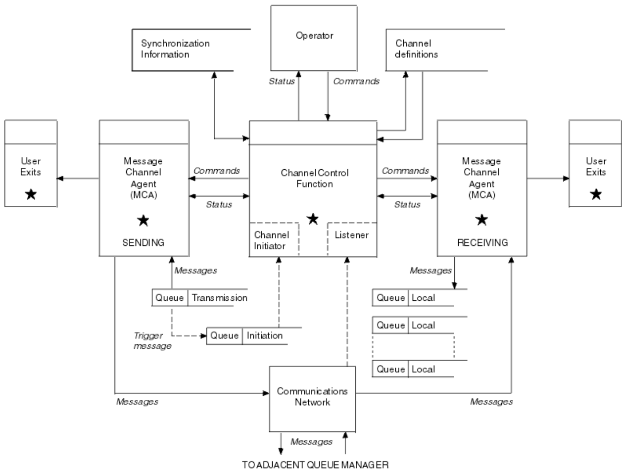
图 17: 分布式队列管理模型
