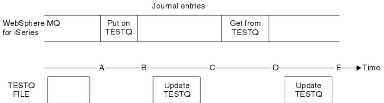
图 28: 更新 MQM 对象时的事件序列
