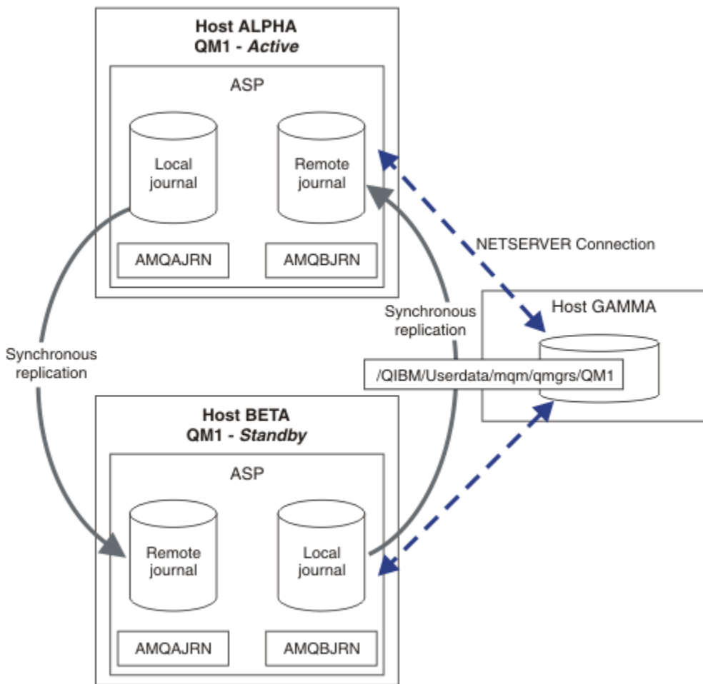
图 32: 镜像日志配置
