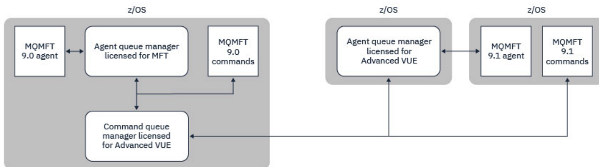
Figura 46. Comandos conectam-se ao gerenciador de filas de comandos para uma topologia MFT. Ao executar esses comandos no z/OS, o gerenciador de filas de comandos também deve estar em z/OS
