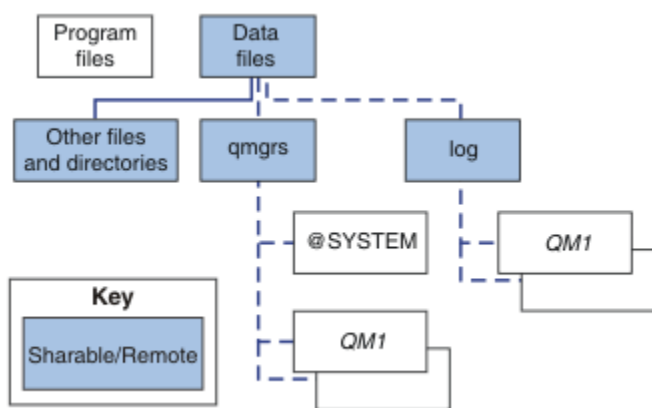
Figura 32. Visão geral da estrutura de diretório do IBM MQ
