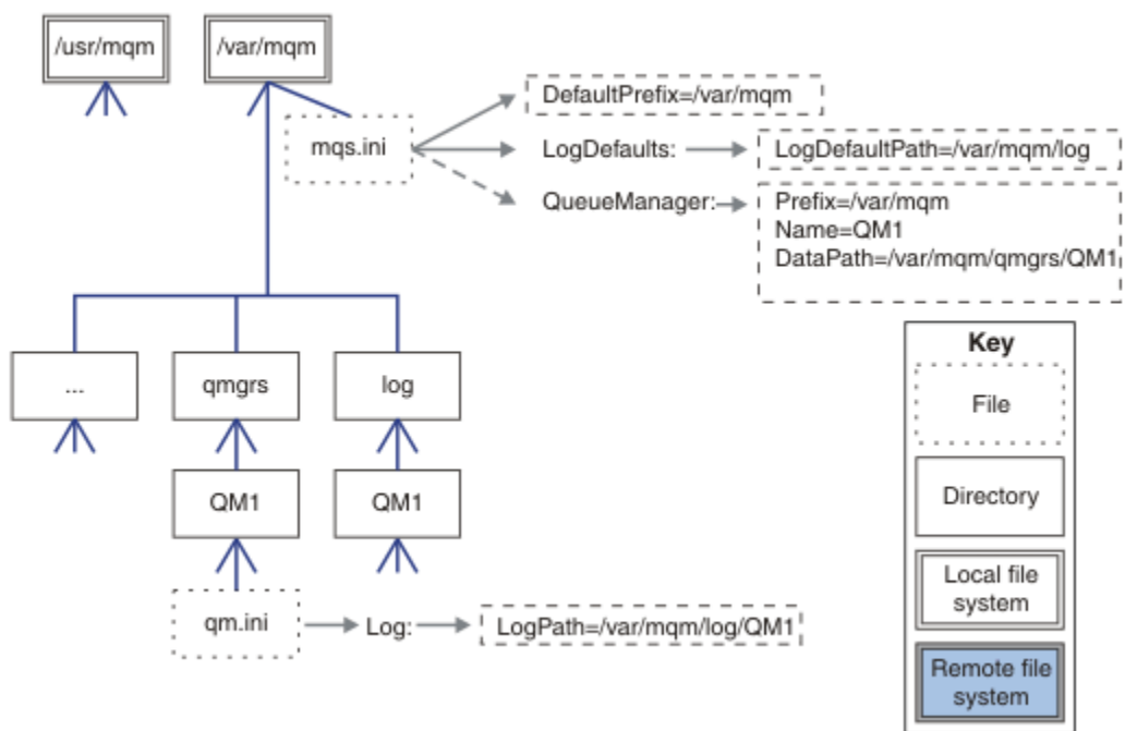
Figura 37. Exemplo de estrutura de diretórios padrão do IBM MQ para os sistemas UNIX and Linux
