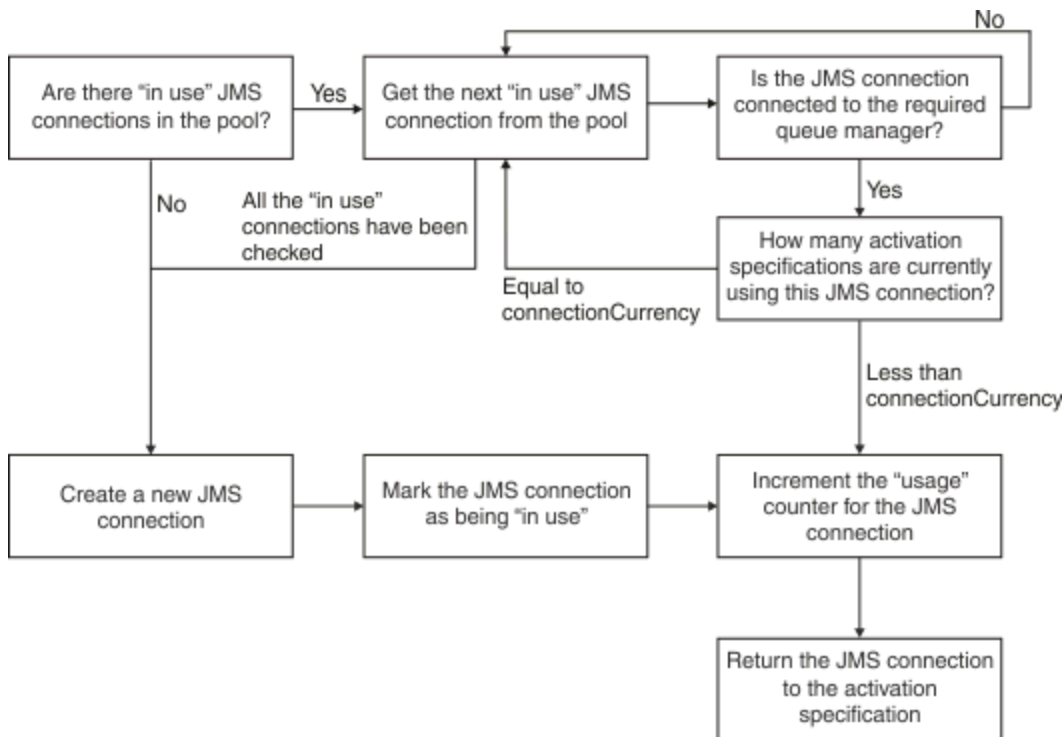
Figura 49. WebSphere Application Server V7.5 e V8.0 - como o conjunto de conexões funciona
