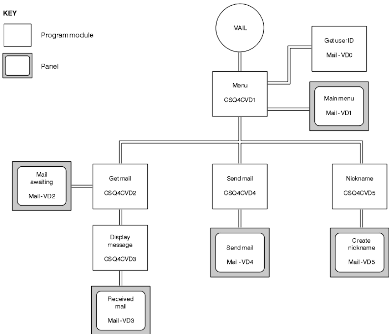
Figura 146. Programas e painéis para a versão do CICS do Mail Manager
