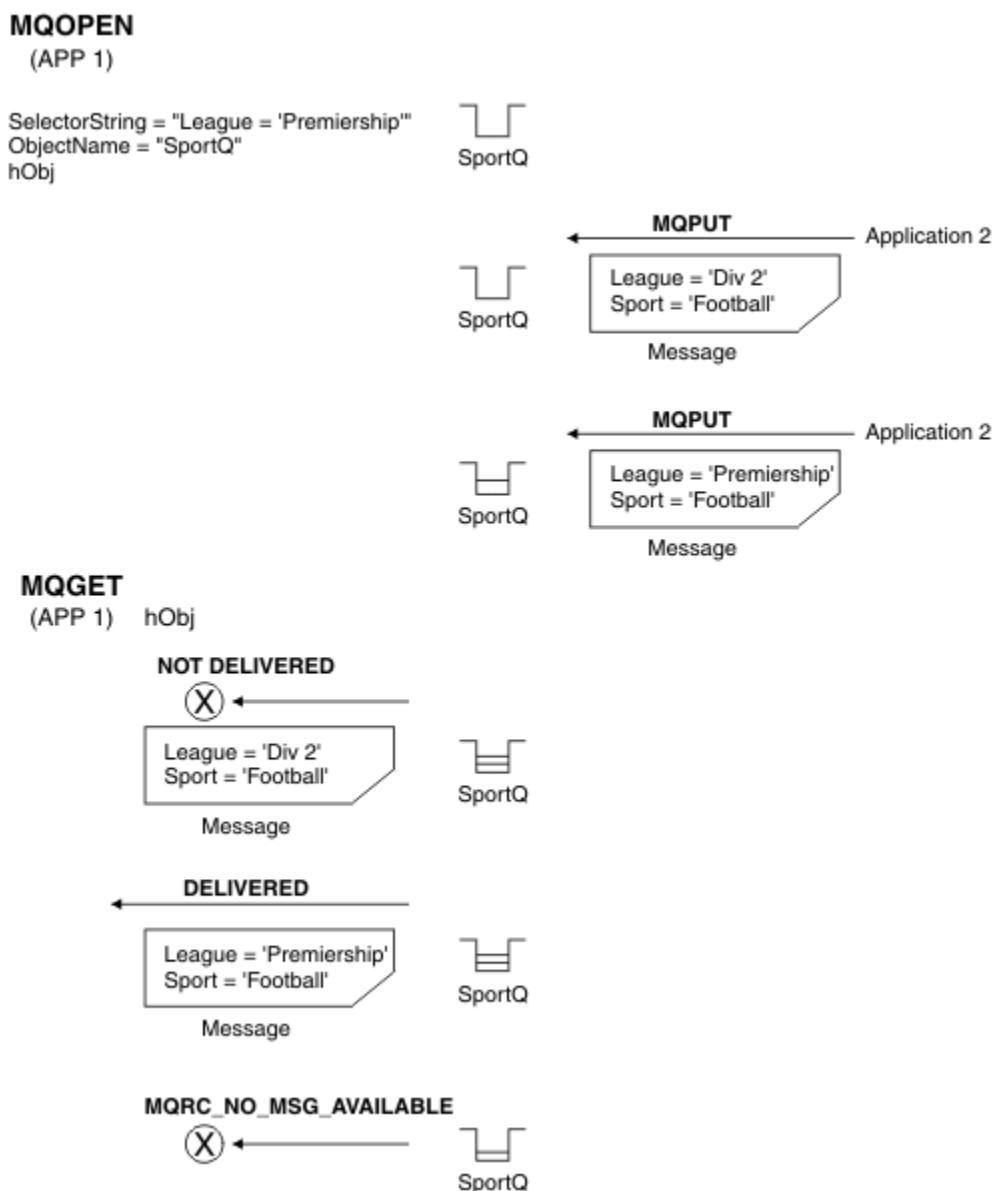
Figura 4. Seleção usando a chamada MQOPEN
