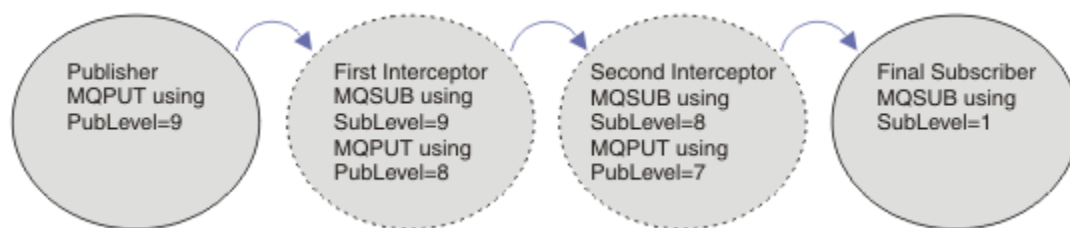
Figura 91. Sequência de assinantes de interceptação
