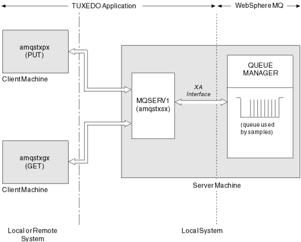
Figura 143. Como as amostras do TUXEDO funcionam juntas
