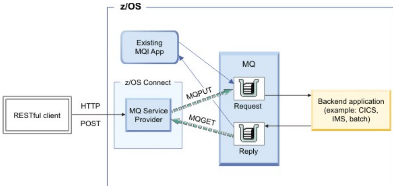
Figura 50. Serviço bidirecional
