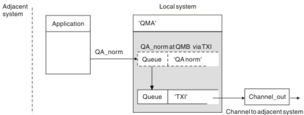
Rysunek 9. Definicja kolejki zdalnej umożliwia użycie innej kolejki transmisji
