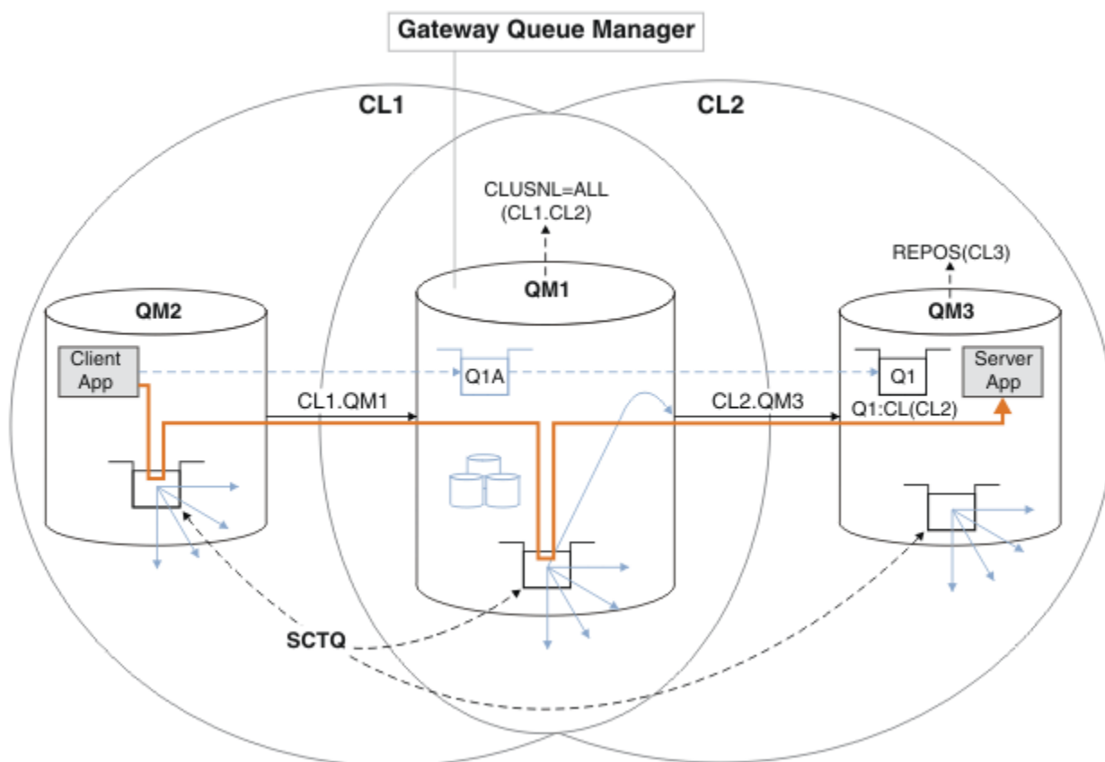
Rysunek 49. Aplikacja klient-serwer wdrażana w architekturze gwiazdистой przy użyciu klastrów IBM MQ
