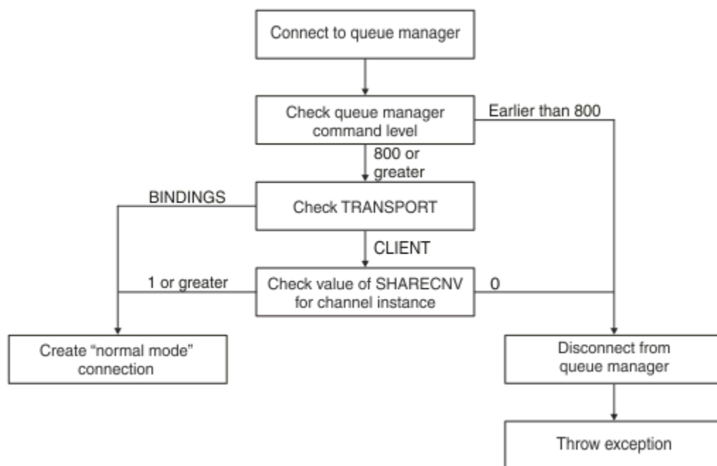
Rysunek 92. Tryb normalny PROVIDERVERSION
