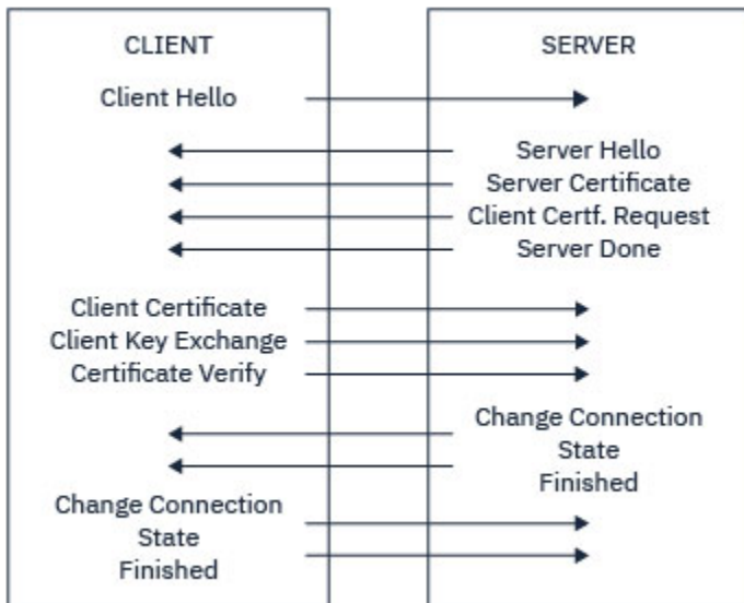
그림 5. TLS 데이터 교환의 개요
