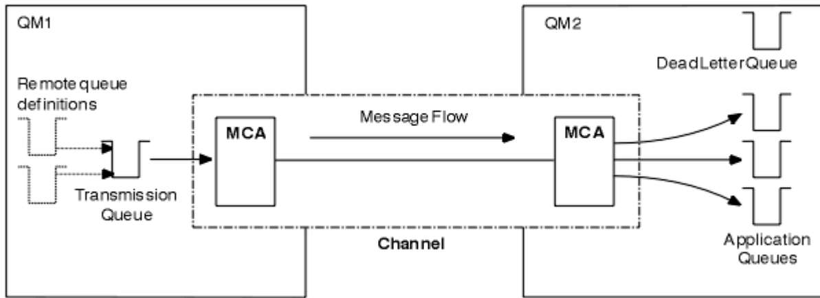
그림 3. 분산 큐잉
