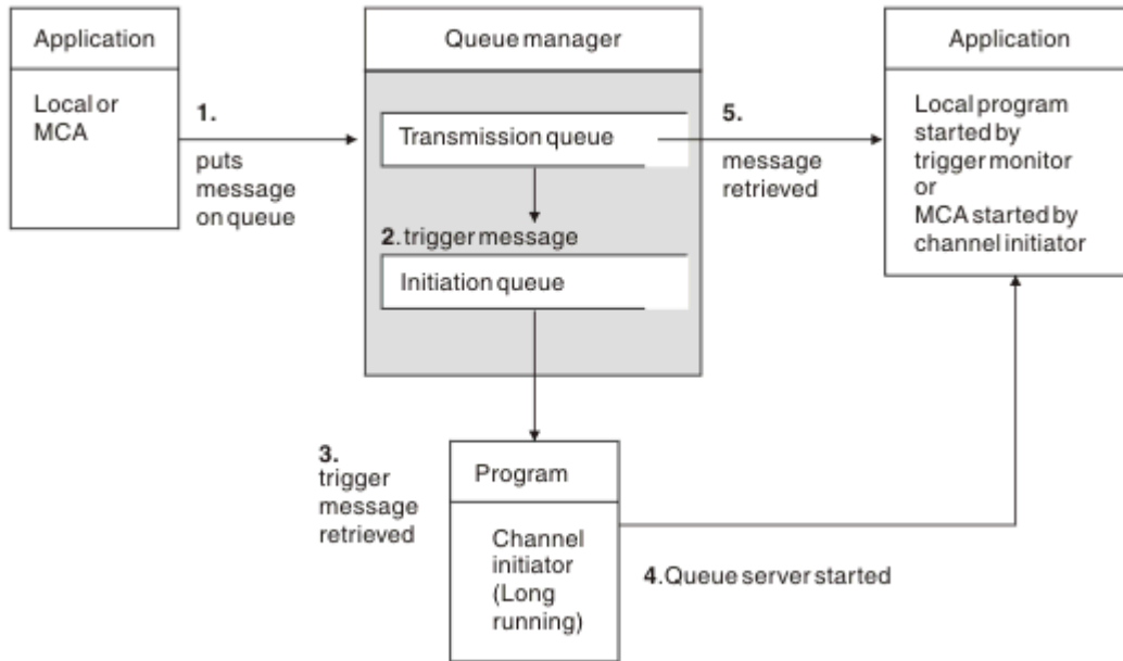
그림 26. 트리거의 개념
