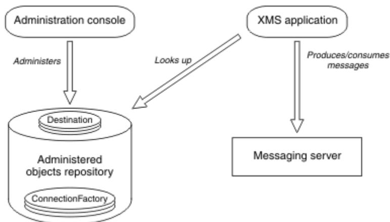
図 59. XMS アプリケーションによる管理対象オブジェクトの標準的な使用方法
