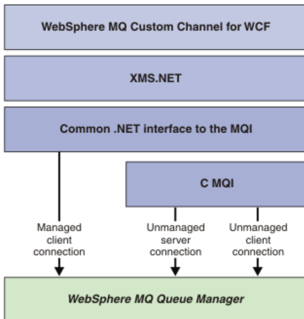
図 154. SOAP/JMS インターフェース対応の WCF アーキテクチャー
