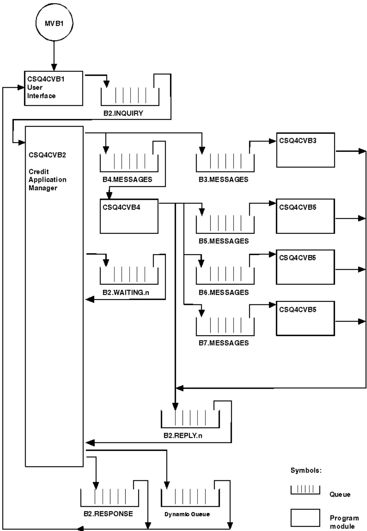
図 150. 信用小切手サンプル・アプリケーションのプログラムとキュー (COBOL プログラムのみ)
