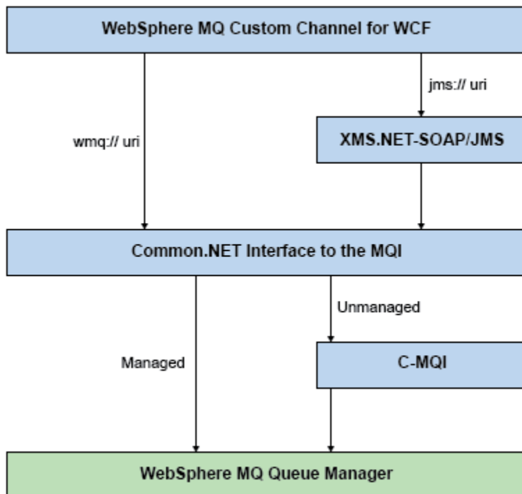
図 155. 非 SOAP/非 JMS インターフェース対応の WCF アーキテクチャー
