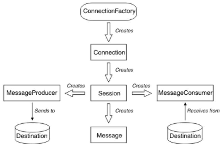
図 9. JMS オブジェクトとその関係
