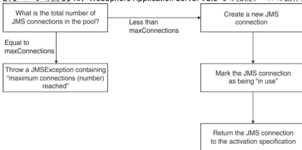
図 50. WebSphere Application Server V8.5 - 接続プールの動作方法
