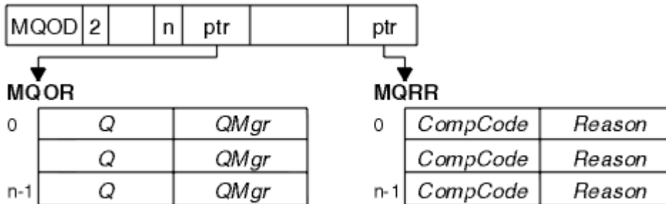
図 62. C による配布リストのオープン
