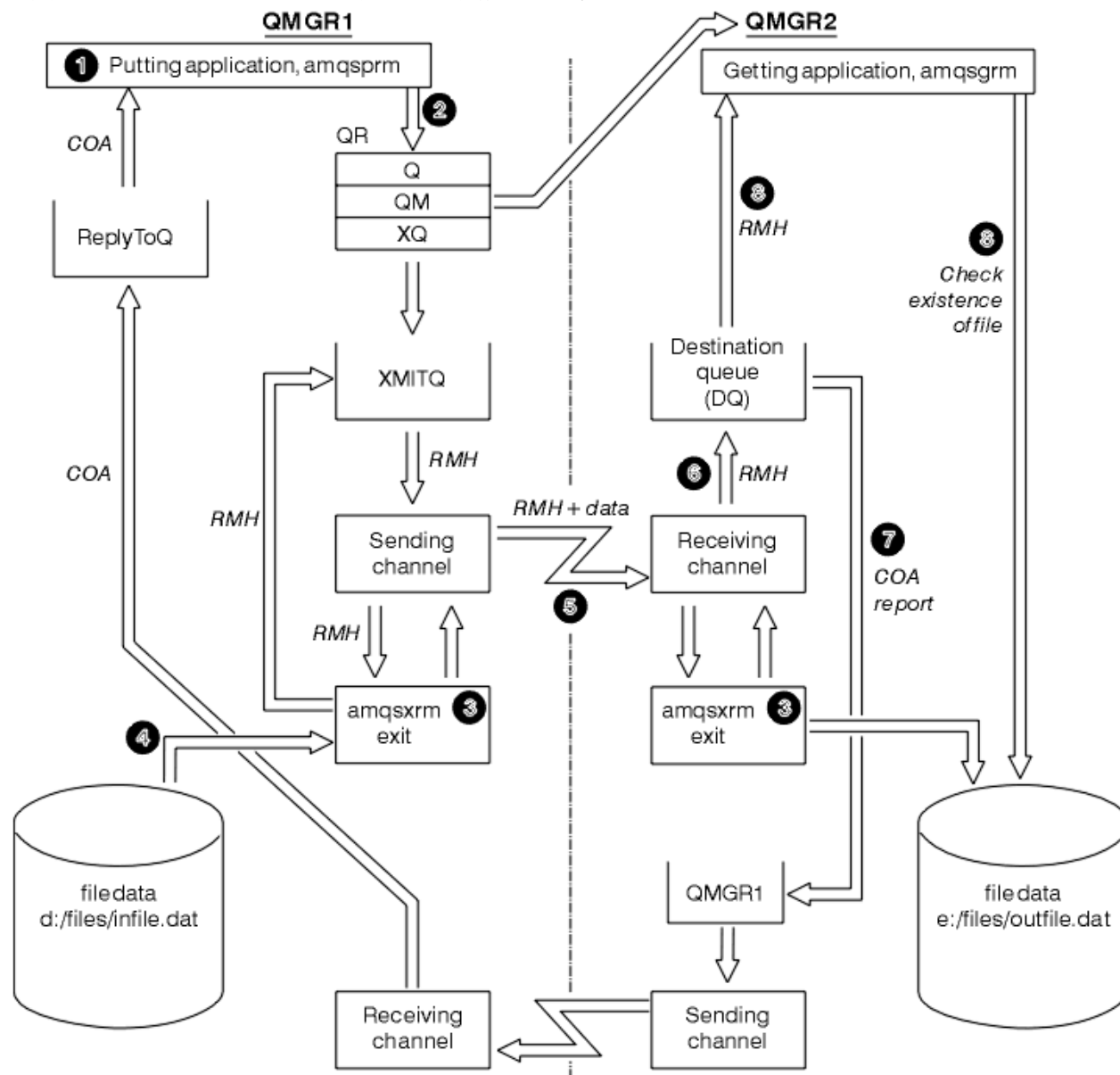
図 136. 参照メッセージ・サンプルの実行
