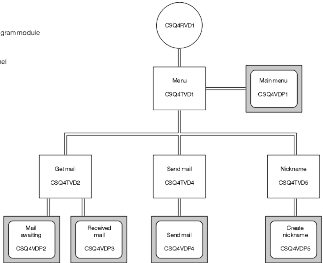
図 145. TSO バージョンのメール管理プログラムのプログラムとパネル
