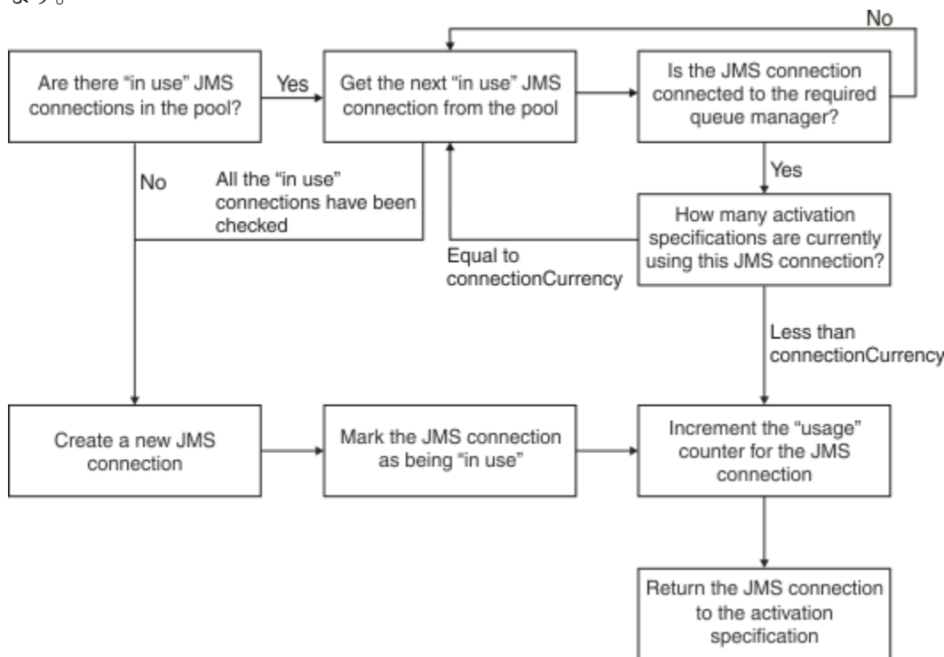
図 49. WebSphere Application Server V7.5 および V8.0 - 接続プールの動作方法
