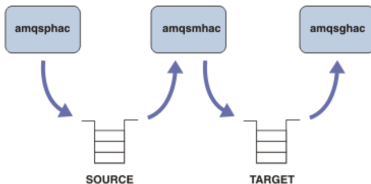
図 134. 再接続可能クライアントのサンプル
