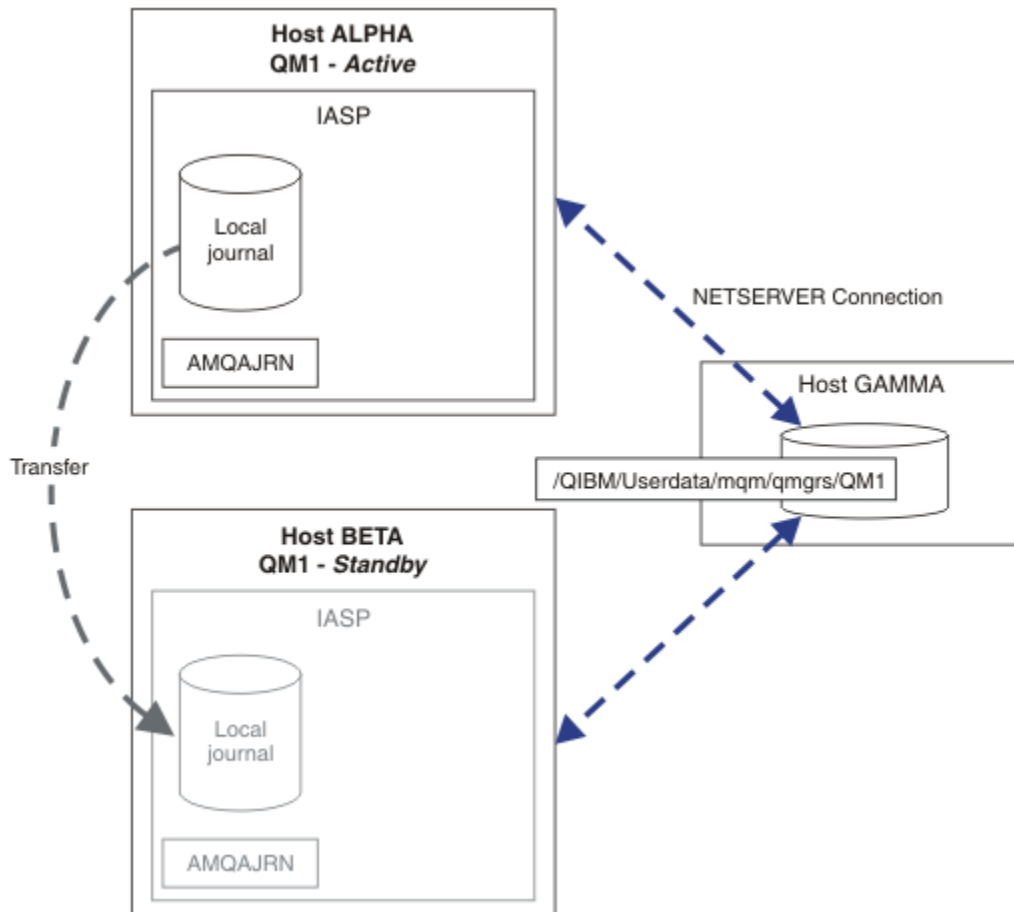
図 34. 独立 ASP を使ったキュー・マネージャー・ジャーナルの転送
