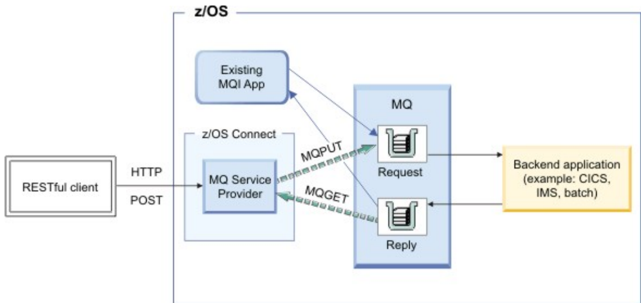
図 50. 両方向サービス
