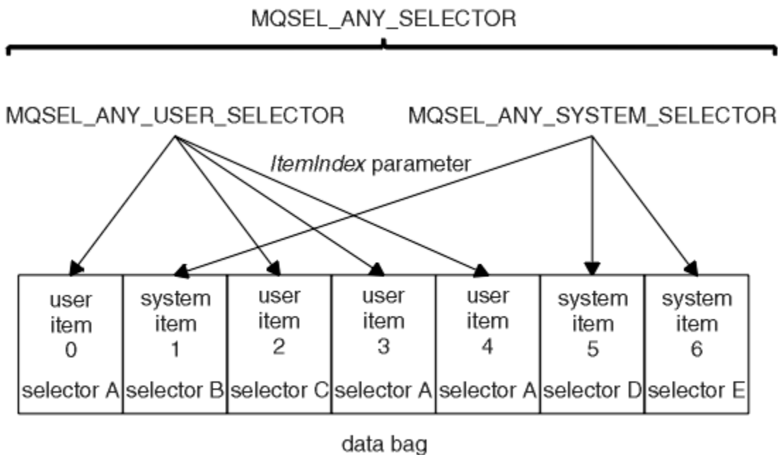
図 3. 索引付け
