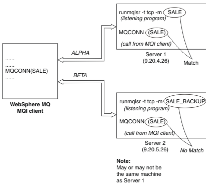
Figura 103. Esempio MQCONN
