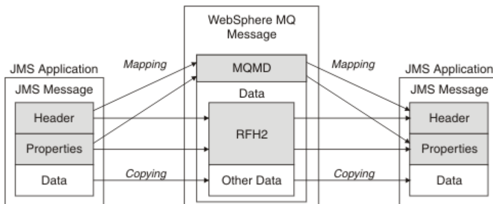
Figura 10. Come vengono trasformati i messaggi tra JMS e IBM MQ utilizzando l'intestazione MQRFH2
