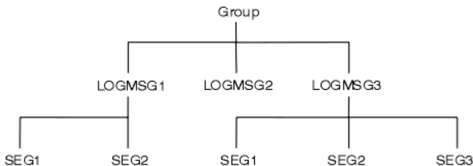
Figura 8. Messaggi segmentati
