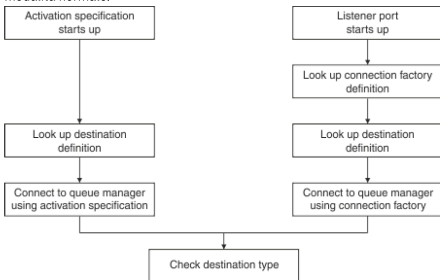
Figura 47. Modalità normale
