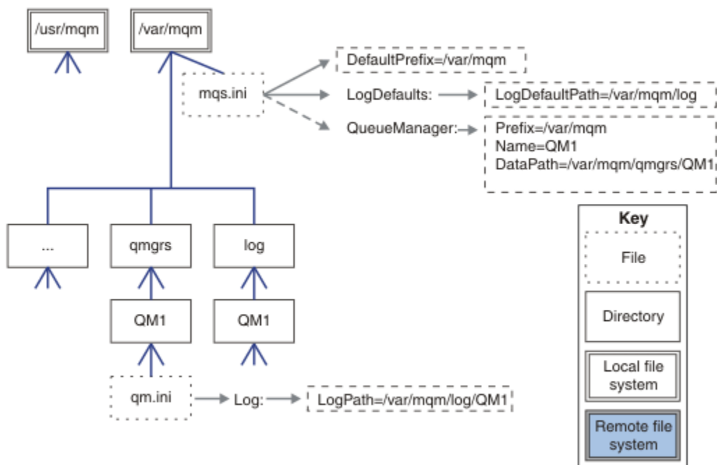
Figure 35. Exemple de structure de répertoire IBM MQ par défaut pour les systèmes UNIX and Linux
