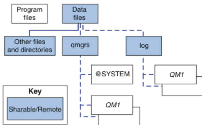
Figure 32. Vue d'ensemble de la structure de répertoire IBM MQ
