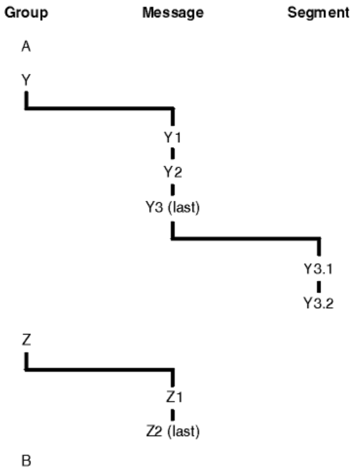
Figure 66. Ordre logique dans une file d'attente
