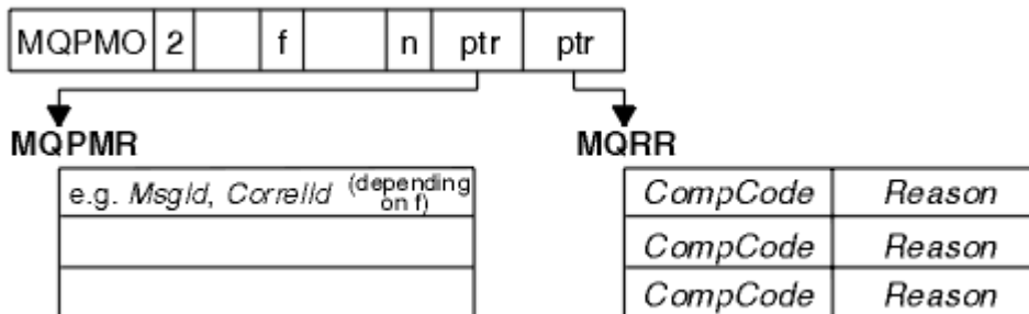
Figure 64. Insertion d'un message dans une liste de distribution en C
