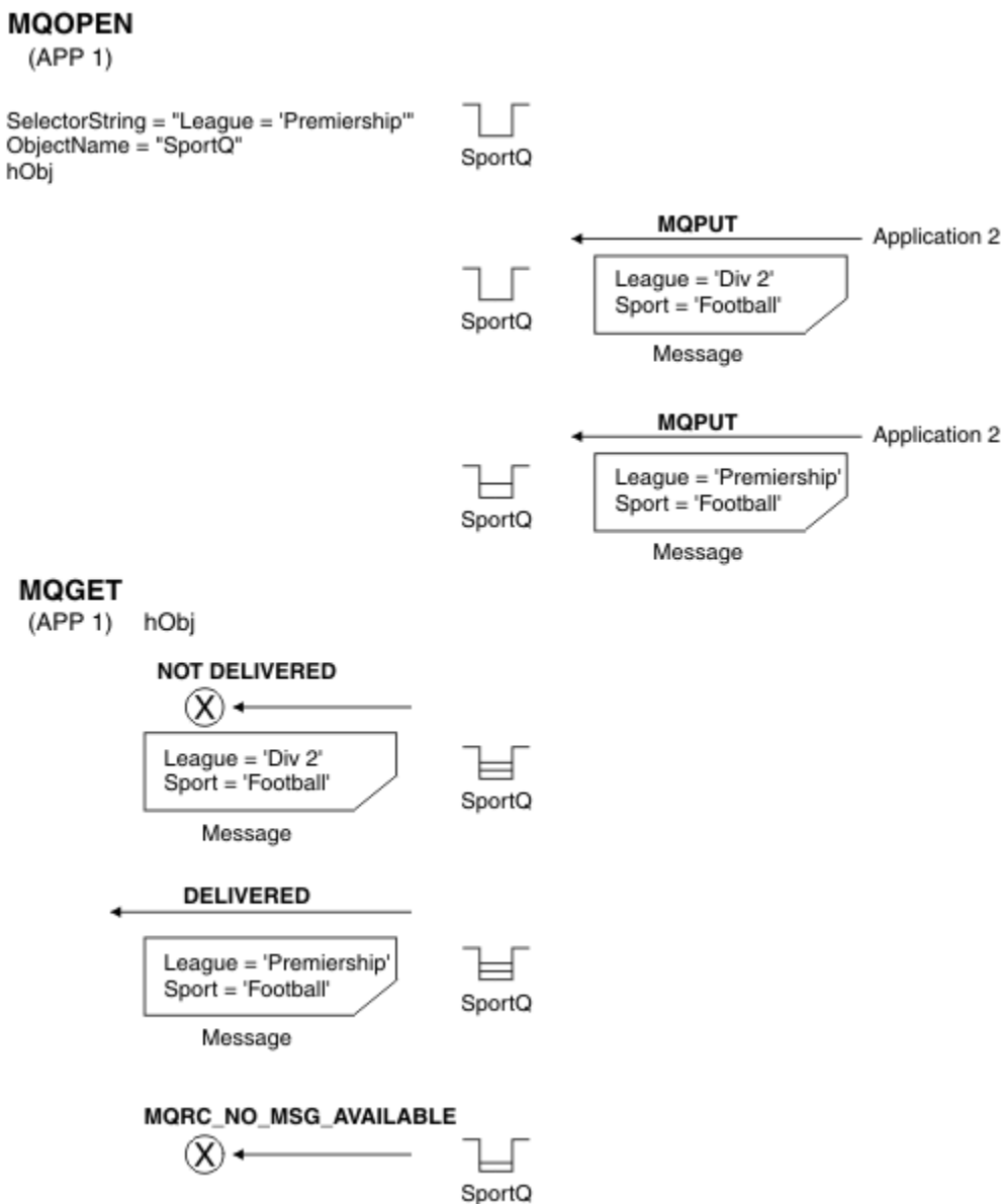
Figure 4. Sélection à l'aide de l'appel MQOPEN
