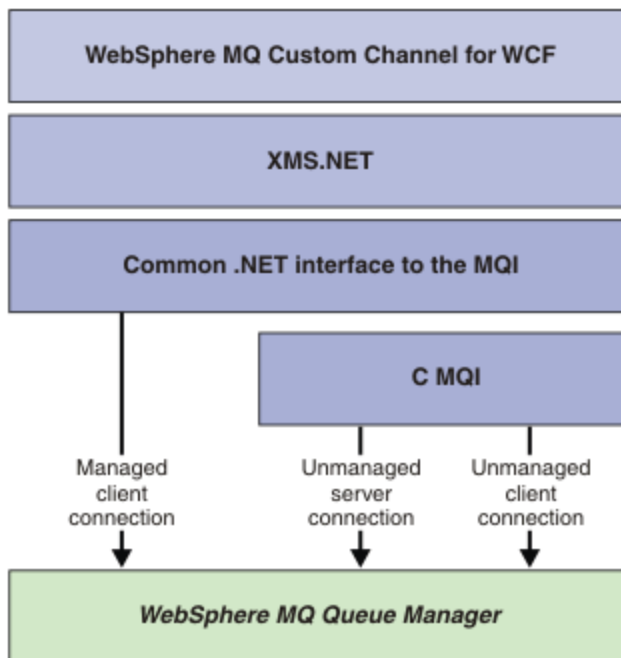
Figure 154. Architecture WCF pour l'interface SOAP/JMS
