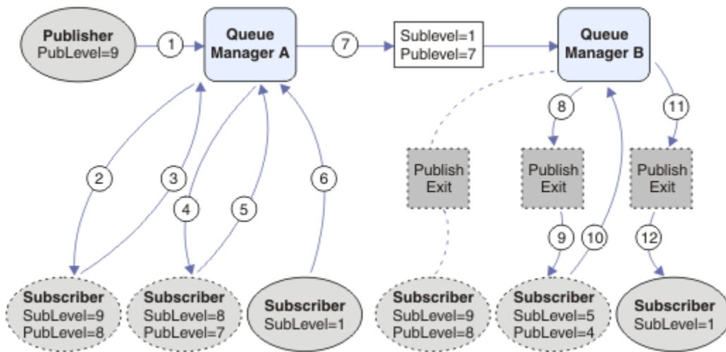
Figure 99. Déploiement complexe de l'interception des abonnés
