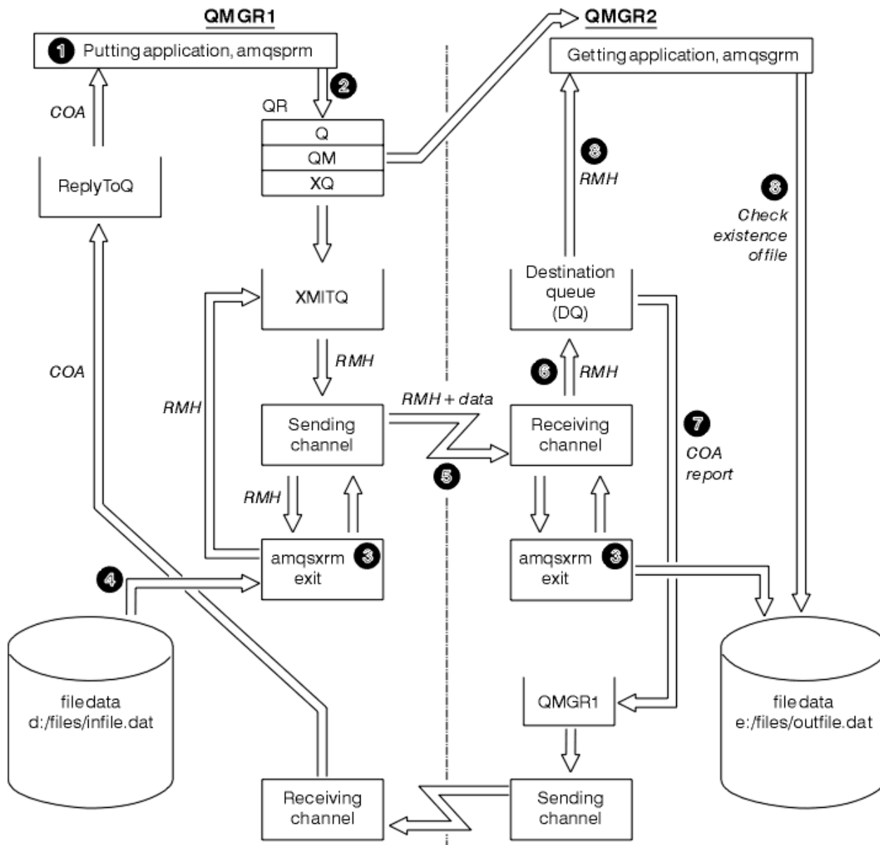
Figure 136. Exécution des exemples de message de référence
