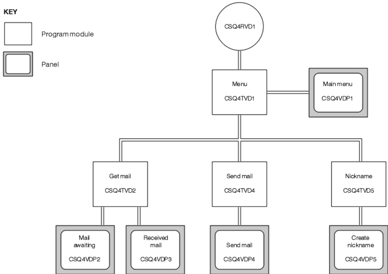
Figure 145. Programmes et panneaux pour les versions TSO du gestionnaire de messagerie
