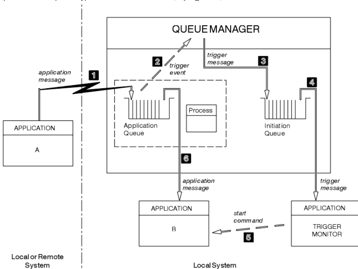
Figure 100. Flux de messages d'application et de déclenchement
