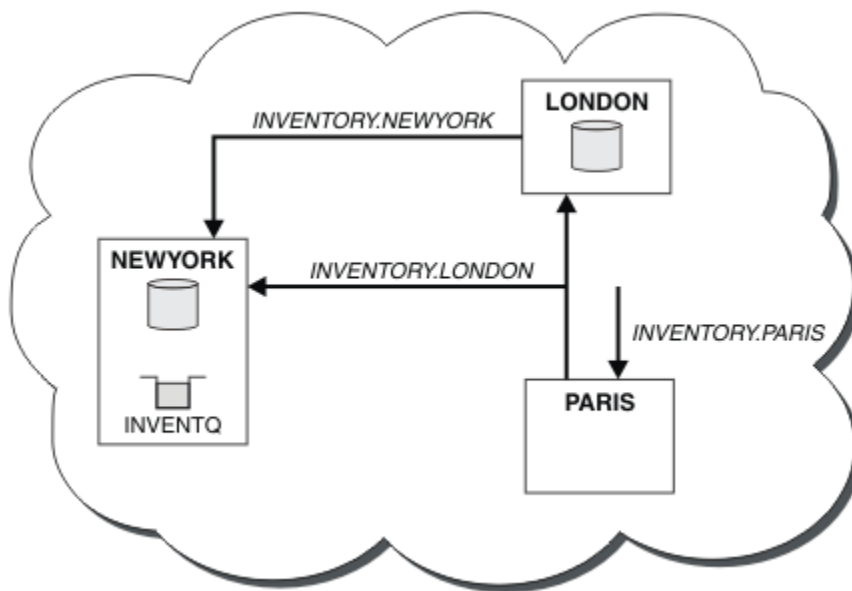
Figure 43. Cluster INVENTORY avec trois gestionnaires de files d'attente
