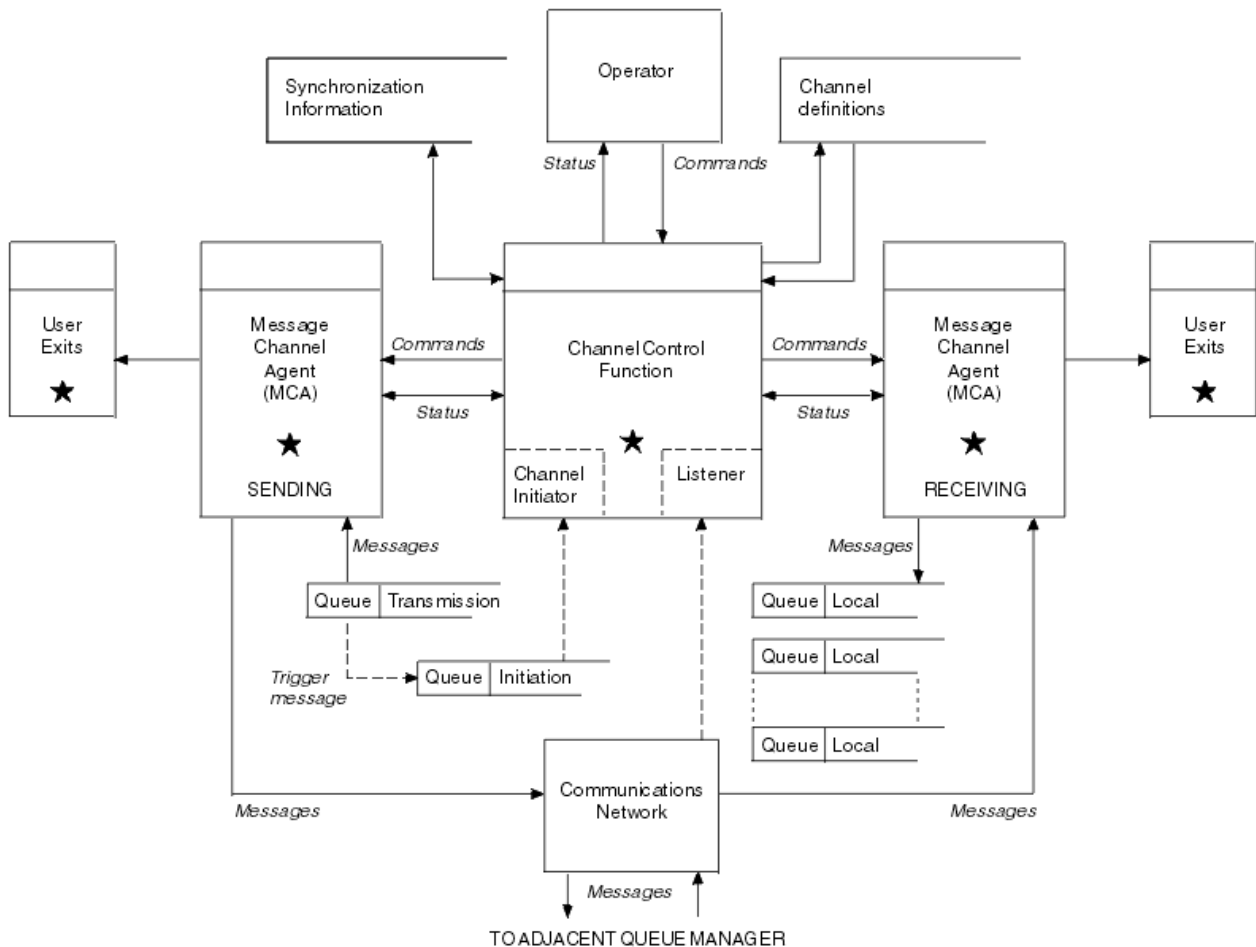
Figure 17. Modèle de gestion de files d'attente réparties
