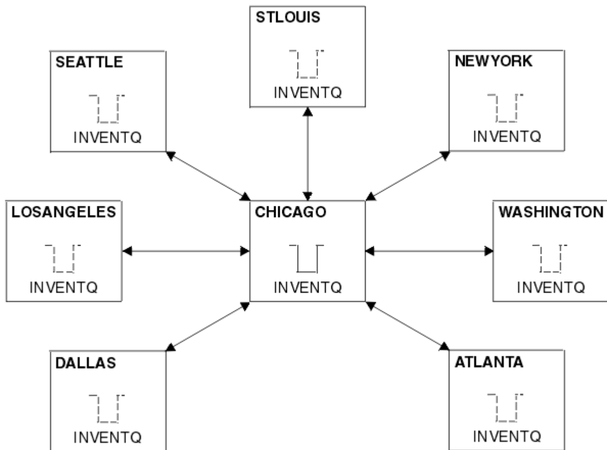
Figure 47. Un réseau concentrateur et satellite
