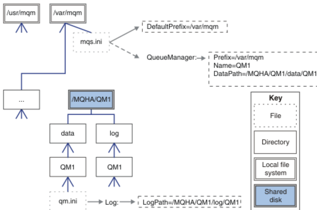
Figure 73. Répertoires data et log partagés
