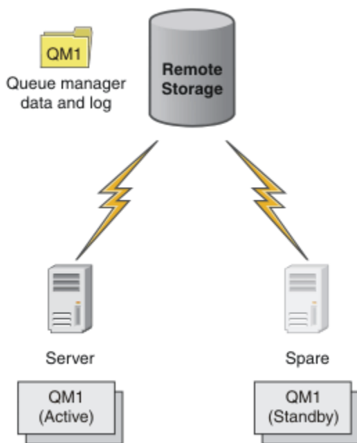
Figure 75. Gestionnaire de files d'attente multi-instance
