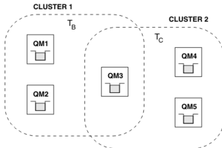
Figure 69. Clusters qui se chevauchent, espaces de sujet qui ne se chevauchent pas
