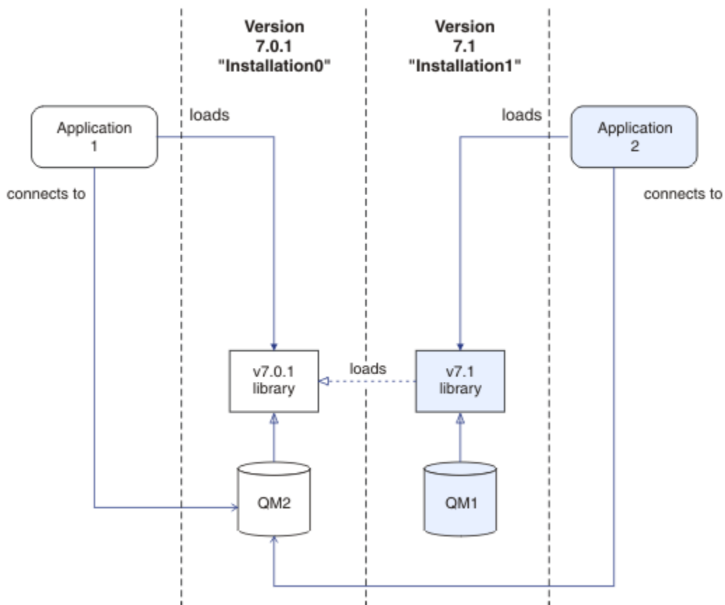
Figure 70. Connexion d'applications dans un environnement avec plusieurs installations
