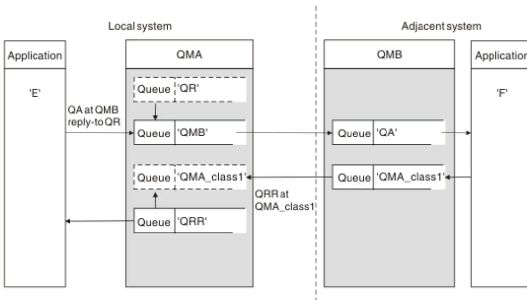
Figure 15. Substitution de nom de file d'attente de réponse lors de l'appel PUT
