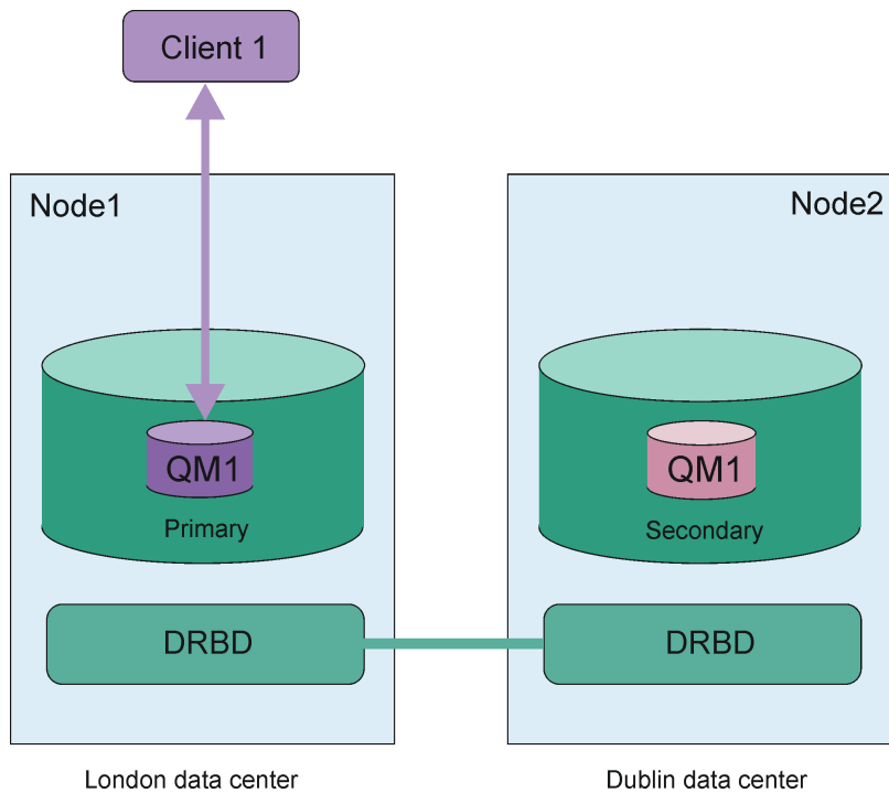
Figure 84. Paire RDQM unique
