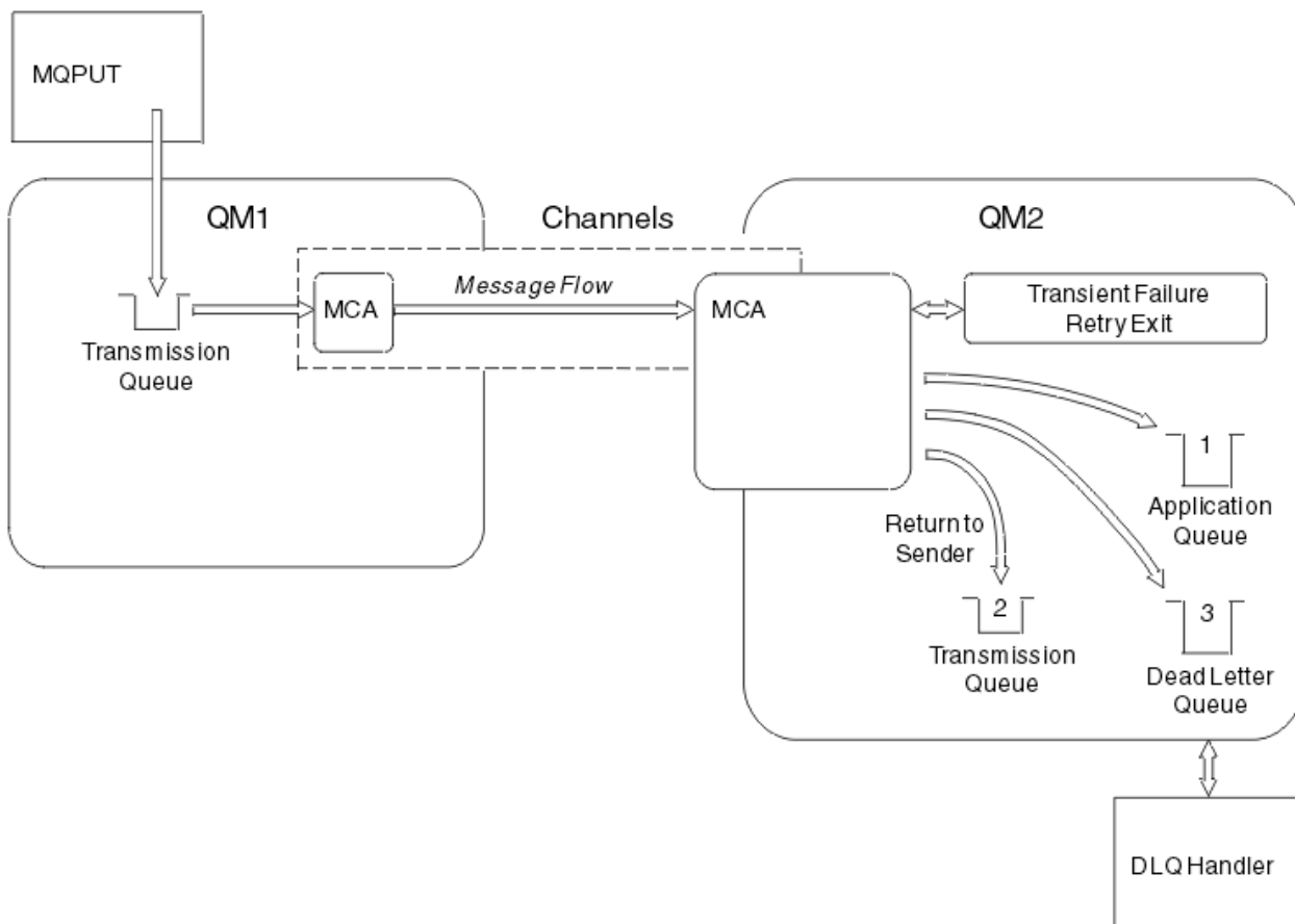
Figure 25. Que se passe-t-il lorsqu'un message ne peut pas être distribué?
