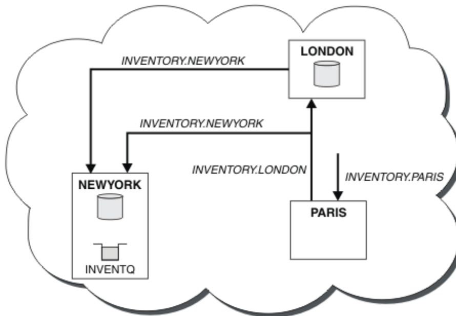
Figure 42. Le cluster INVENTORY avec trois gestionnaires de files d'attente
