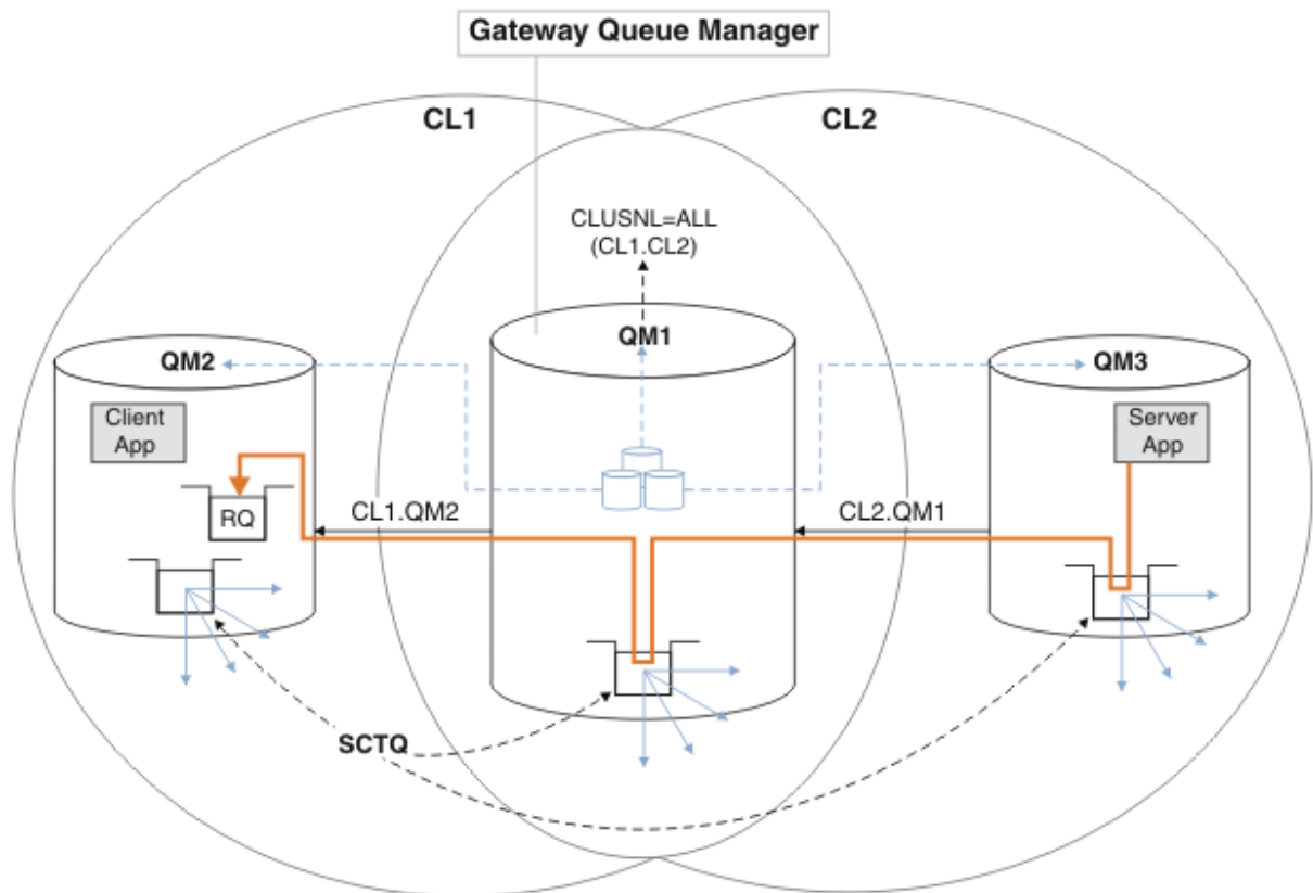
Figure 60. Utilisation d'un alias de gestionnaire de files d'attente pour renvoyer le message de réponse à un autre cluster
