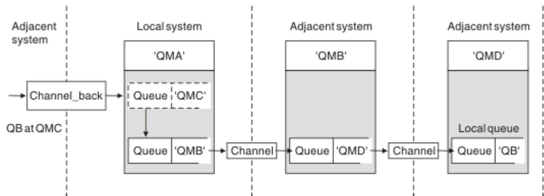
Figure 14. Détournement des flux de messages vers une autre destination
