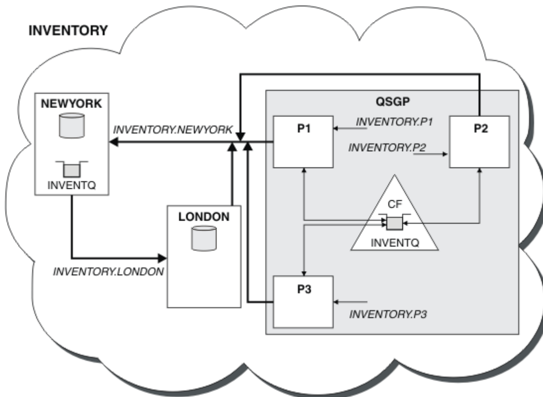
Figure 45. Cluster et groupe de partage de files d'attente
