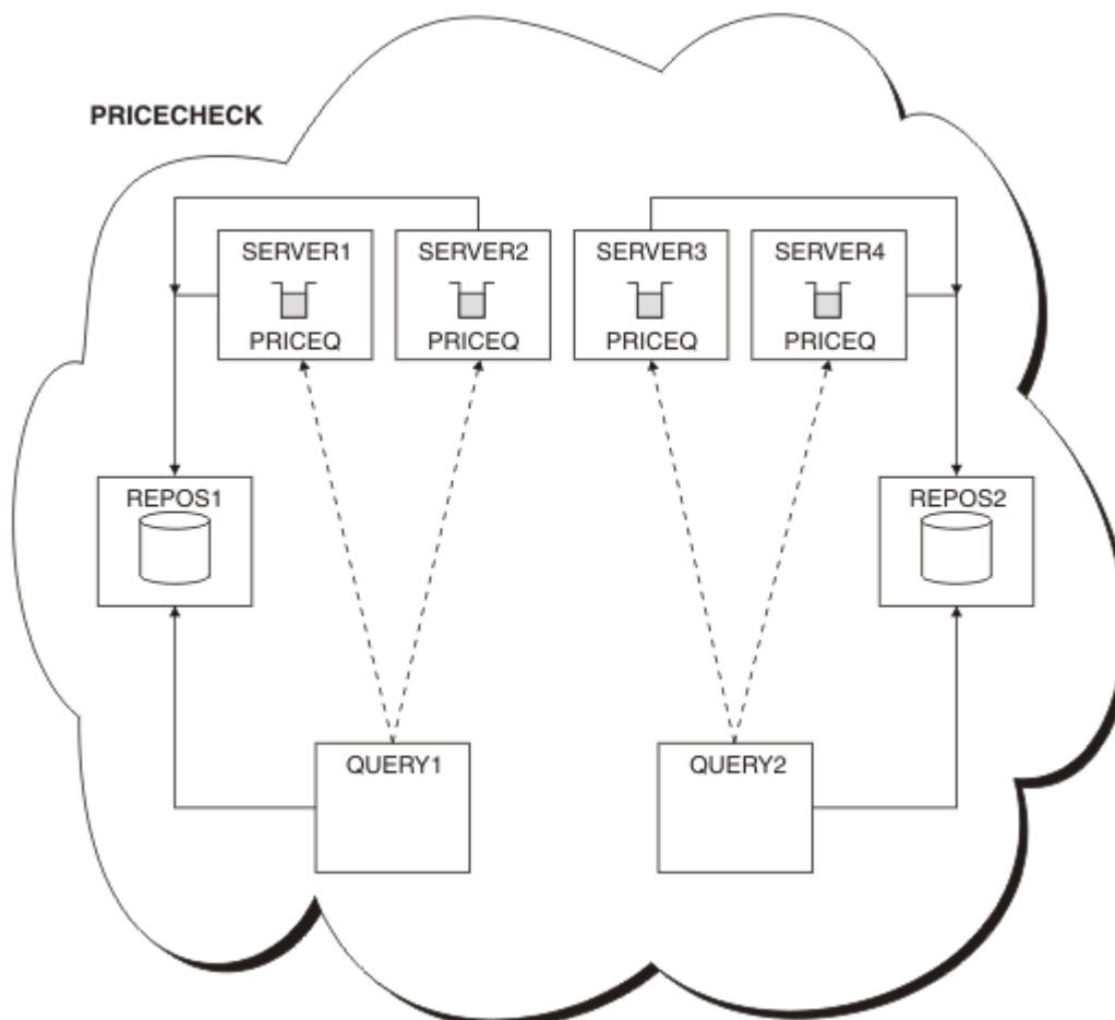
Figure 65. Le cluster PRICECHECK, avec quatre gestionnaires de files d'attente de serveur, deux référentiels et deux gestionnaires de files d'attente de requêtes
