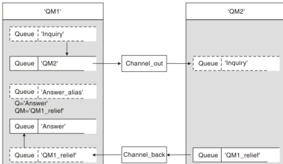
Figura 16. Ejemplo de alias de cola de respuesta
