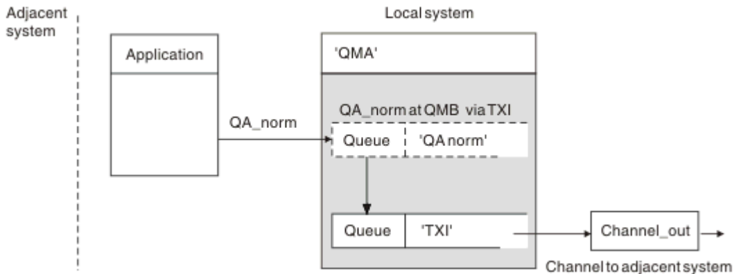
Figura 9. La definición de cola remota permite que se utilice una cola de transmisión diferente
