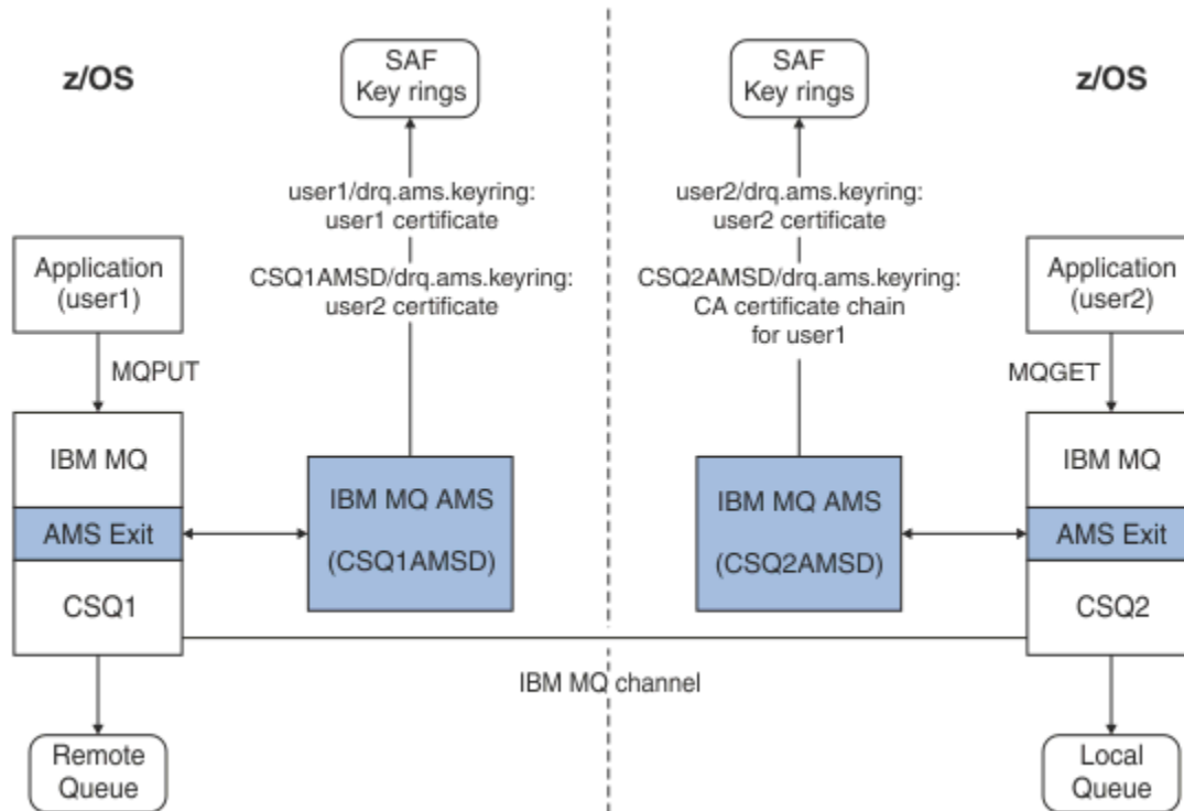
Abbildung 35. Anwendungs- und Zertifikatsbeziehungen
