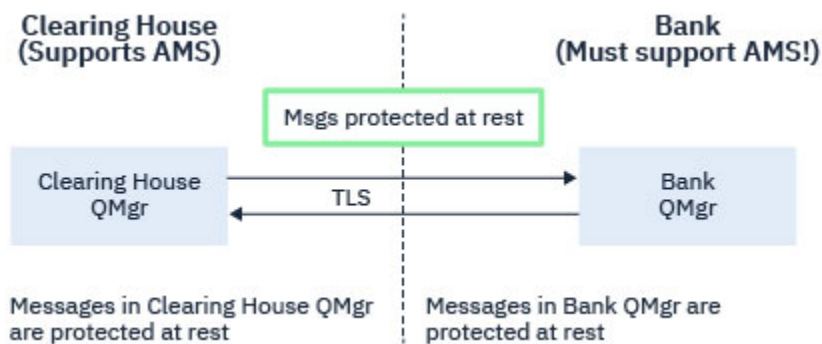
Abbildung 32. Aktuelle Verwendung von AMS
