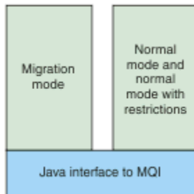
Abbildung 91. Messaging-Provider-Modi
