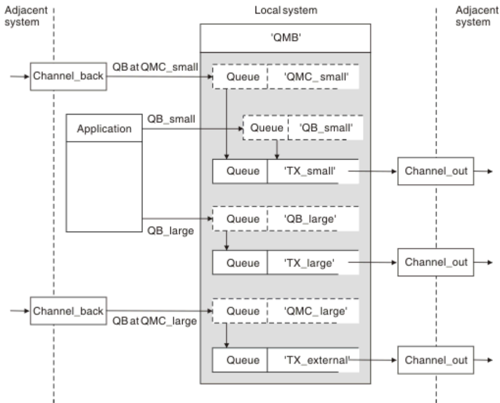
Abbildung 12. Nachrichtenflüsse trennen
