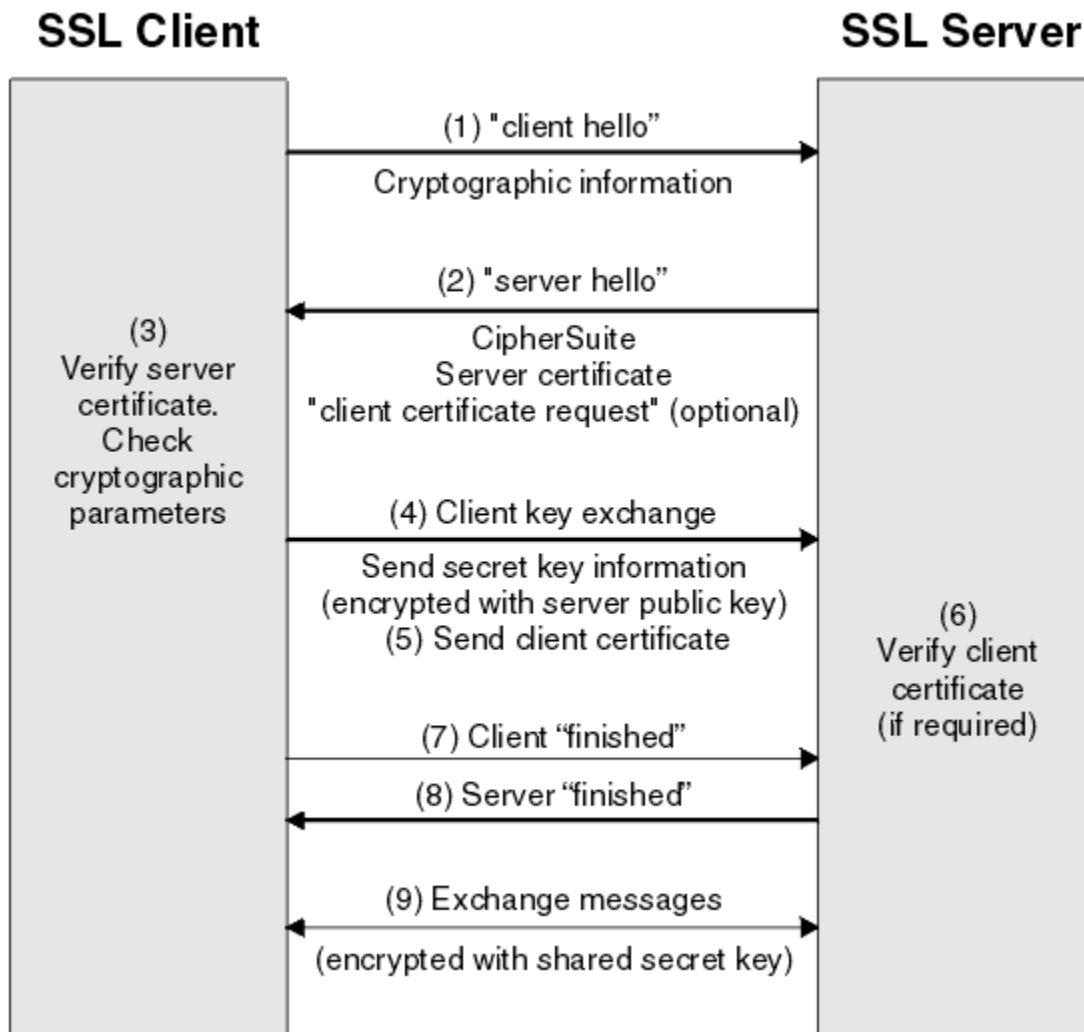
圖 5: TLS 信號交換概觀
