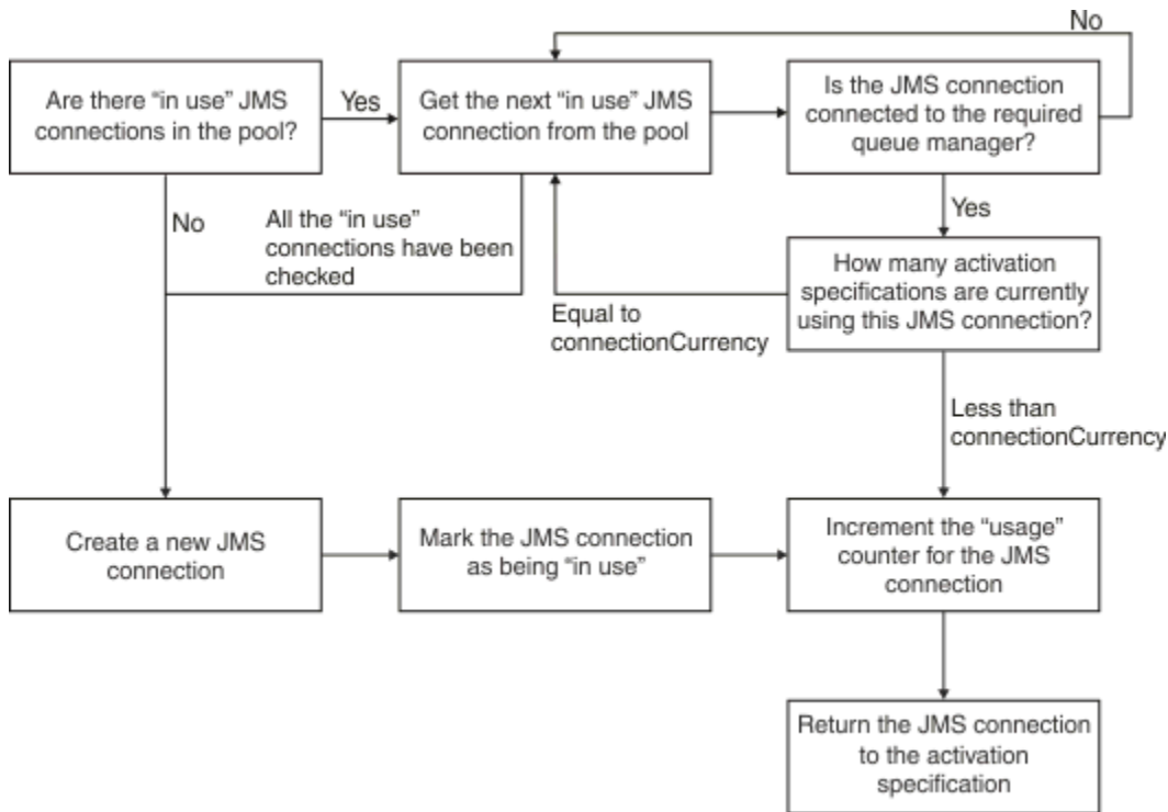
圖 49: WebSphere Application Server 7.5 和 8.0 -連線儲存區的運作方式
