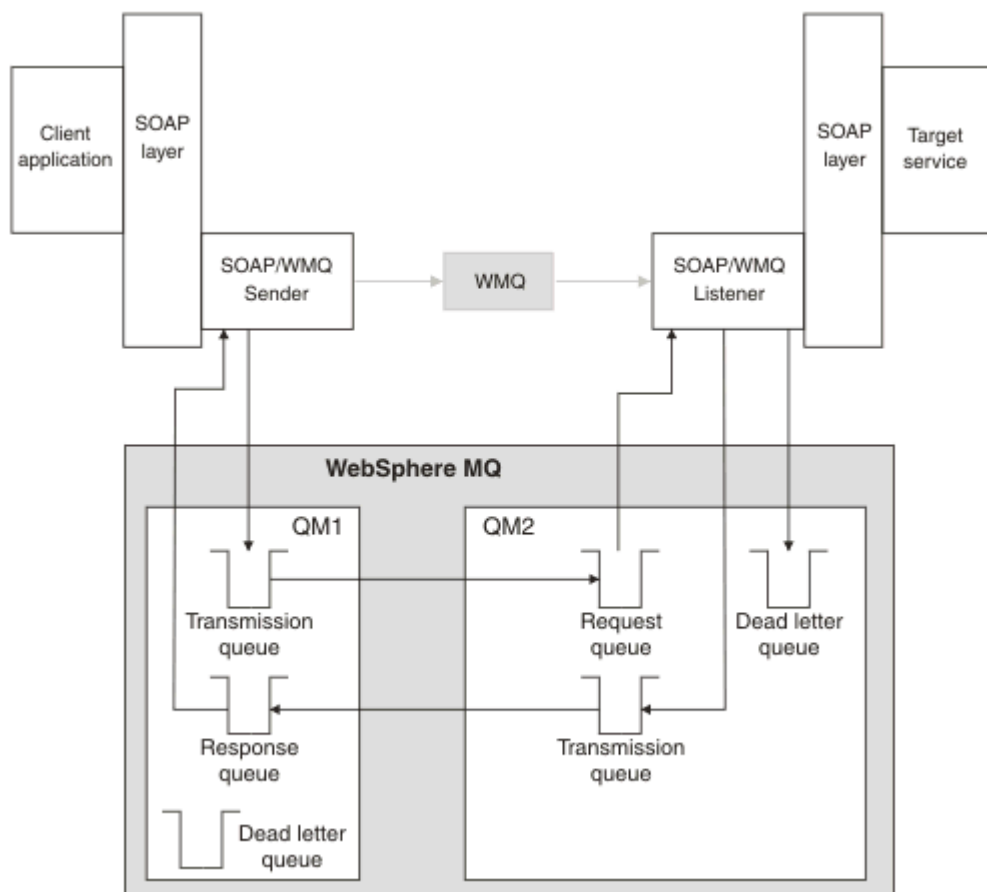
圖 166: SOAP/IBM MQ 使用的佇列 (個別佇列管理程式)
