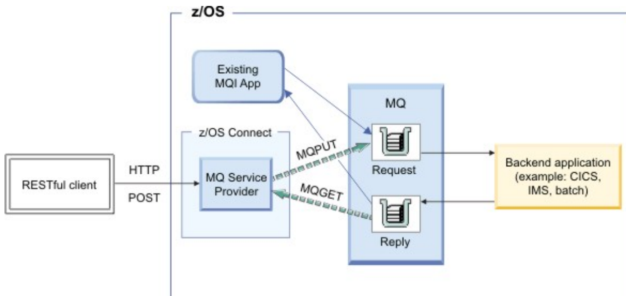
圖 56: 雙向服務
