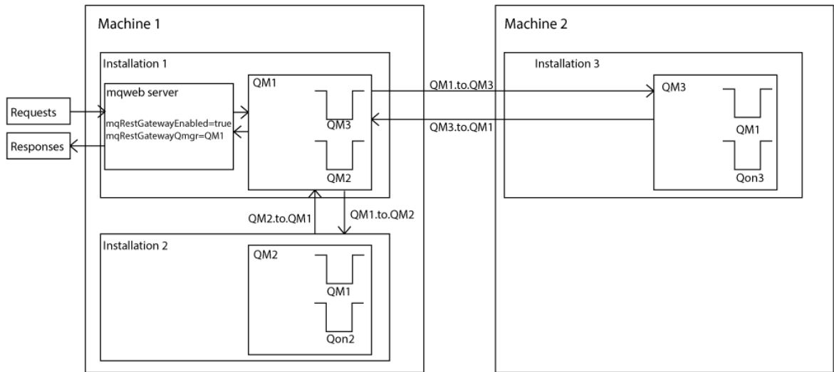
圖 15: 使用 REST API 進行遠端管理的範例配置圖。
