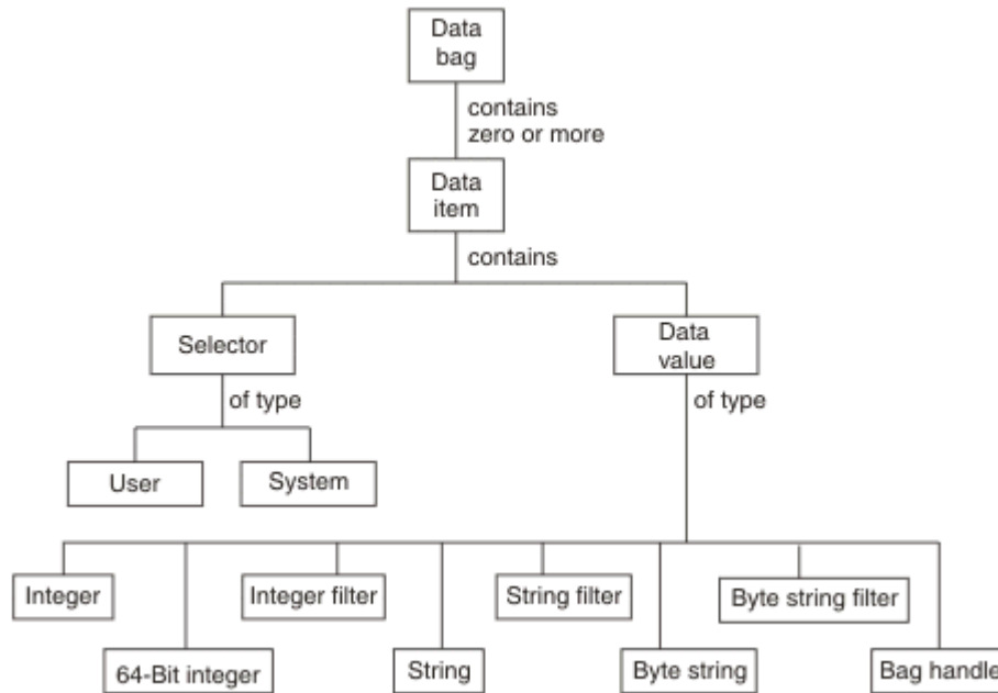
圖 5: MQAI 概念的階層
