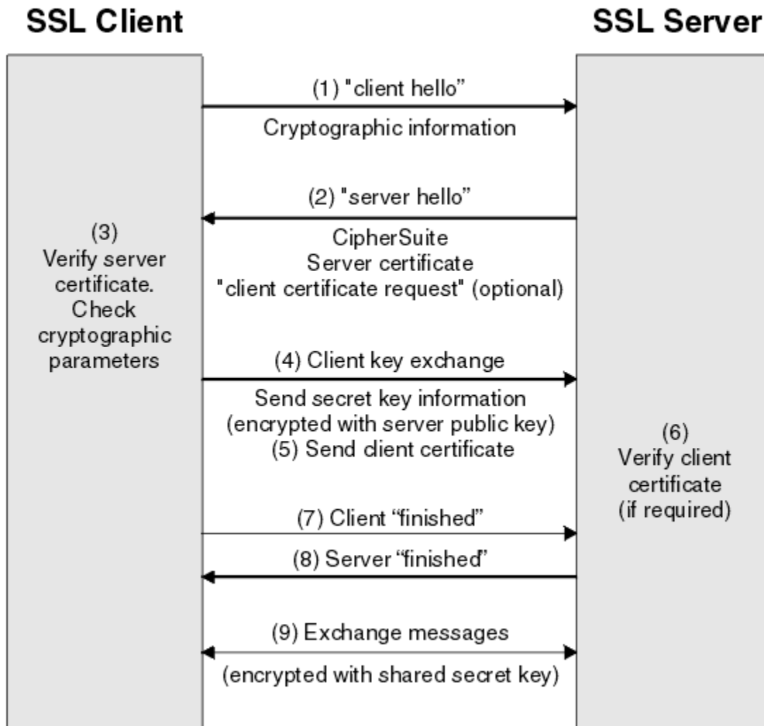
图 5: TLS 握手概述
