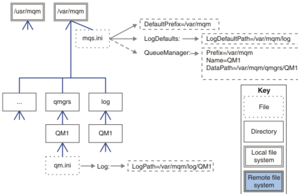
图 46: UNIX and Linux 系统的缺省 IBM MQ 目录结构示例
