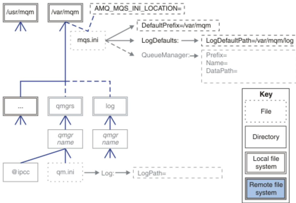
图 45: 目录结构模式模板
