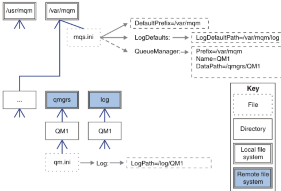
图 47: 共享 qmgrs 和 log 目录
