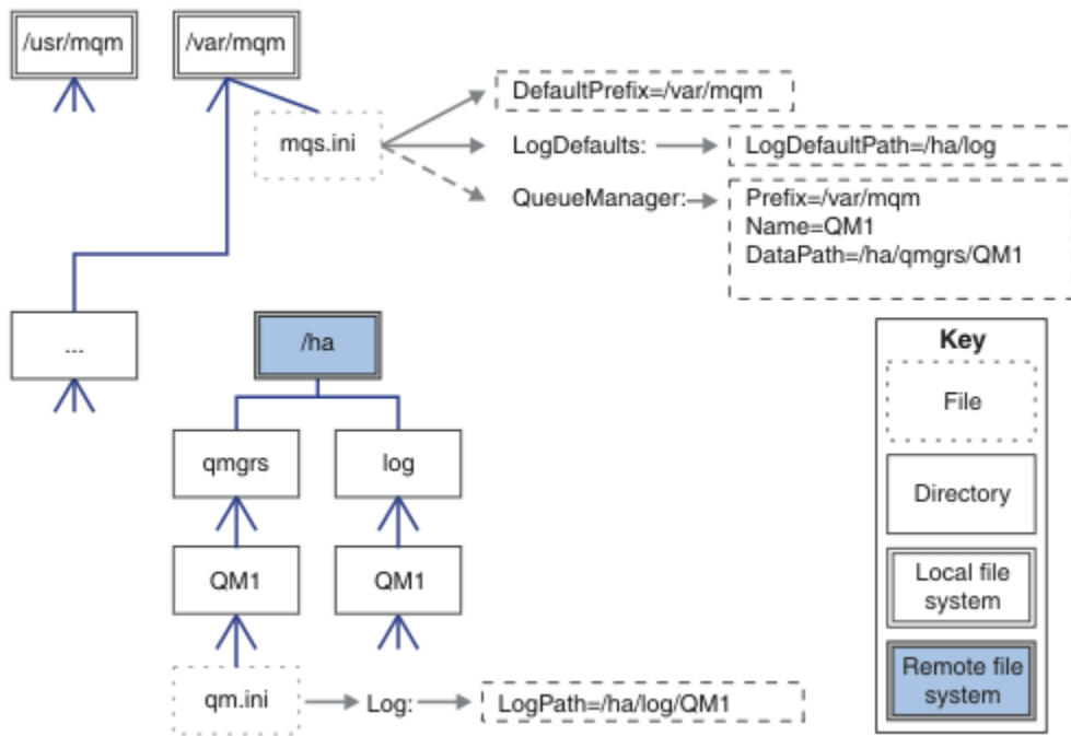
图 48: 共享名为 qmgrs 和 log 的目录
