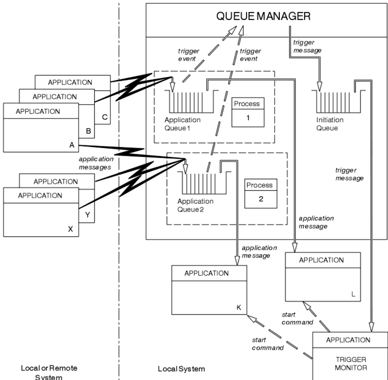
图 106: 触发内队列的关系
