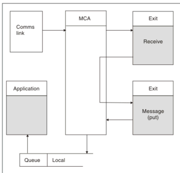
图 117: 消息通道的接收方端的接收出口示例
