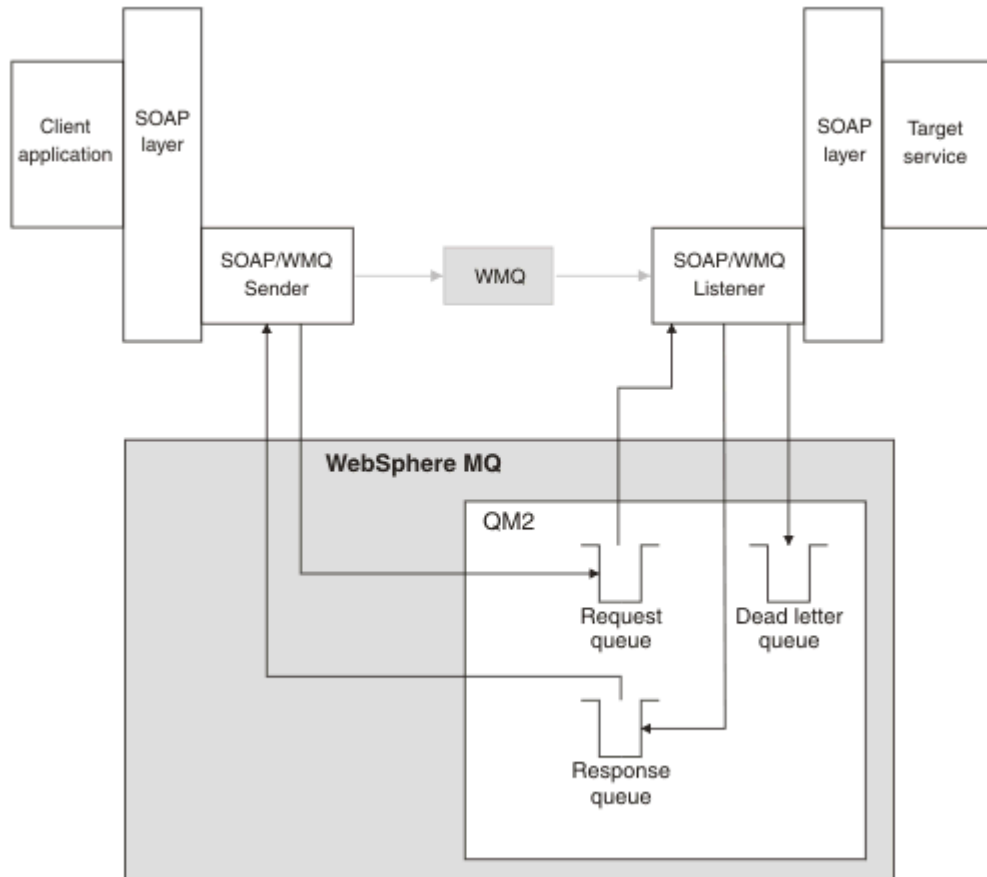
图 165: SOAP/IBM MQ 所使用的队列（单个队列管理器）
