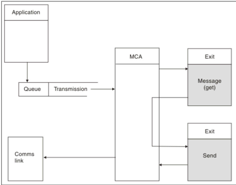
图 116: 消息通道的发送方端的发送出口示例
