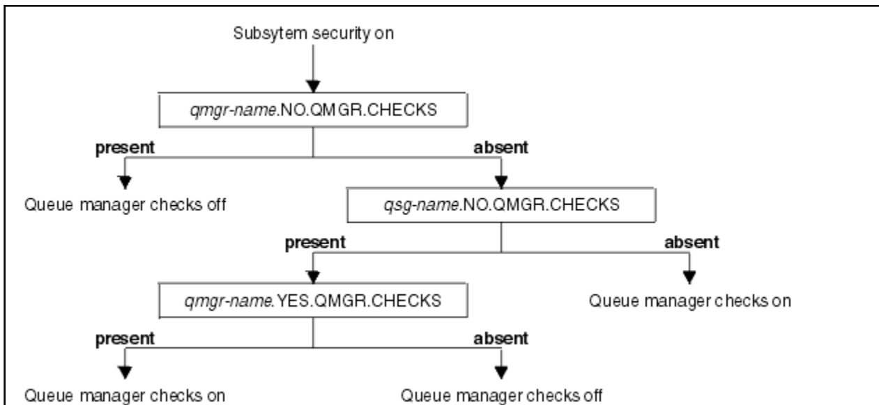
Rysunek 15. Sprawdzanie bezpieczeństwa na poziomie menedżera kolejek
