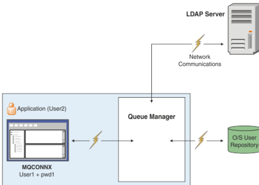
Rysunek 7. Typy obiektów informacji uwierzytelniających
