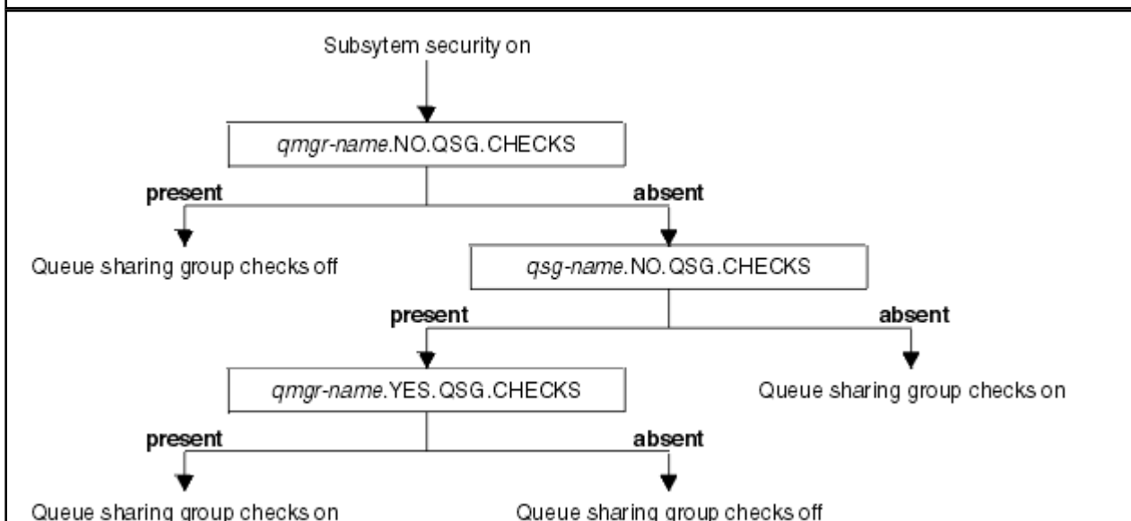
Rysunek 16. Sprawdzanie bezpieczeństwa na poziomie grupy współużytkowania kolejek
