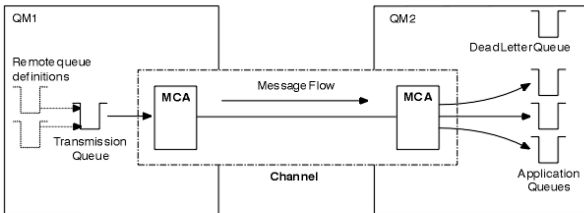
그림 3. 분산 큐잉
