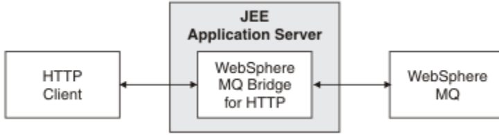
그림 59. IBM MQ bridge for HTTP
