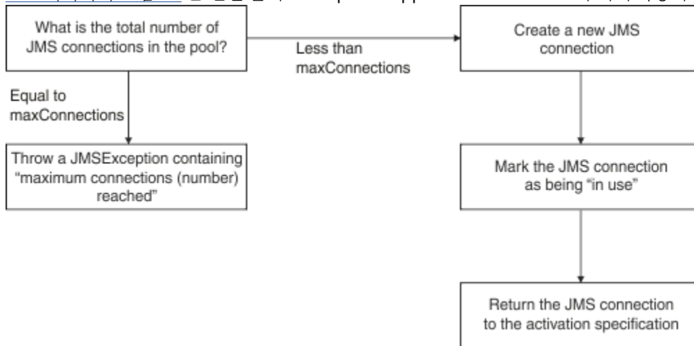
그림 50. WebSphere Application Server 8.5 -연결 풀의 작동 방식
