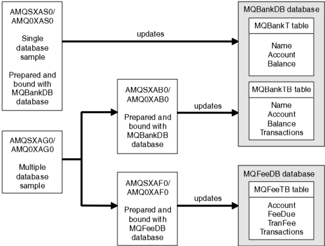
그림 140. 데이터베이스 조정 샘플
