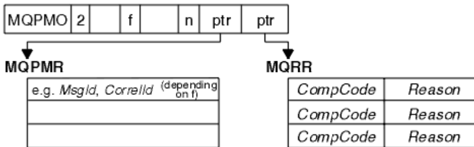
그림 69. C로 된 분배 목록에 메시지 넣기
