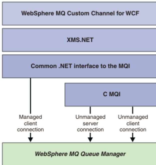
그림 161. SOAP/JMS 인터페이스용 WCF 아키텍처
