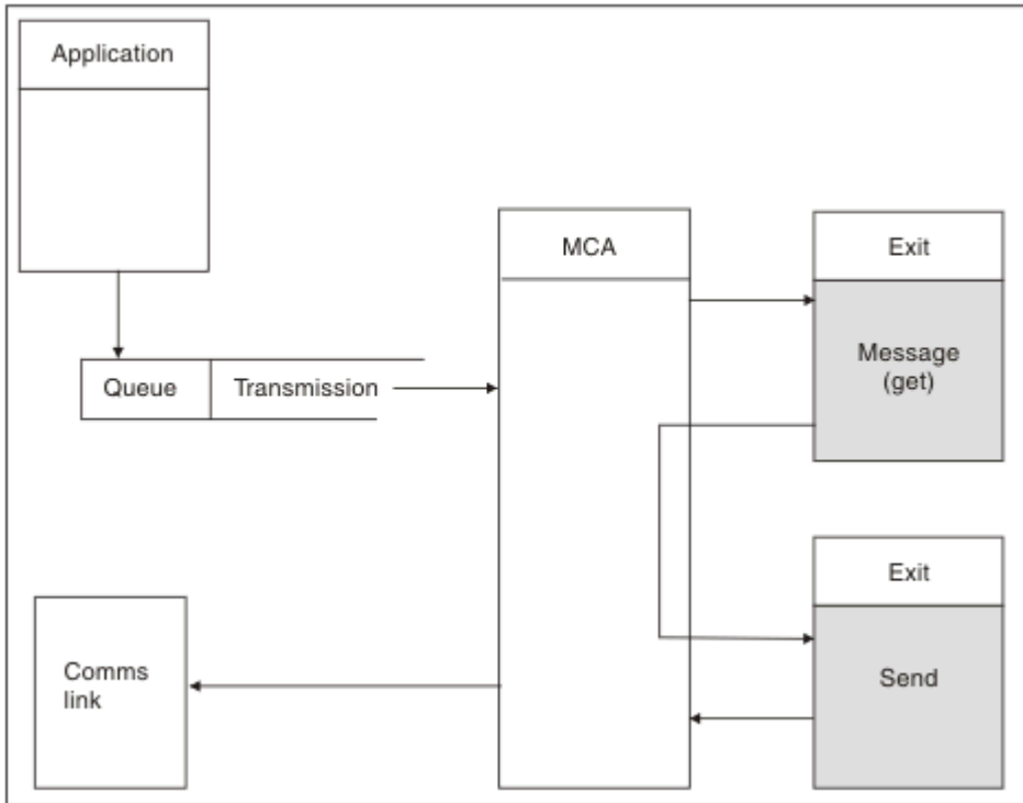
그림 116. 메시지 채널의 송신자 끝에서의 송신 엑시트의 예
