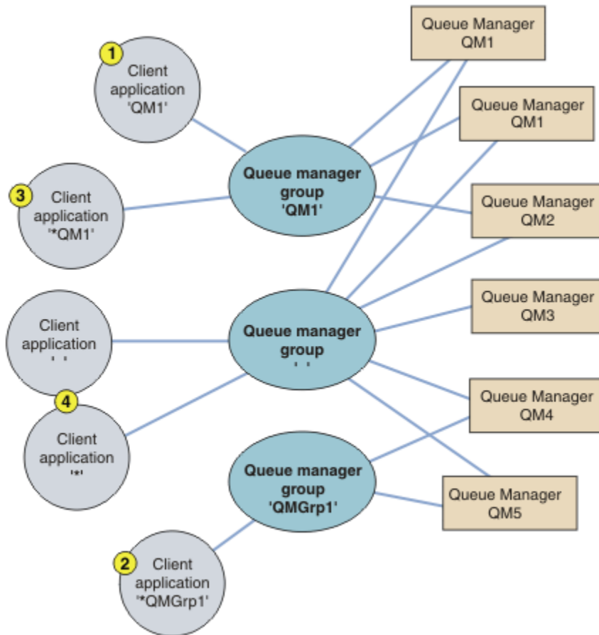
그림 107. 큐 관리자 그룹
