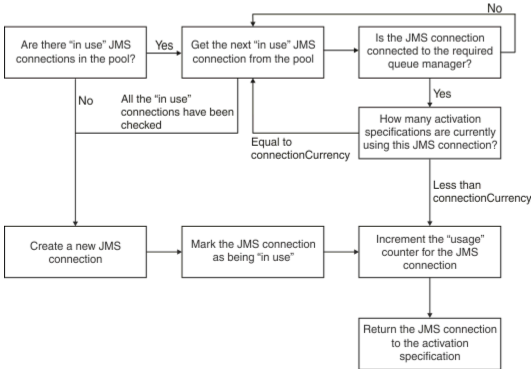
그림 49. WebSphere Application Server 7.5 및 8.0 -연결 풀의 작동 방식
