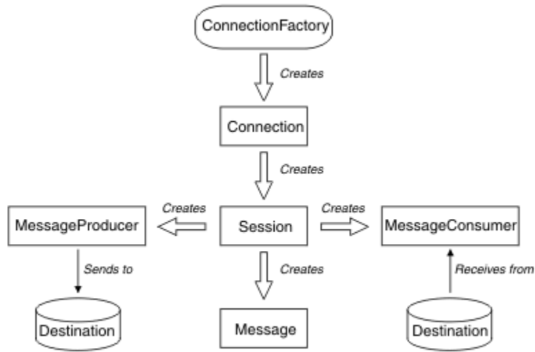
그림 9. JMS 오브젝트 및 해당 관계
