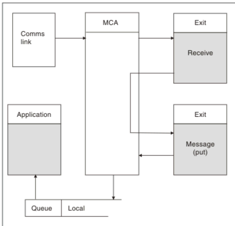
그림 117. 메시지 채널의 수신자 끝에서의 수신 엑시트의 예
