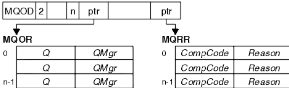
그림 67. C로 분배 목록 열기
