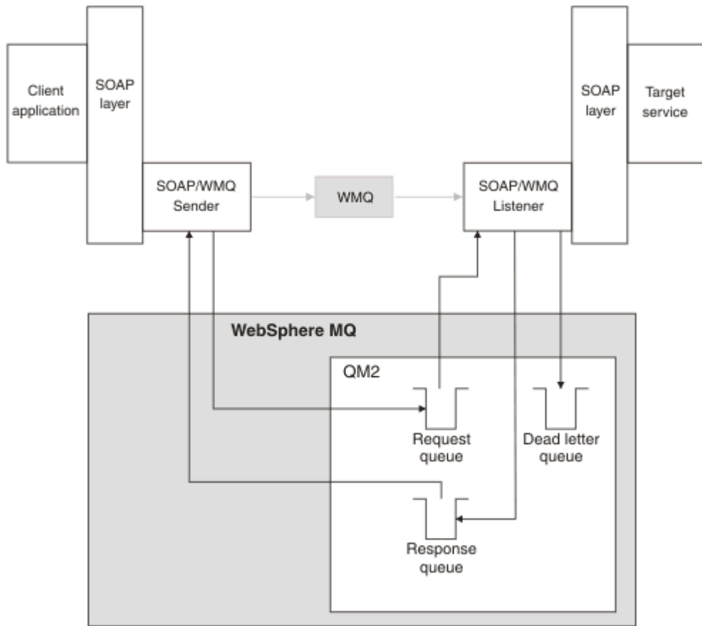
그림 165. SOAP/IBM MQ(단일 큐 관리자)에서 사용하는 큐
