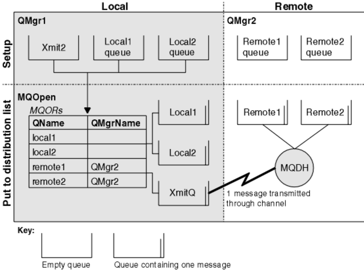
그림 66. 분배 목록의 작동 방법
