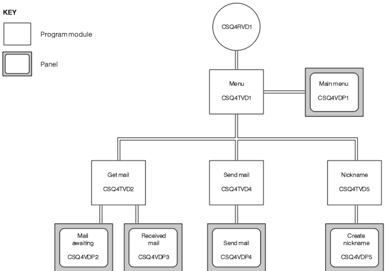
그림 152. 메일 관리자의 TSO 버전에 대한 프로그램 및 패널
