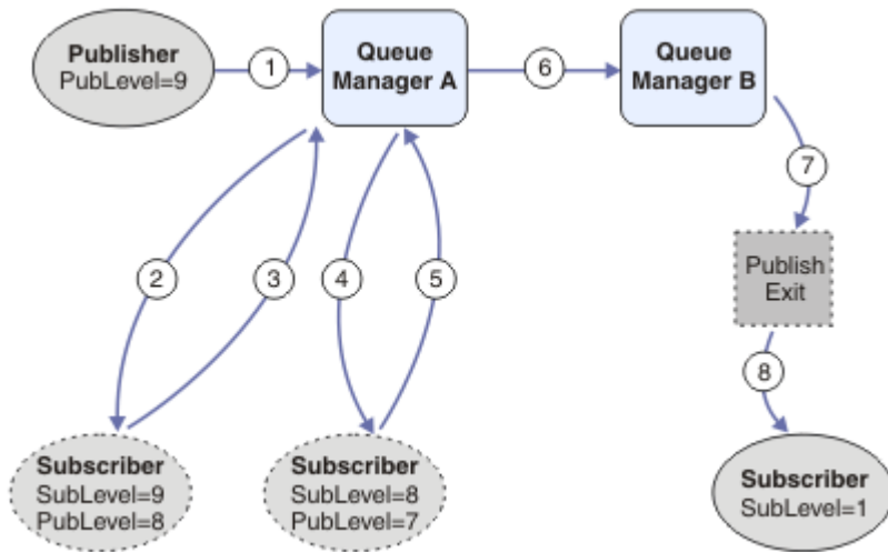
그림 103. 클러스터의 인터셉션 및 발행 엑시트
