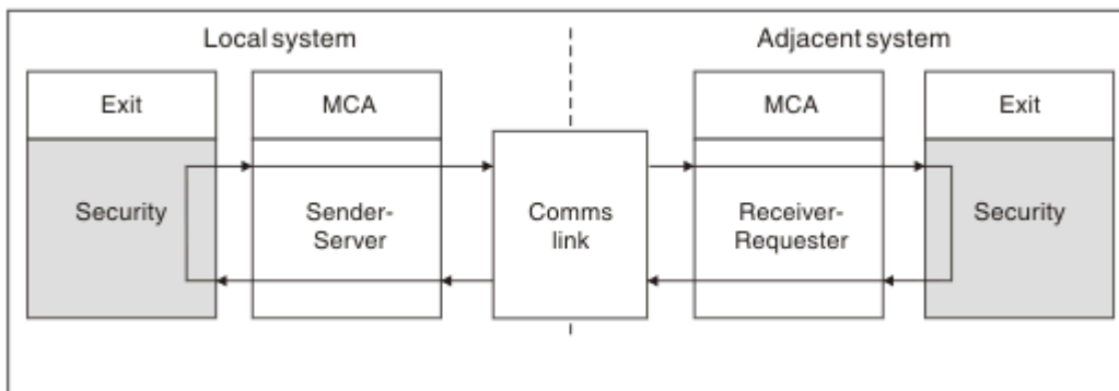
그림 115. 보안 엑시트 루프
