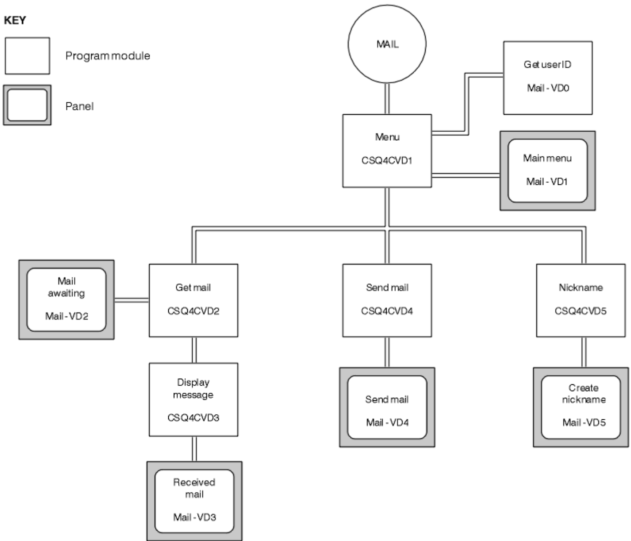
그림 153. 메일 관리자의 CICS 버전에 대한 프로그램 및 패널
