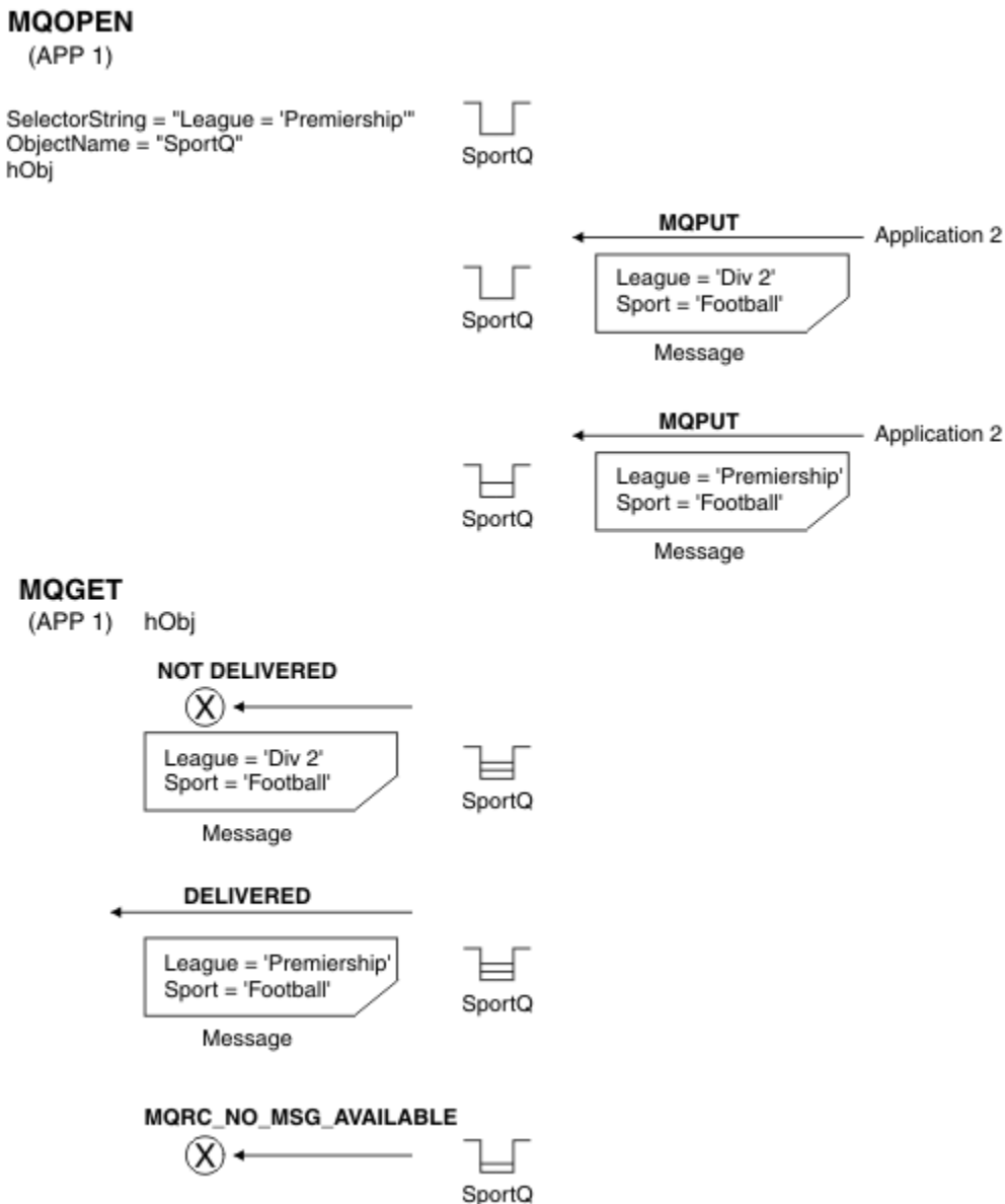
그림 4. MQOPEN 호출을 사용한 선택
