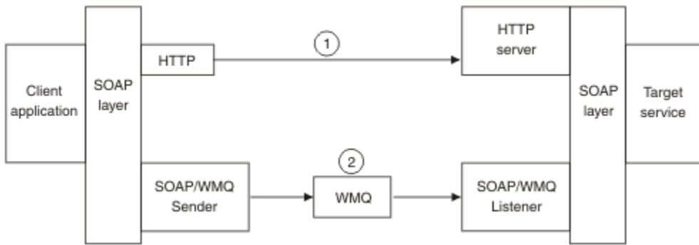
그림 164. SOAP용 IBM MQ 전송 개요
