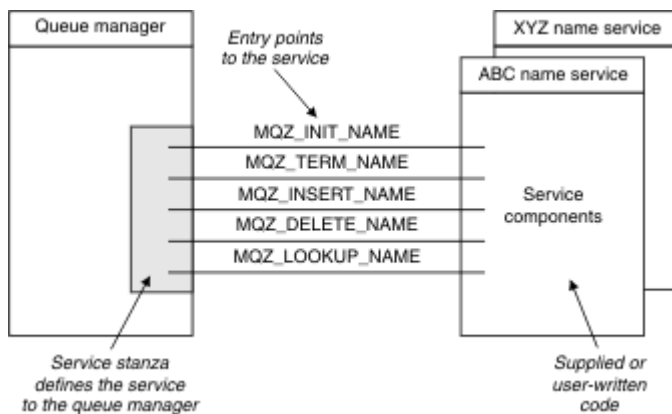
그림 109. 서비스, 컴포넌트 및 시작점 이해
