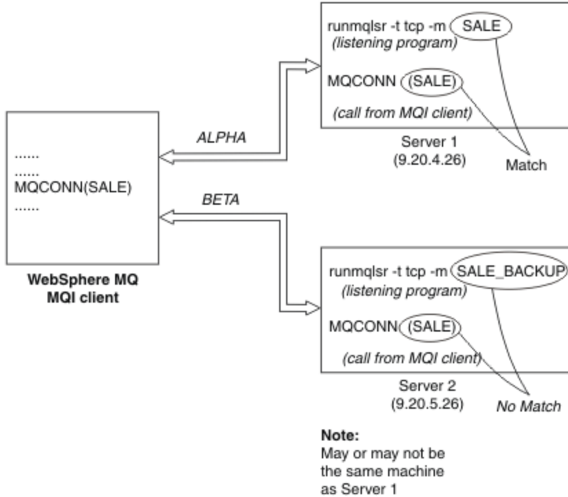
그림 108. MQCONN 예
