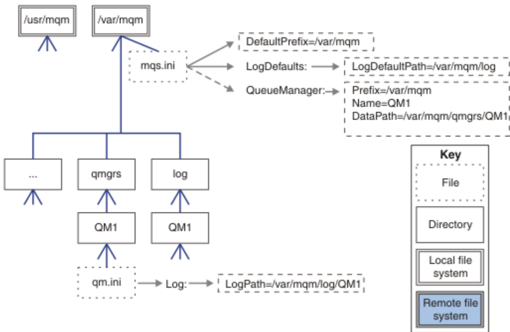
Figure 46. Exemple de structure de répertoire IBM MQ par défaut pour les systèmes UNIX and Linux
