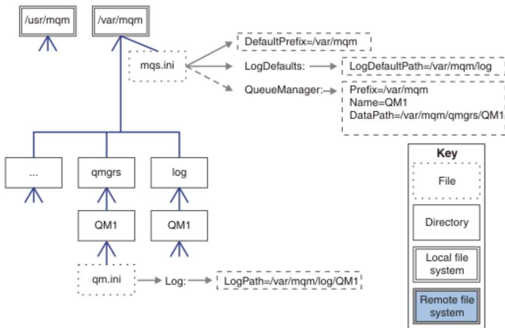
Figure 44. Exemple de structure de répertoire IBM MQ par défaut pour les systèmes UNIX and Linux
