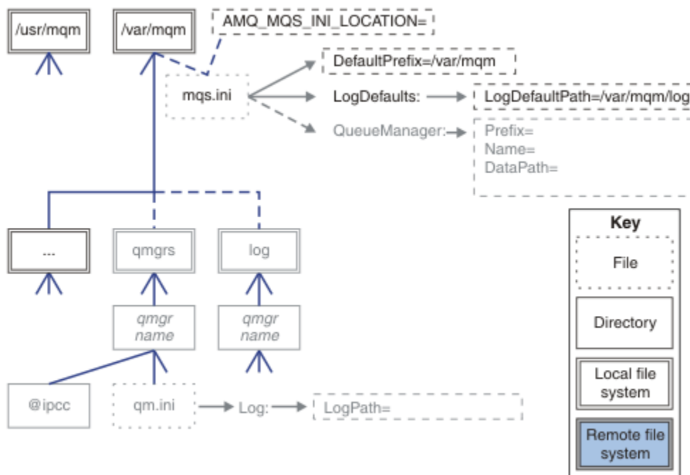
Figure 45. Modèle de canevas de structure de répertoire
