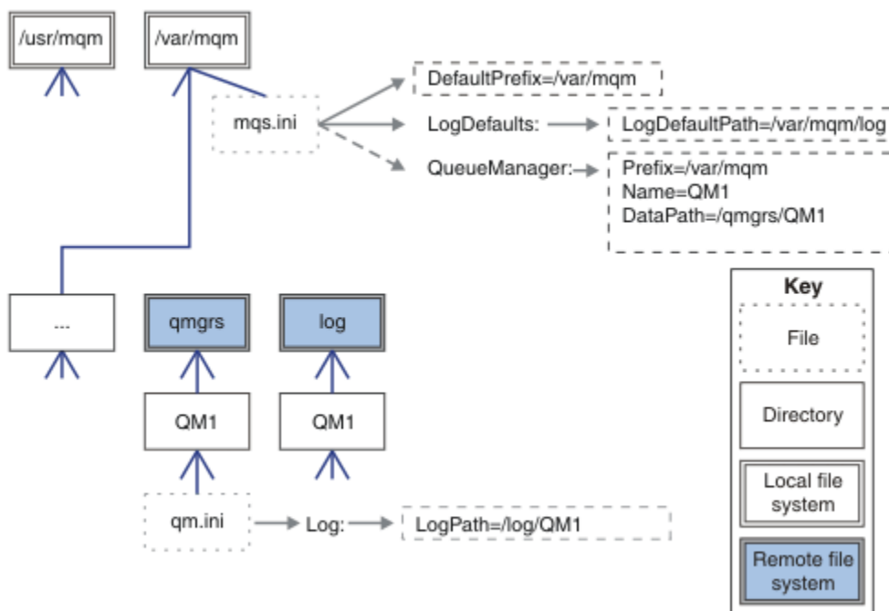
Figure 47. Partage des répertoires qmgrs et Log
