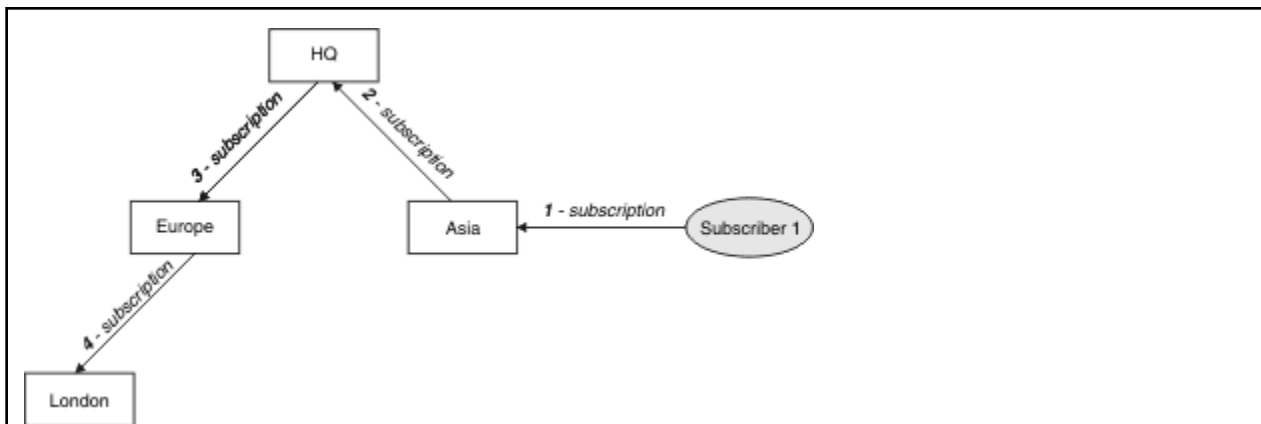
Figure 29. Propagation des abonnements via un réseau de gestionnaires de files d'attente
