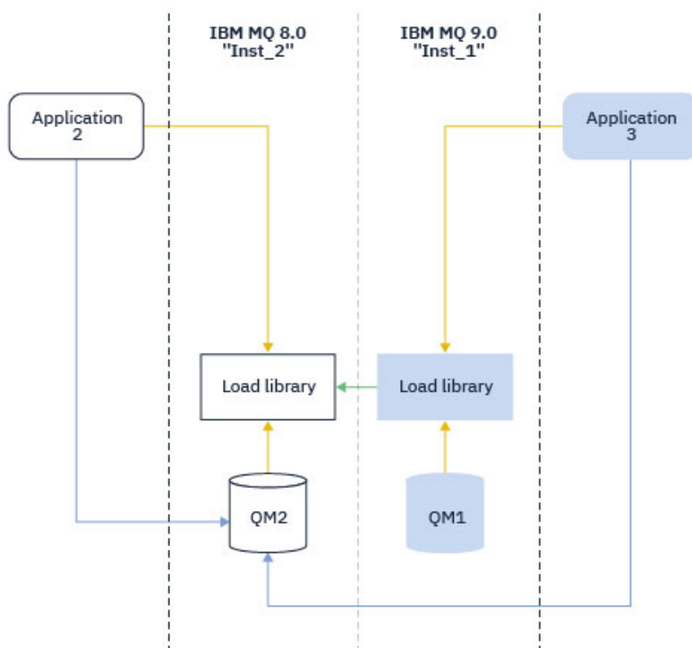
Figure 12. Chargement des appels dans une bibliothèque différente
