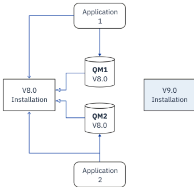
Figure 5. Migration côte à côte : version plus récente installée avec des gestionnaires de files d'attente toujours connectés et des applications toujours associées à la version précédente
