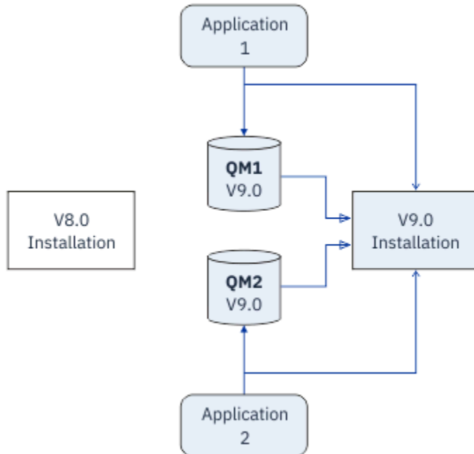
Figure 6. Migration côte à côte : gestionnaires de files d'attente migrés connectés la version plus récente et applications associées à la version plus récente
