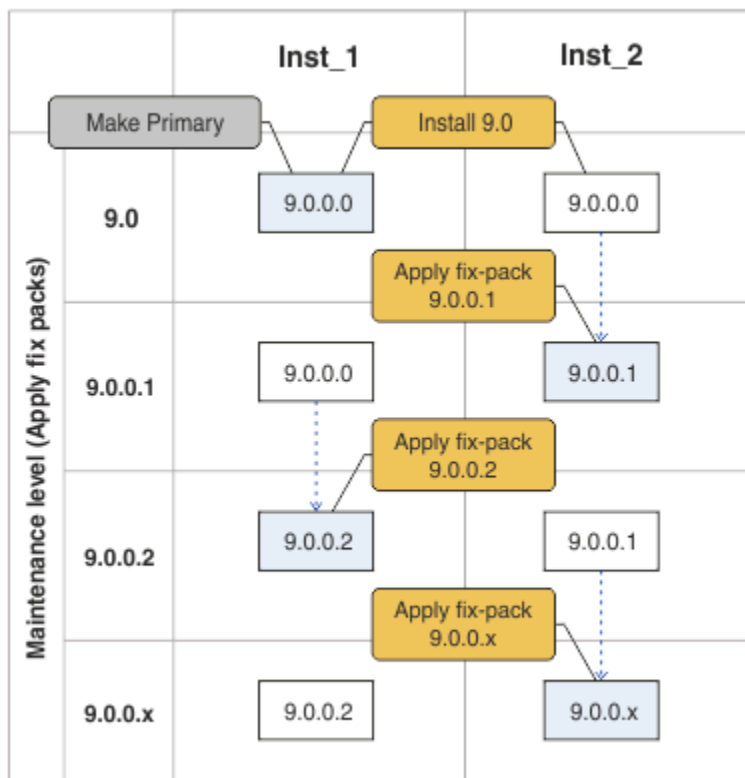
Figure 10. Déploiement de correctifs
