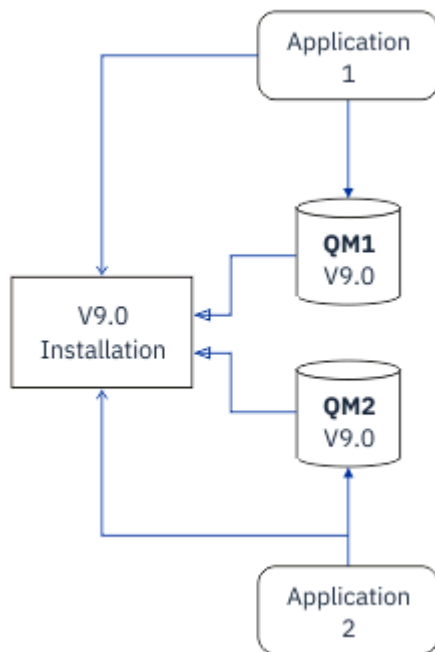
Figure 4. Migration à une seule étape : gestionnaires de files d'attente migrés connectés et applications associées à la version plus récente
