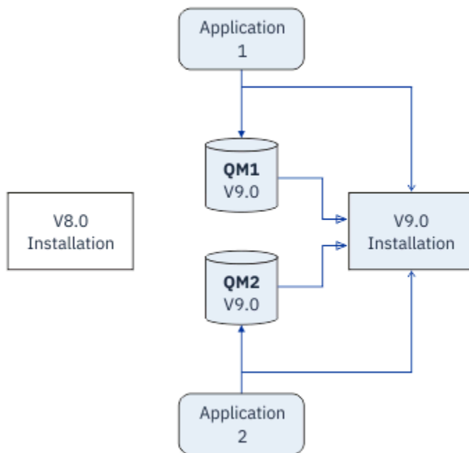
Figure 9. Installation côte à côte - étape 4
