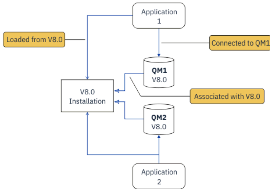
Figure 2. Migration à une seule étape : version précédente installée avec des gestionnaires de files d'attente connectés et des applications associées
