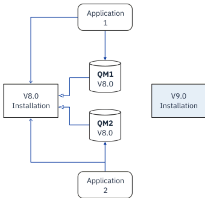
Figure 8. Installation côte à côte - étape 2
