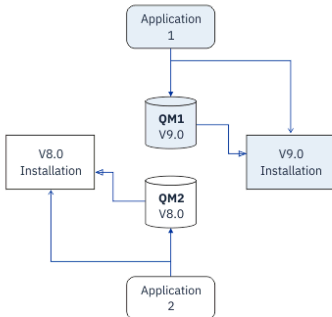
Figure 7. Migration à plusieurs étapes : un gestionnaire de files d'attente et une application migrés vers la version plus récente, et un autre gestionnaire de files d'attente et une autre application toujours à la version précédente
