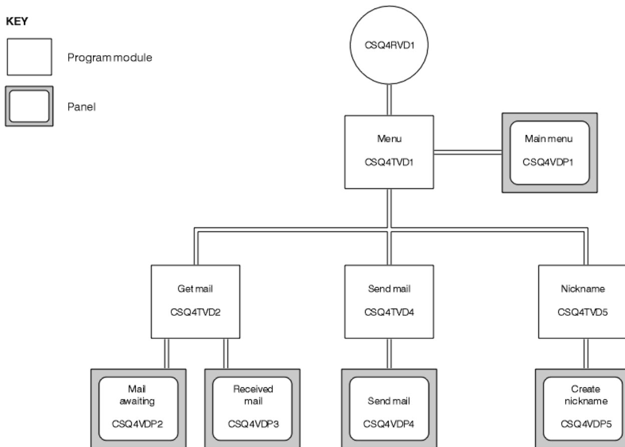
Figure 152. Programmes et panneaux pour les versions TSO du gestionnaire de messagerie
