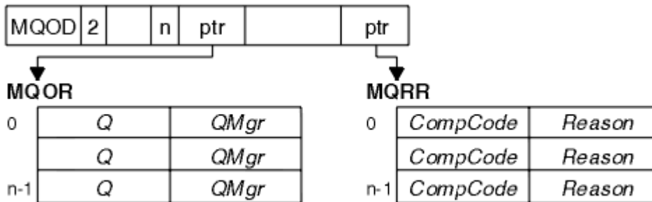
Figure 67. Ouverture d'une liste de distribution en C
