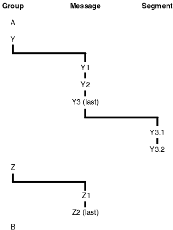
Figure 71. Ordre logique dans une file d'attente
