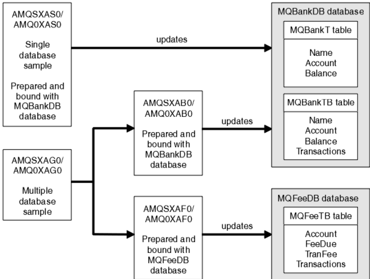
Figure 140. Exemples de coordination de base de données
