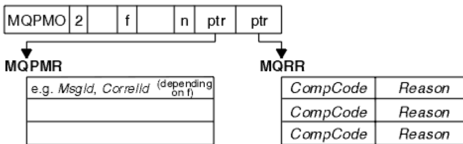
Figure 69. Insertion d'un message dans une liste de distribution en C
