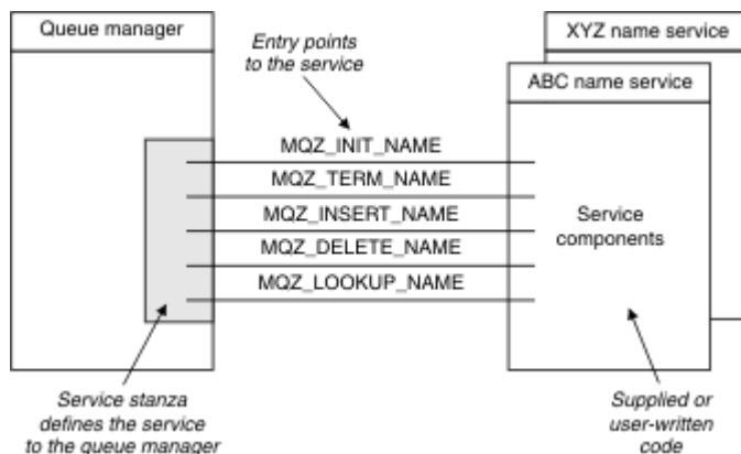
Figure 109. Description des services, des composants et des points d'entrée
