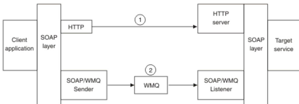
Figure 164. Présentation du transport IBM MQ pour SOAP
