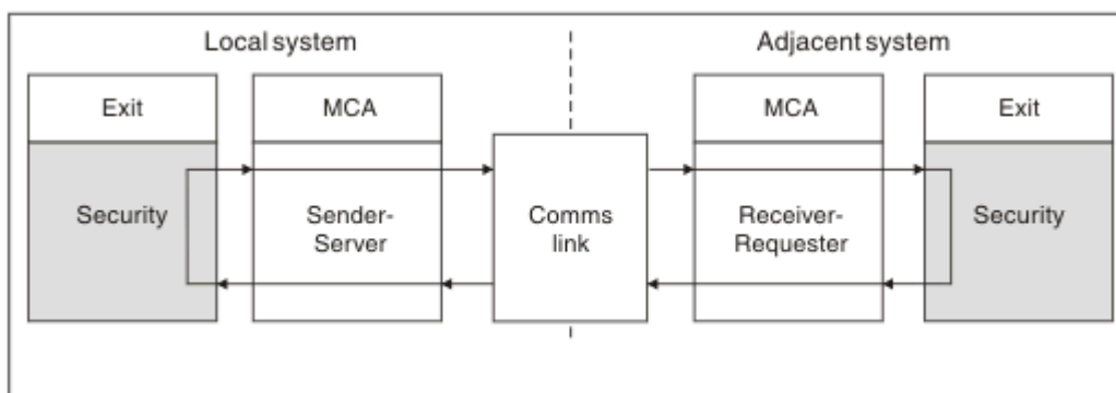
Figure 115. Boucle d'exit de sécurité
