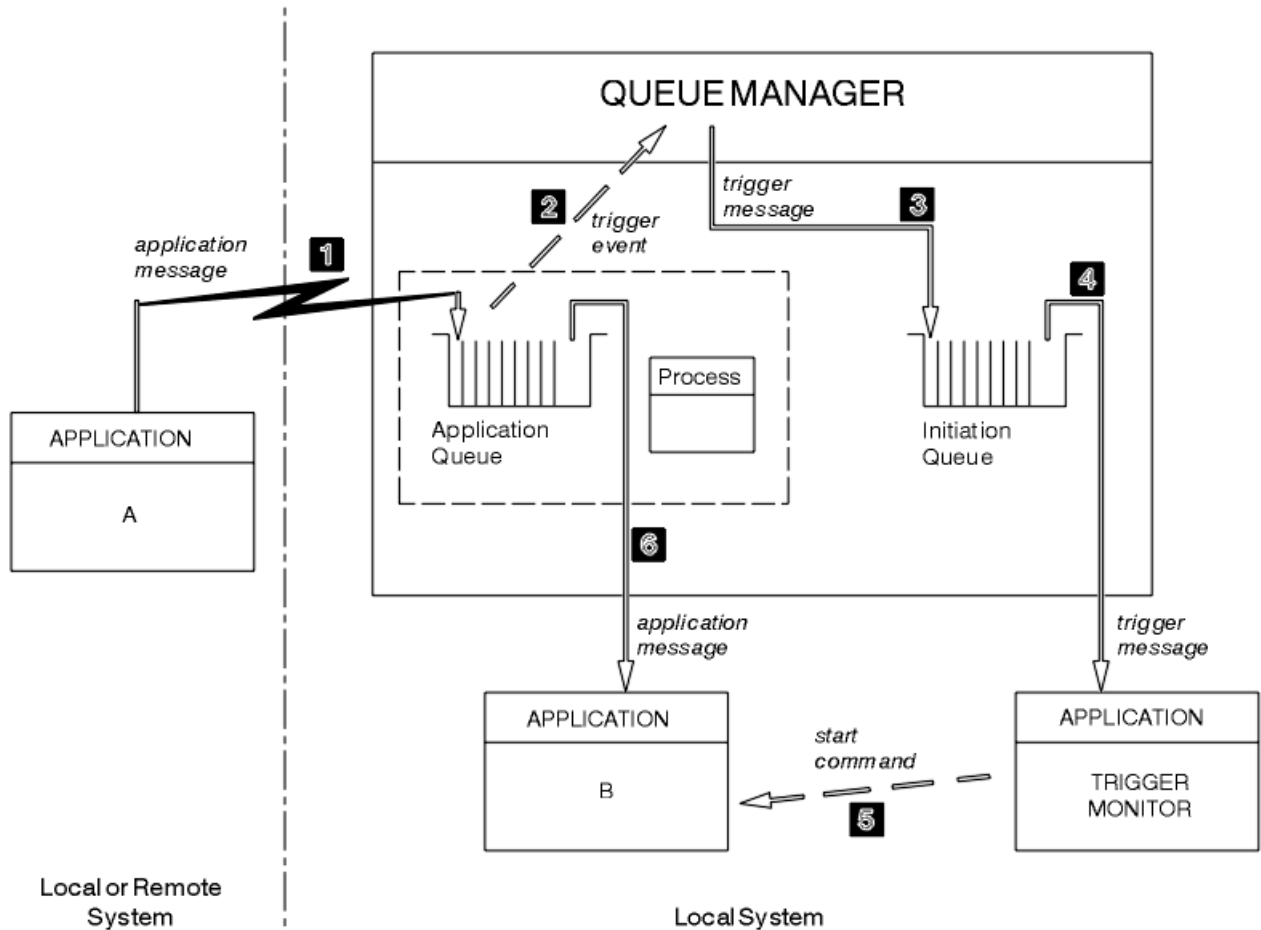
Figure 105. Flux de messages d'application et de déclenchement
