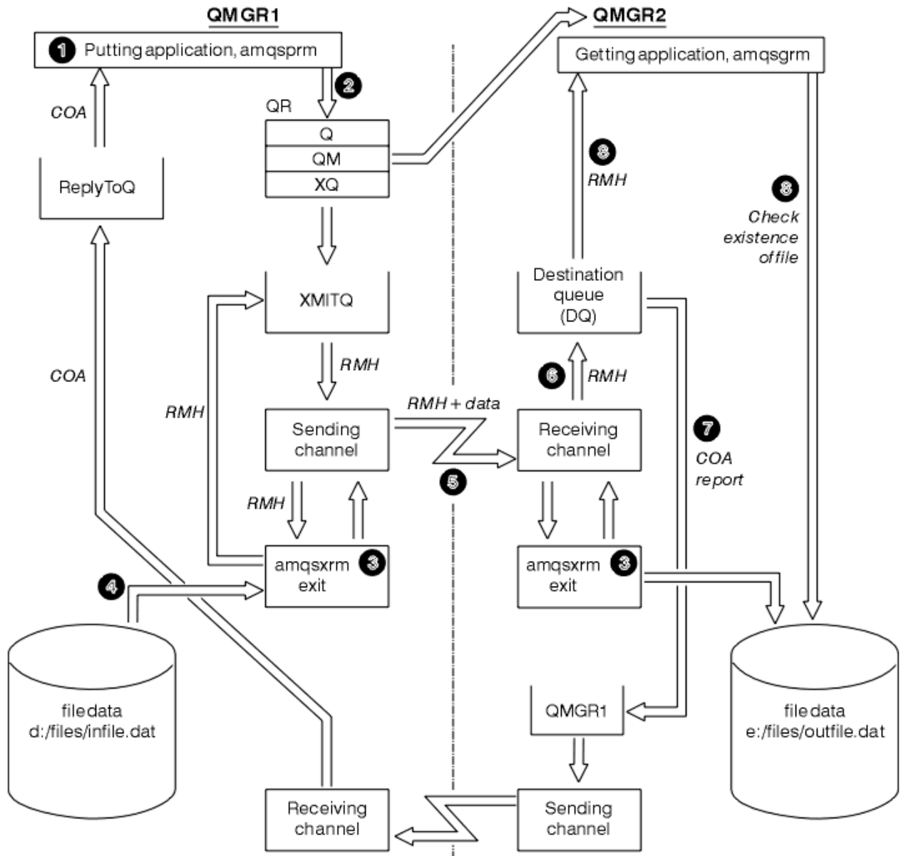
Figure 143. Exécution des exemples de message de référence
