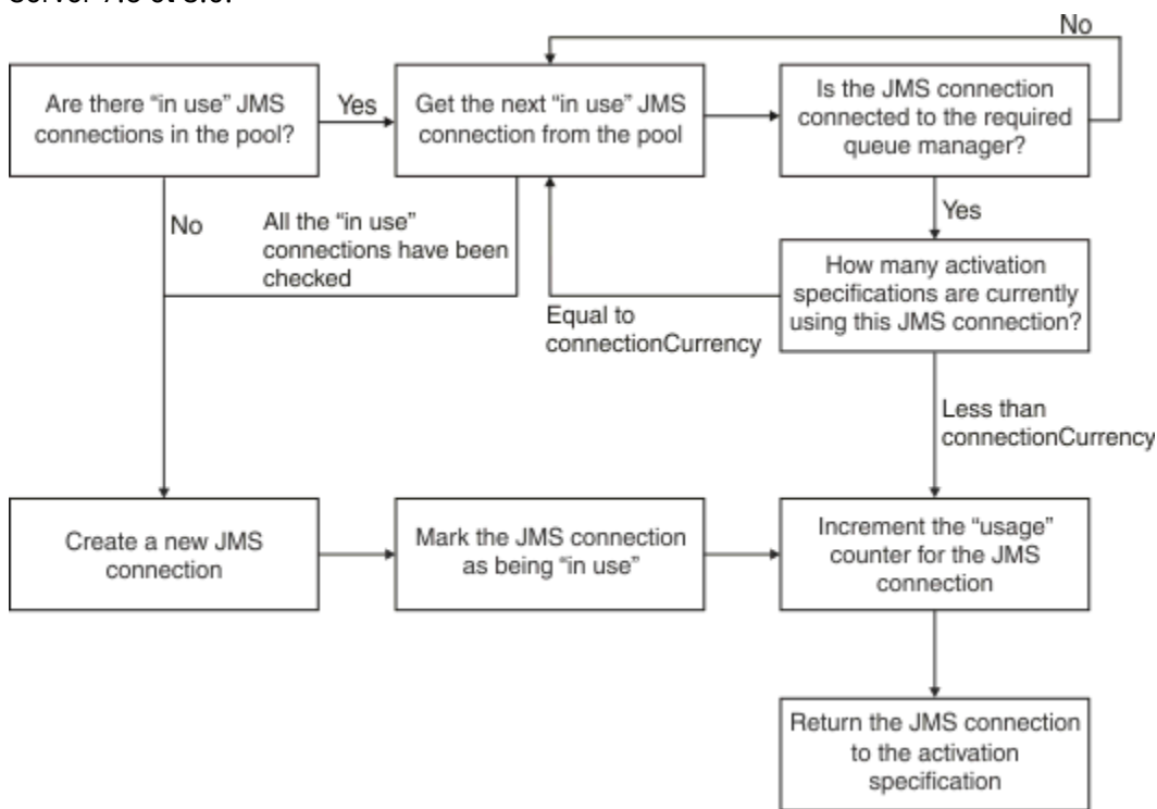
Figure 49. WebSphere Application Server 7.5 et 8.0 -mode de fonctionnement du pool de connexions
