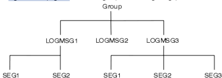
Figure 8. Messages segmentés
