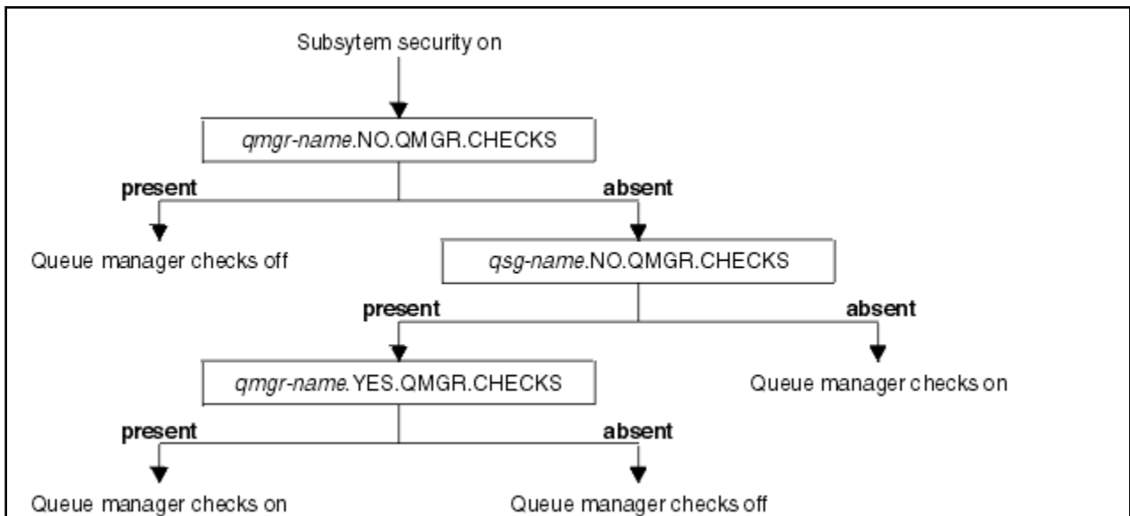
Figura 15. Comprobación de la seguridad a nivel de gestor de colas
