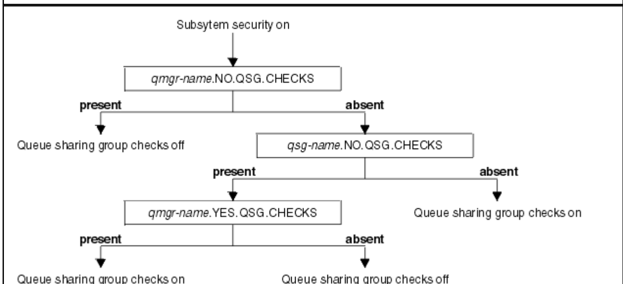
Figura 16. Comprobación de la seguridad a nivel de grupo de compartición de colas
