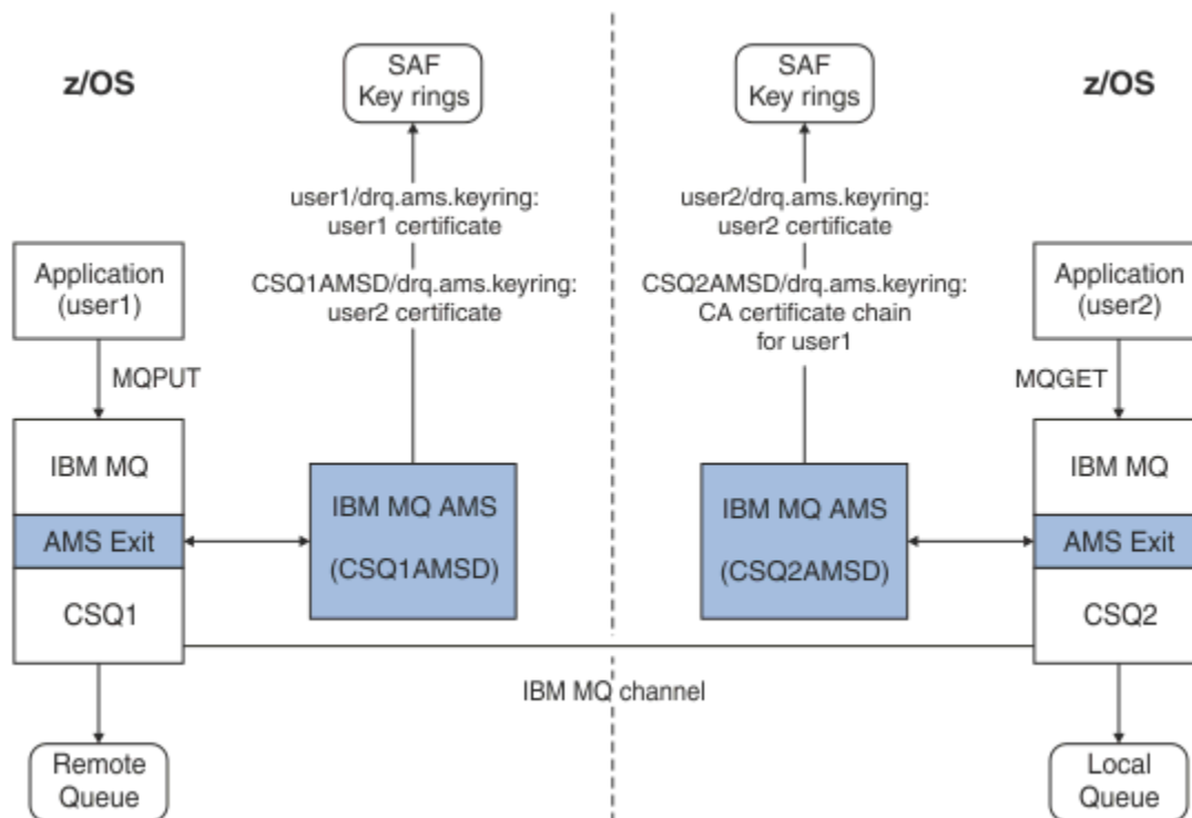
Figura 32. Relaciones entre las aplicaciones y los certificados
