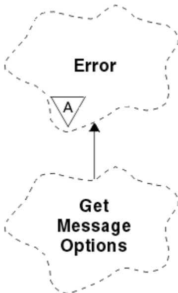
Figura 54. Clase ImqGetMessageOptions
