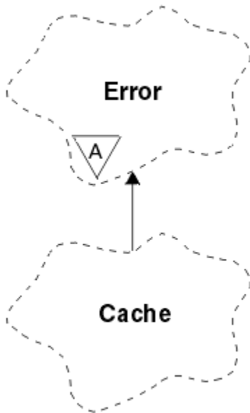
Figura 48. Clase ImqCache
