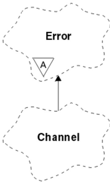
Figura 49. Clase ImqChannel
