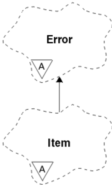
Figura 57. Clase ImqItem
