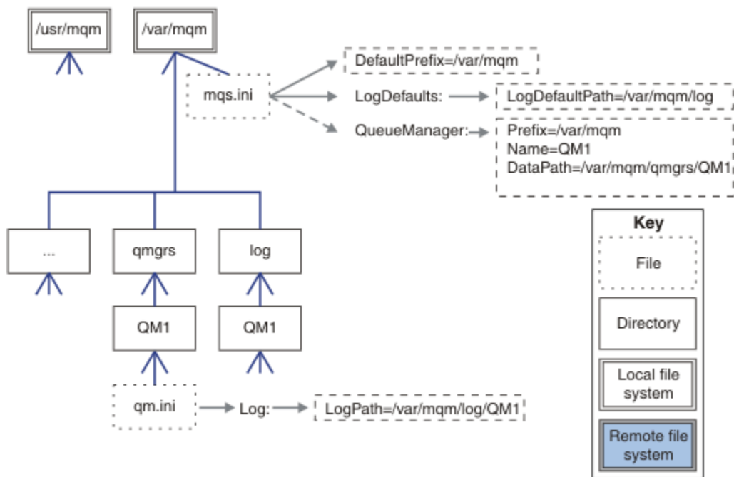
Abbildung 44. Beispiel für eine standardmäßige IBM MQ-Datei- und Verzeichnisstruktur für Systeme mit UNIX and Linux
