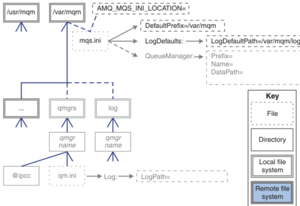
Abbildung 45. Vorlage für Verzeichnisstrukturmuster
