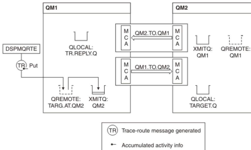
Abbildung 13. Anforderung einer Trace-Route-Antwortnachricht, Diagramm 1
