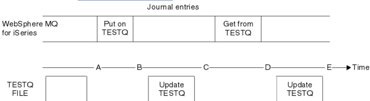
Obrázek 34. Posloupnost událostí při aktualizaci objektů MQM
