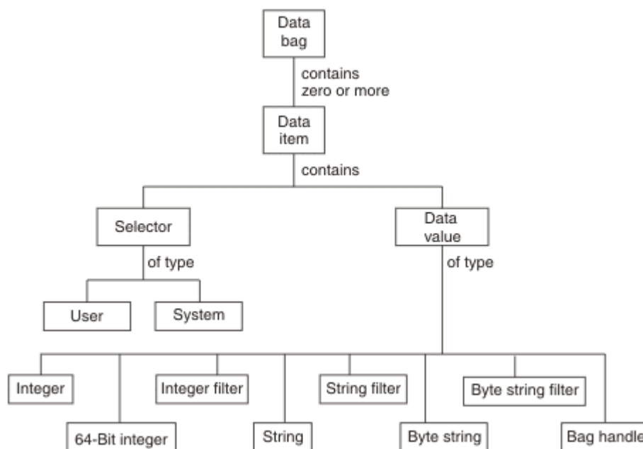
Obrázek 5. Hierarchie konceptů MQAI
