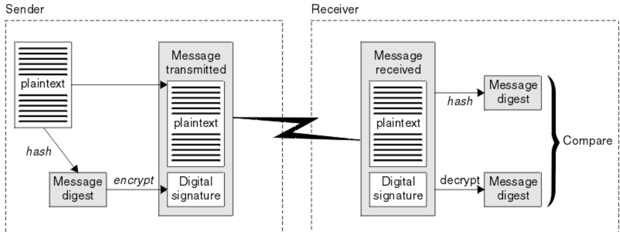
圖 6: 數位簽章處理程序
