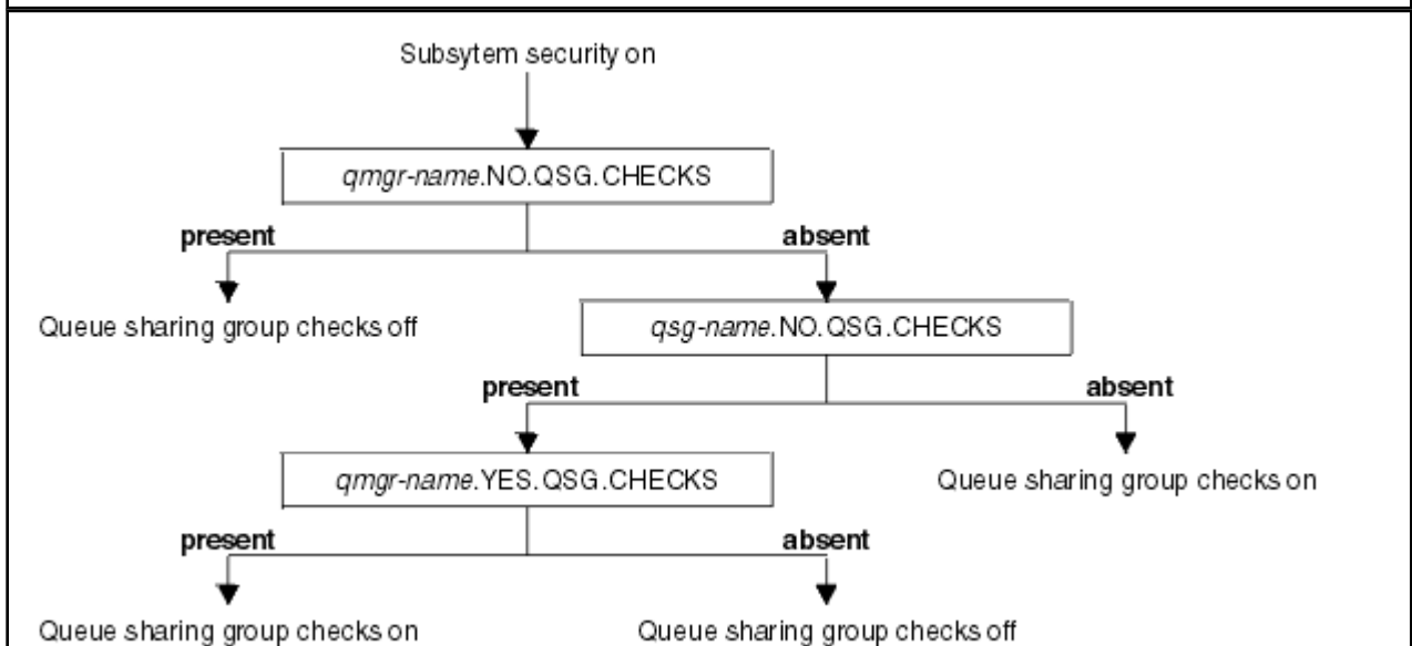
圖 16: 檢查佇列共用群組層次安全
